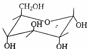
Dạng 1C
