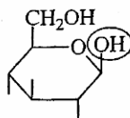
Công thức vòng Haworth
