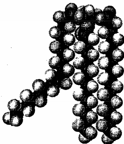
Hình 20.2. Mô hình phân tử của triglycerid no (a) và chưa no (b)
