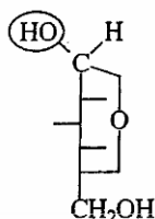
Công thức hình chiếu Fischer
