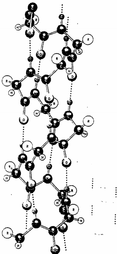
Hình 22.1. Cấu trúc của \alpha -keratin
