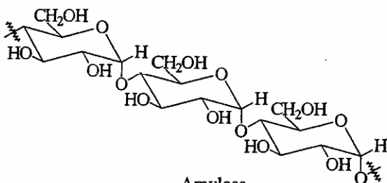
Amylose Polymer của [1-4'-O-( \alpha -D-glucopyranosid)]
