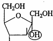
\alpha -D-fructofuranose
