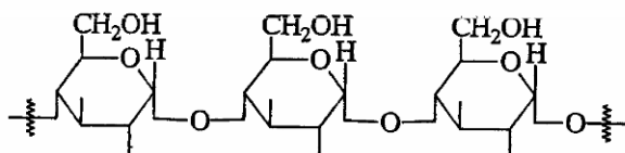
Amylose Polymer của [1-4'-O-( \alpha -D-glucopyranosid)]
