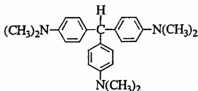
Base không màu của (leucobase) tím gentian
