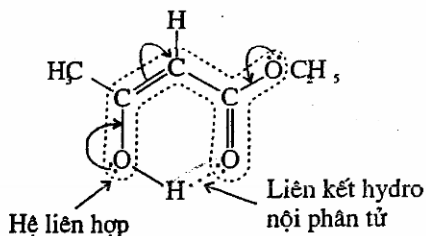
Dạng enol của ester aceto acetic
