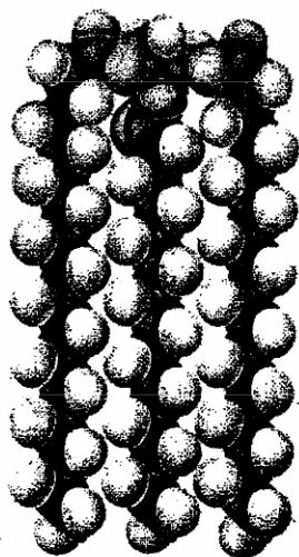
Hình 20.2. Mô hình phân tử của triglycerid no (a) và chưa no (b)
