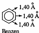
Benzen
