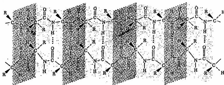
Hình 22.2. Cấu trúc bậc 2 gấp nếp \beta trong sợi fibroin.
