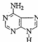
Adenin (6-aminopurin)
