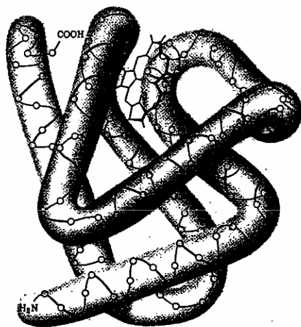
Hình 22.3. Cấu trúc của mioglobin.
