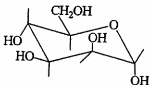
\alpha -D-manopyranose
