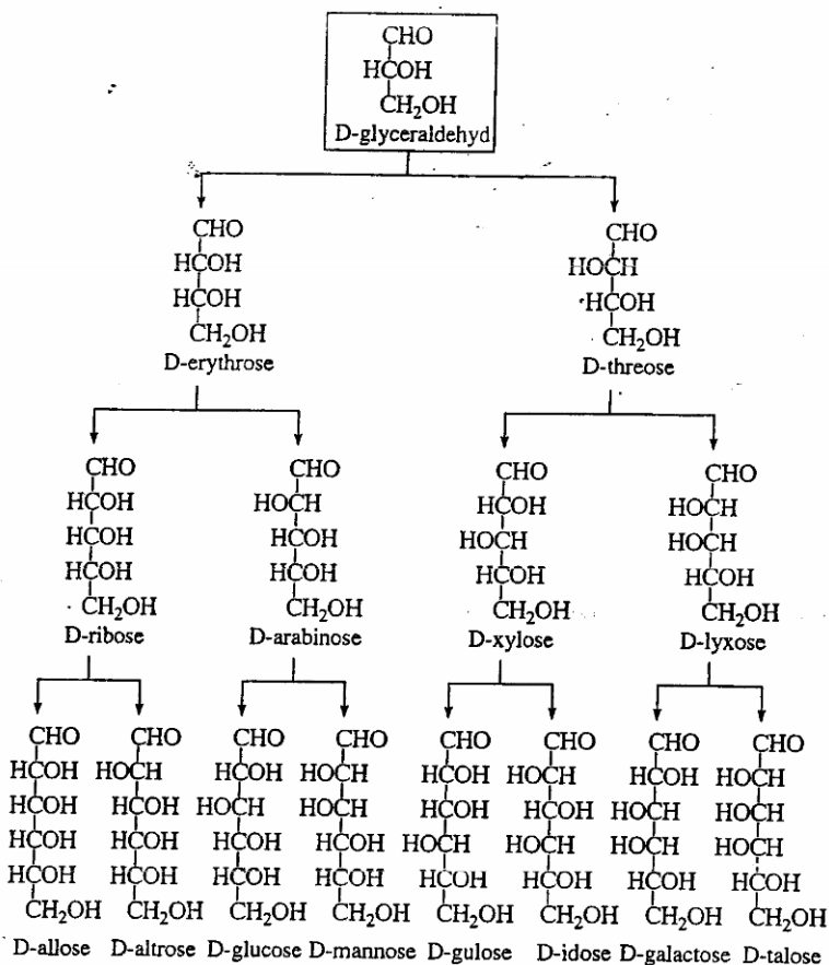
Hình 21.1. Một số đường dây D xuất phát từ D-glyceraldehyd
