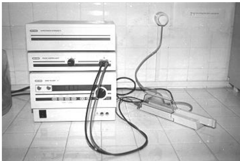
Hình 2.16: Máy xung gen (Gene pulser) (Hãng Biorad)
