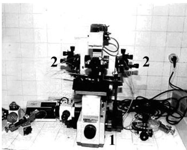
Hình 2.9: Máy vi thao tác Olympus (Hãng Narishige)
