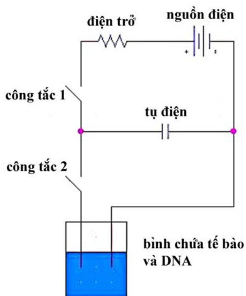
Hình 2.17: Sơ đồ bố trí mạch cơ bản của máy xung điện
