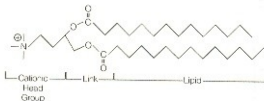
Hình 2.3: Cấu trúc tổng quát của lipid cation tổng hợp
