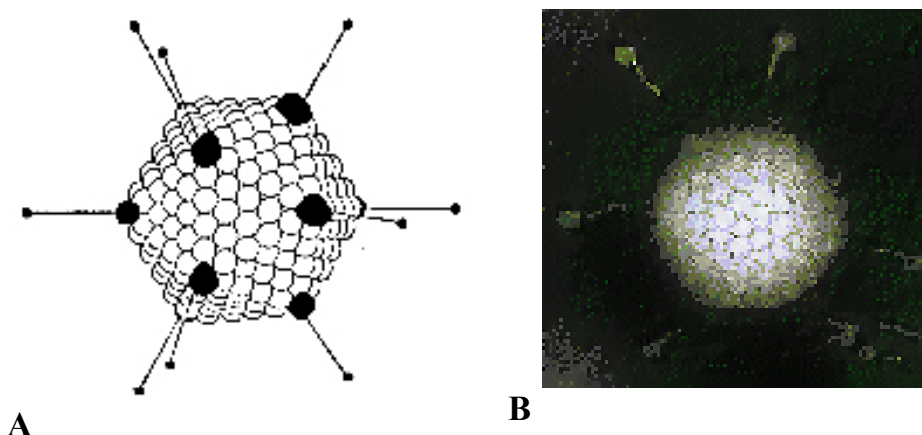
Hình 1.10: Adenovirus
