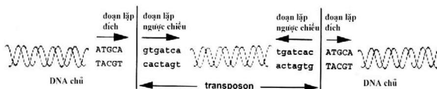
Hình 1.2: Cấu trúc của transposon
