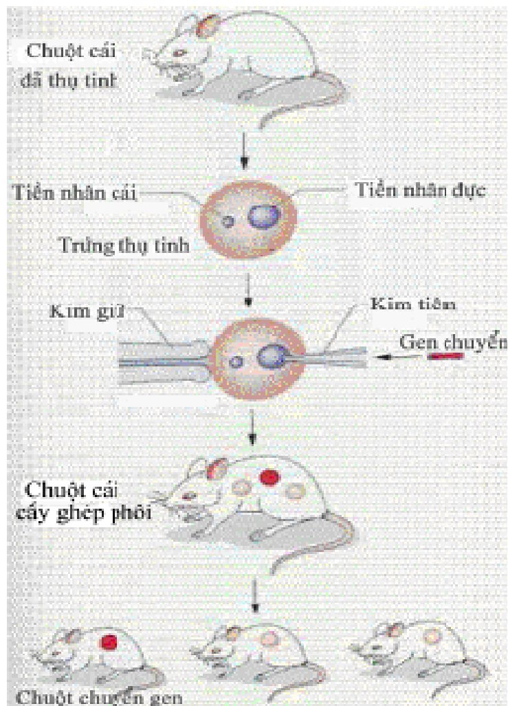
Hình 2.10: Chuyển gen bằng vi tiêm
