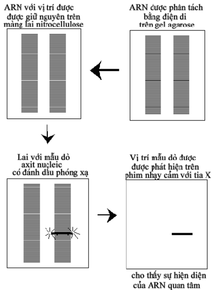
Hình 3.2: Sơ đồ mô tả phương pháp Northern blot
