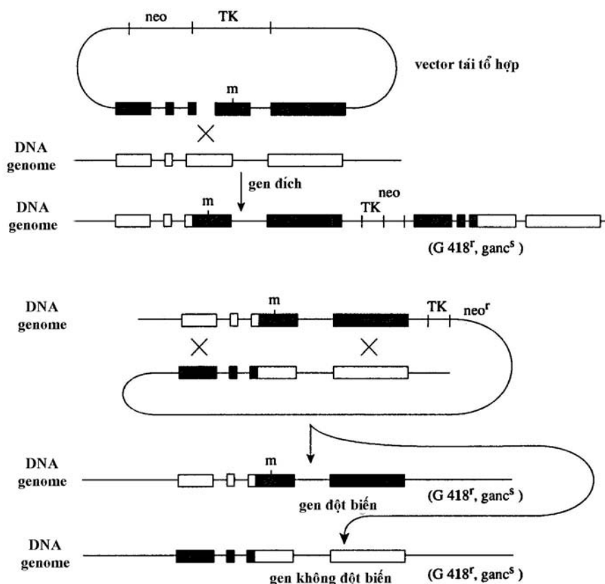
Hình 1.17: Sự thay thế gen bằng thể đột biến sử dụng tái tổ hợp tương đồng kép
