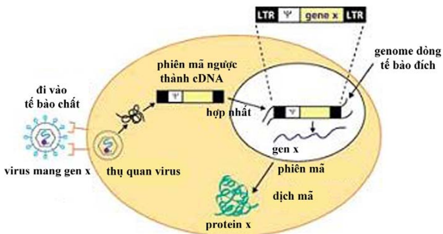
Hình 1.8: Cơ chế hoạt động của vector retrovirus
