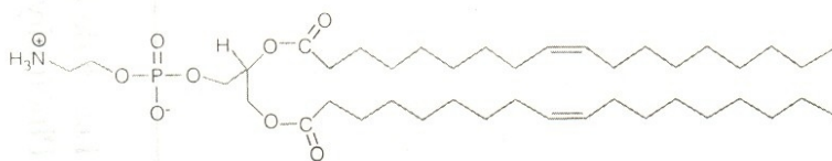
Hình 2.4: Cấu trúc của DOPE (L-dioleoyl phosphatidylethanolamine)
