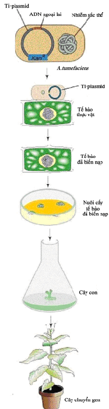
Hình 2.23: Tạo thực vật chuyển gen bằng phương pháp chuyển gen gián tiếp nhờ Agrobacterium
