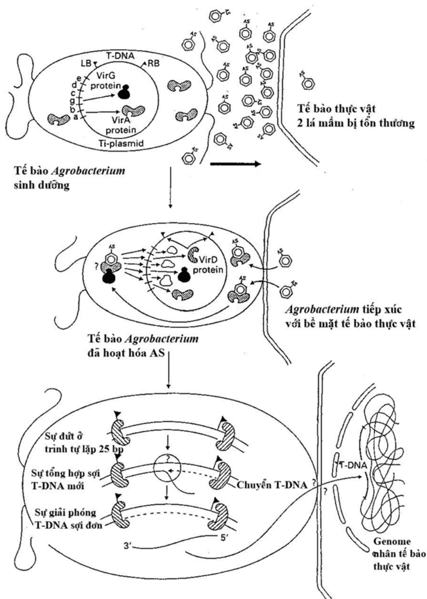
Hình 1.12: Sự tương tác giữa Agrobacterium với tế bào thực vật và cơ chế chuyển T-DNA
