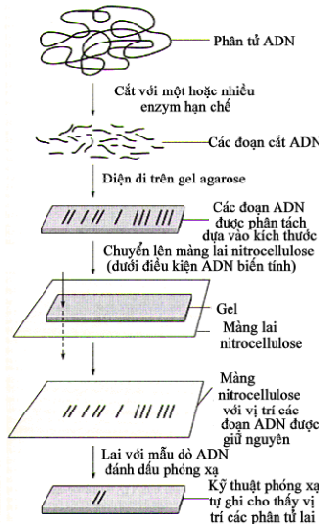
Hình 3.1: Sơ đồ tái phôi ảnh phản Southern blot
