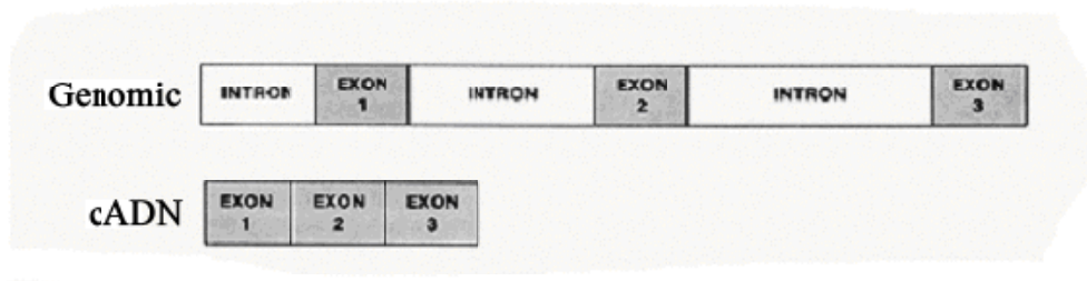
Hình 4.2: So sánh hai dạng gen chuyển
