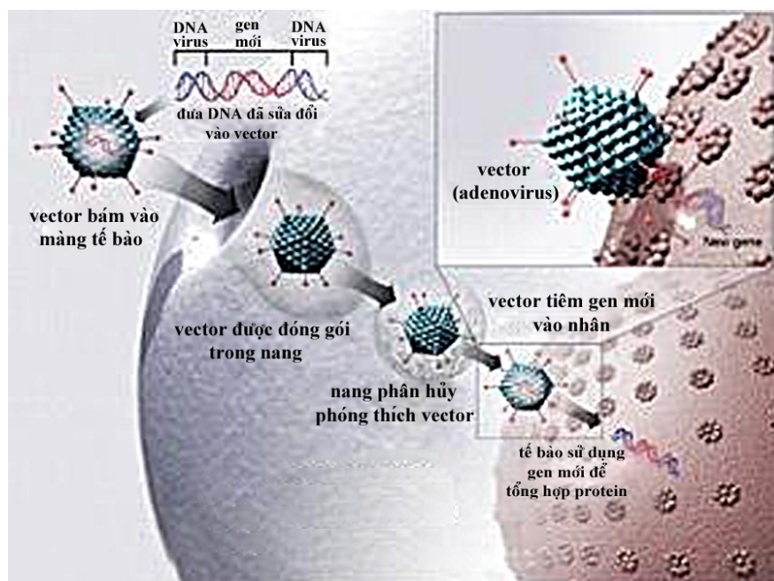
Hình 1.12: Cơ chế hoạt động của vector adenovirus
