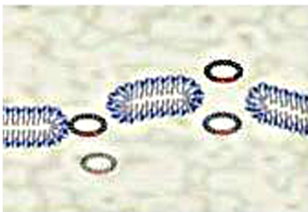
Hình 2.18: Sơ đồ plasmid chứa DNA ngoại lai đi qua các lỗ tạm thời trên màng bào chất
