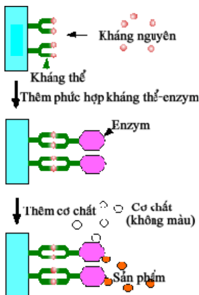
Hình 3.5: Nguyên tắc của phương pháp ELISA
