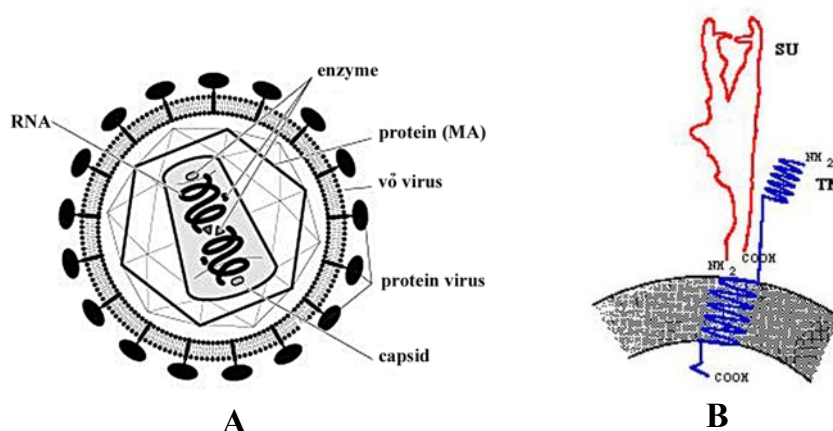
Hình 1.4: Sơ đồ cấu trúc cắt ngang của retrovirus
