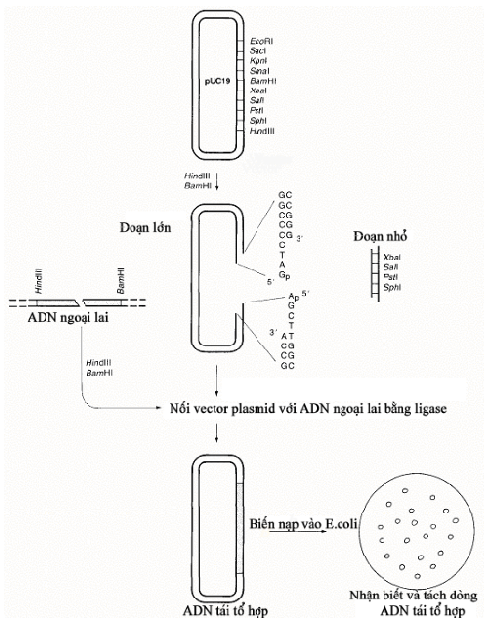
Hình 1.1: : Tạo dòng bằng vector plasmid
