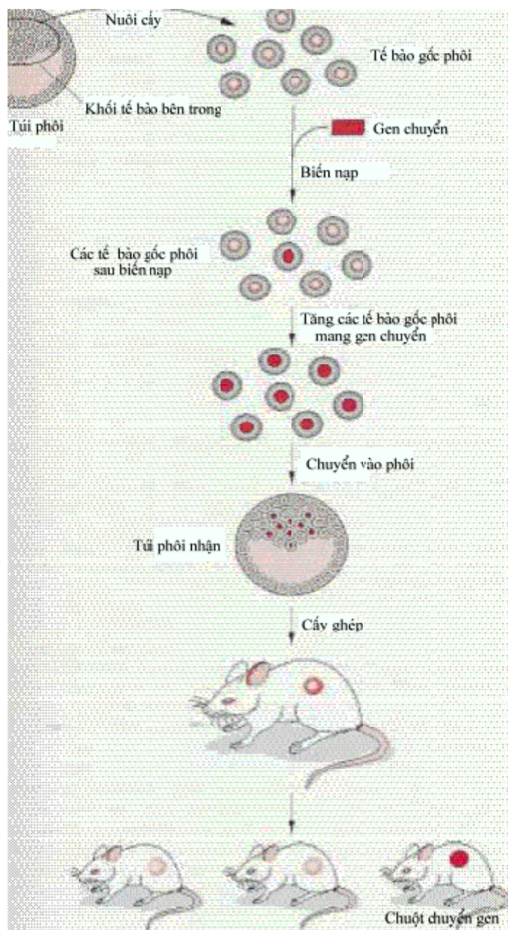
Hình 2.12: Phương pháp chuyển gen bằng cách sử dụng tế bào gốc phôi
