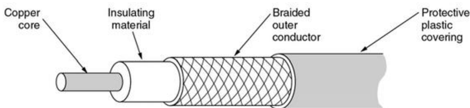
H3.10 Cáp đồng trục
