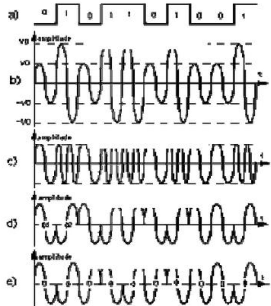
H3.26 Mã hóa đường truyền bằng tín hiệu tuần tự
