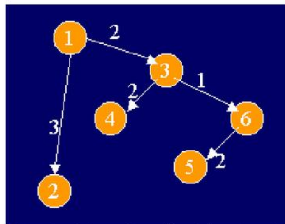
H6.7 Cây đường đi ngắn nhất từ nút 1
