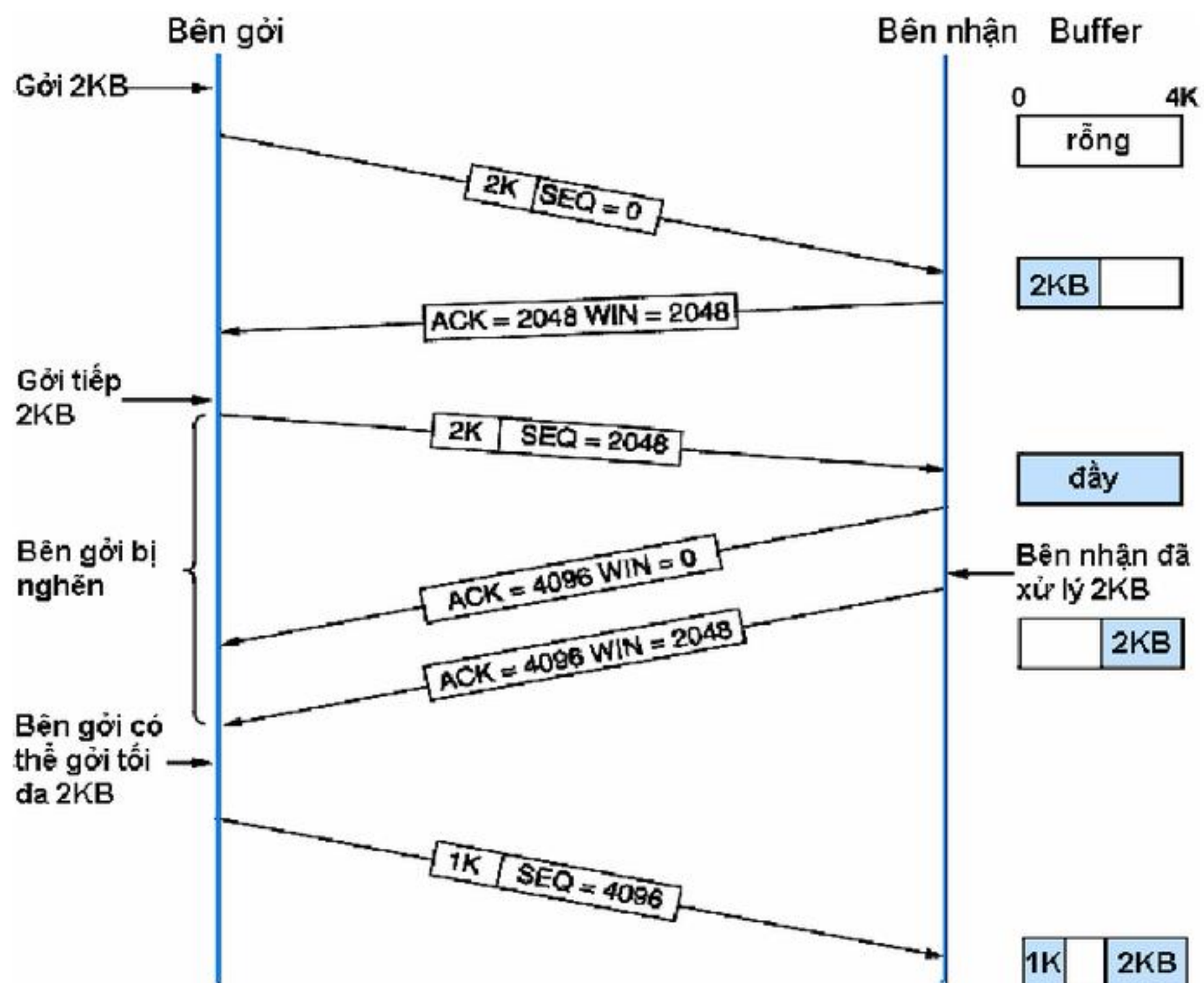
H7.16 Ví dụ về điều khiển thông lượng trong TCP
