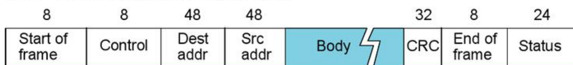
H5.35 Khung thông tin FDDI
