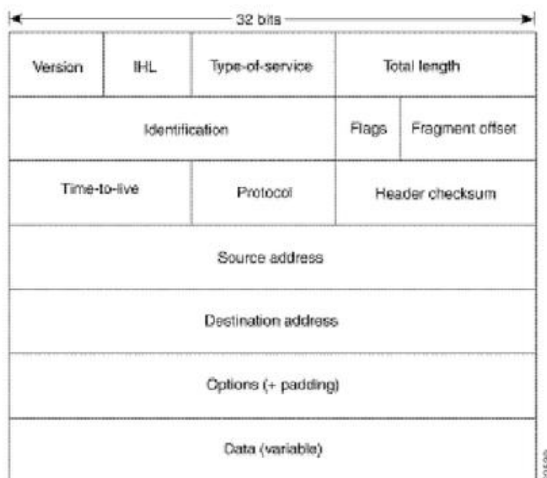
H6.30 Cấu trúc gói tin IP
