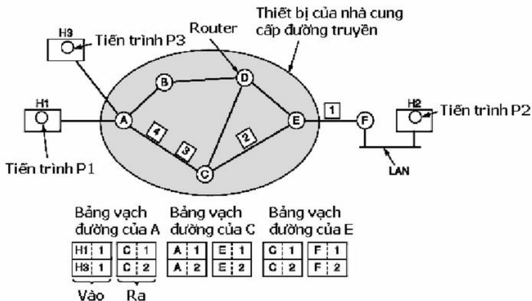
H6.3 Hoạt động của Datagram subnet
