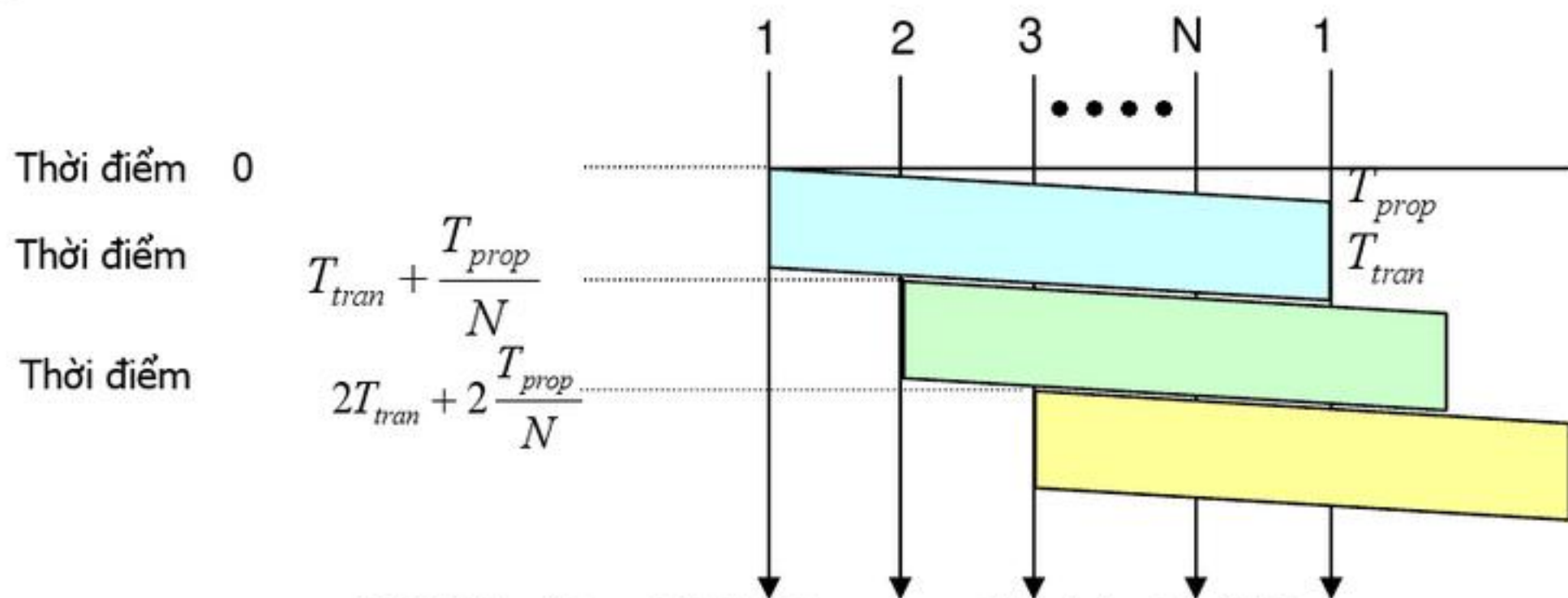
H5.23 Khi một trạm phải nhả token ngay sau khi nó vừa phát dữ liệu
