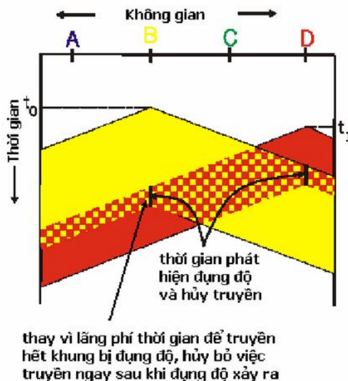
H5.13 Xử lý khu đụng độ
