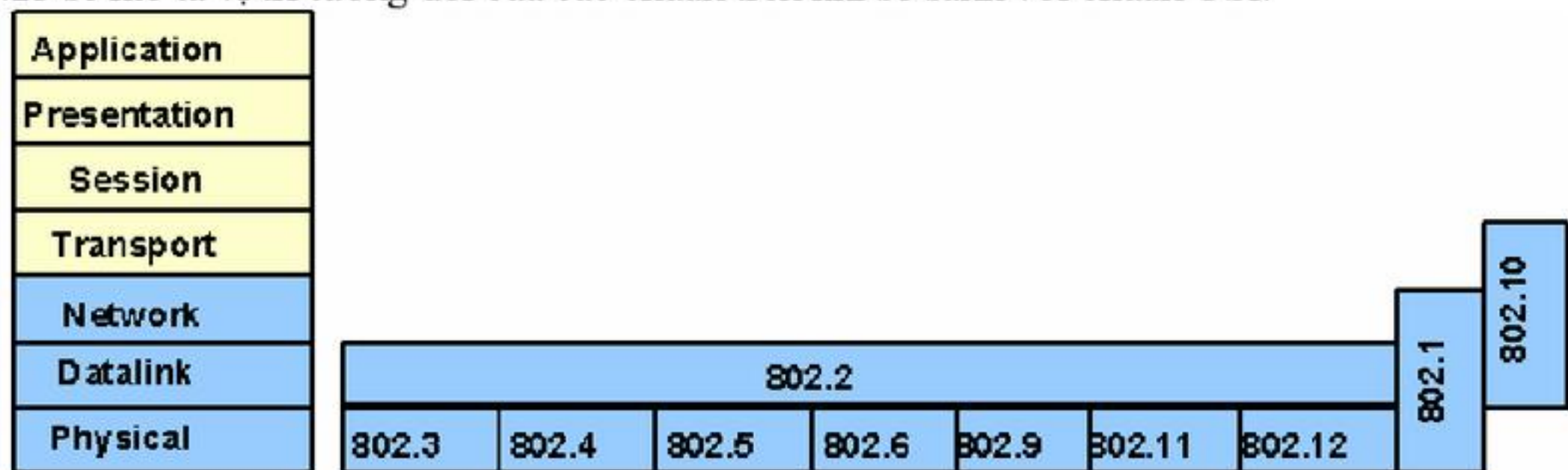
H5.26 Quan hệ giữa các chuẩn IEEE và mô hình OSI
