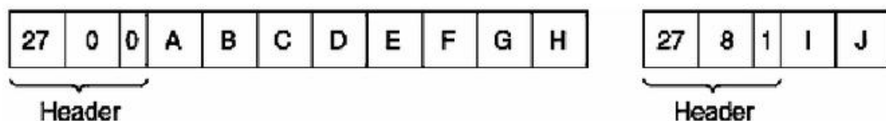
H6.28(b) Gói bị chia thành hai mảnh 8 bytes và 2 bytes
