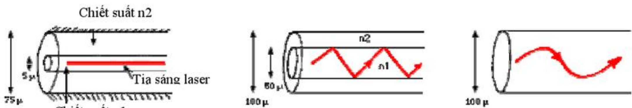
H3.14 Cáp quang chế độ đơn - chế độ đa không thấm thấu - chế độ đa thấm thấu
