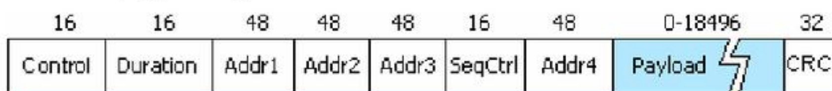
H5.40 Khuôn dạng khung 802.11
