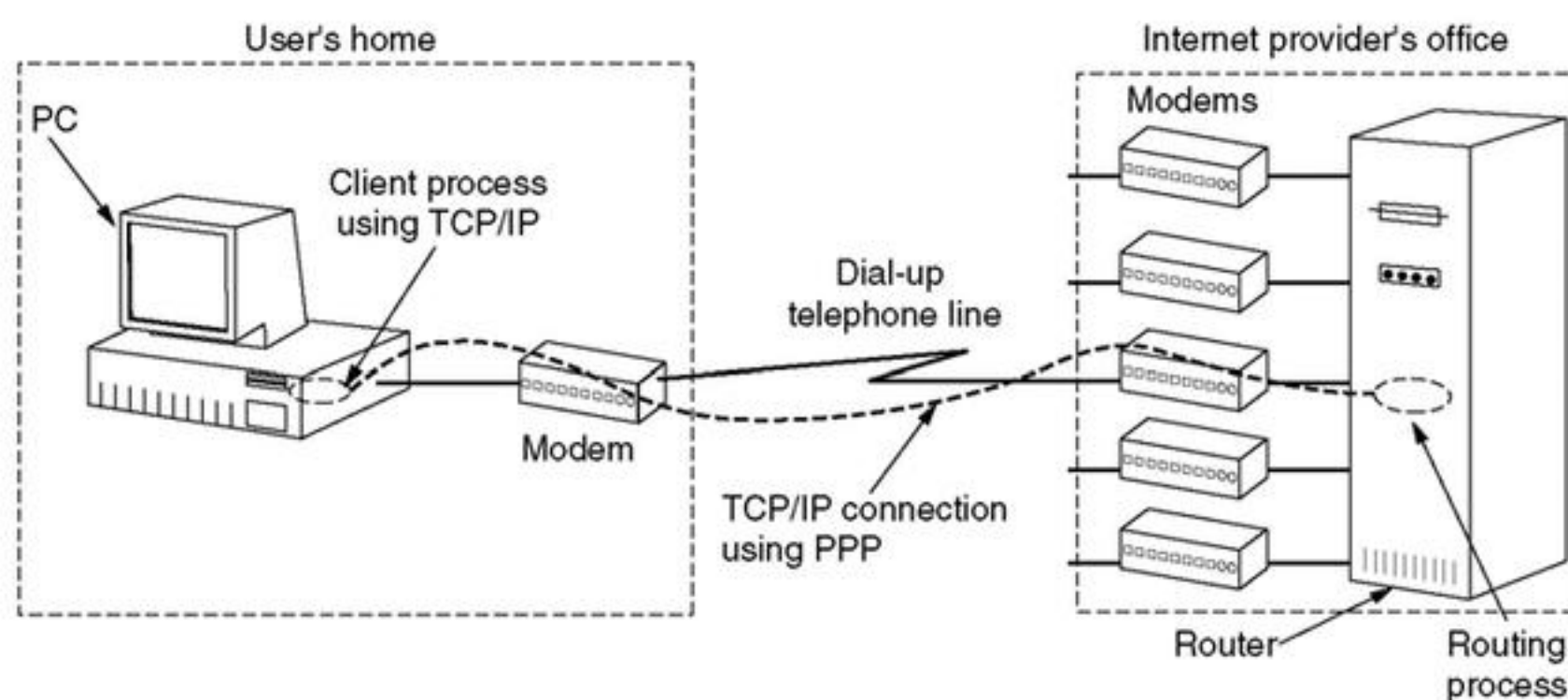
H4.15 Sơ đồ nối kết của giao thức PPP
