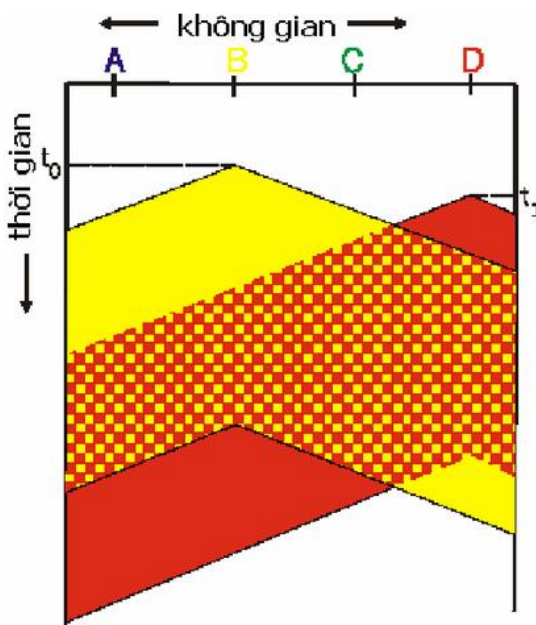
H5.9 Mô tả không gian và thời gian diễn ra đụng độ
