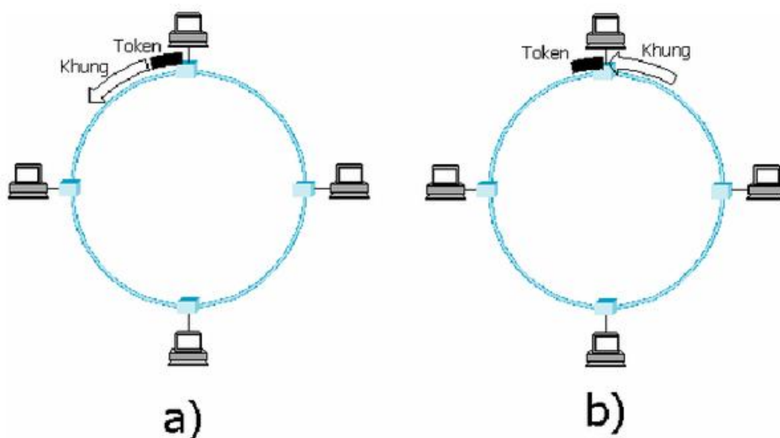
H5.16 Nhả token: a)RAT b)RAR
