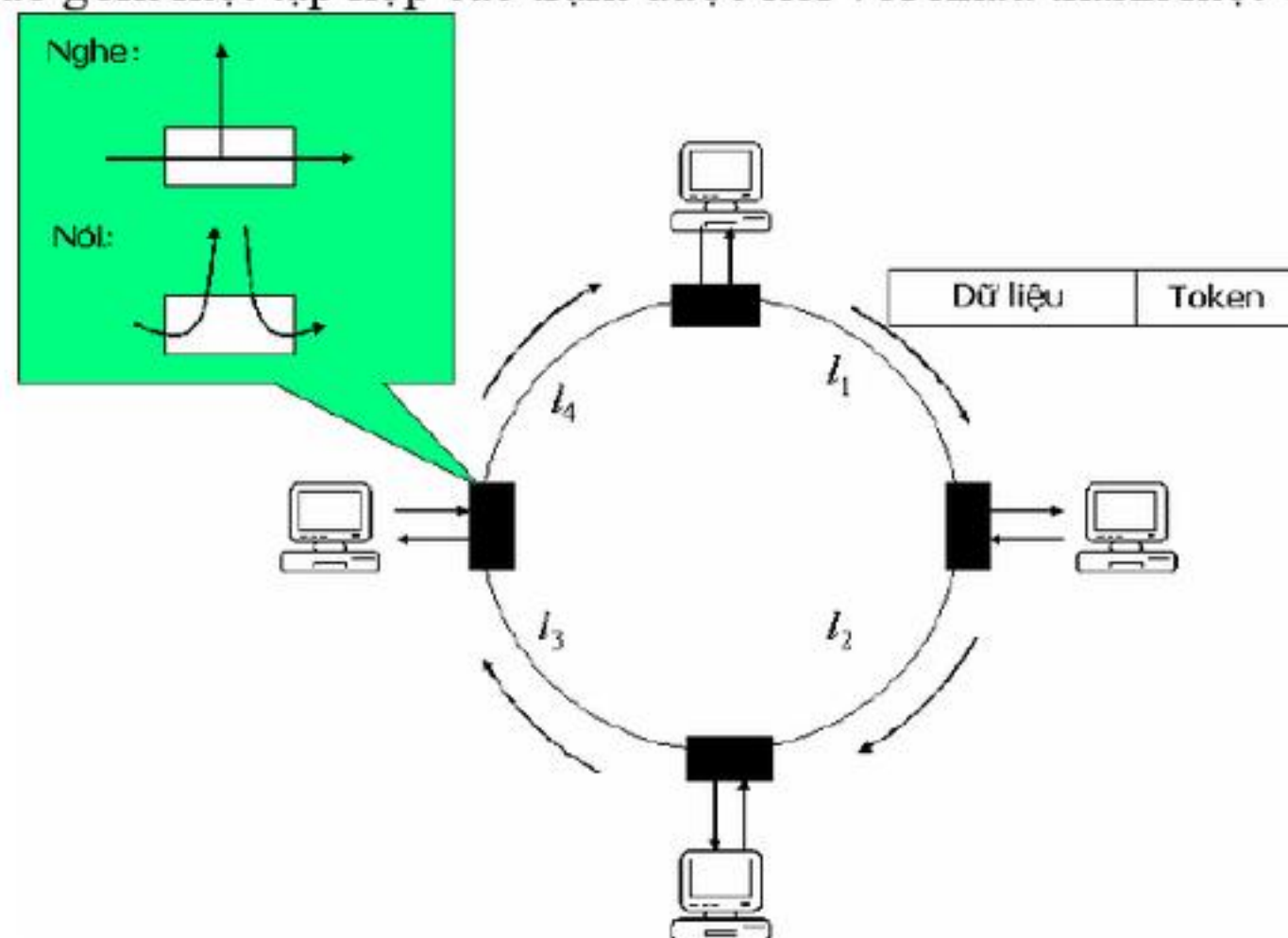
H5.15 Mô hình hoạt động của mạng Token Ring
