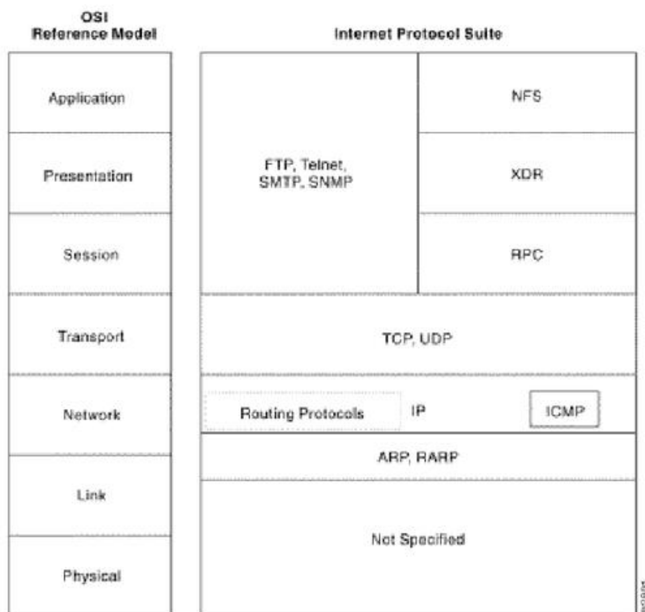
H6.29 Kiến trúc của mạng TCP/IP so với mô hình OSI
