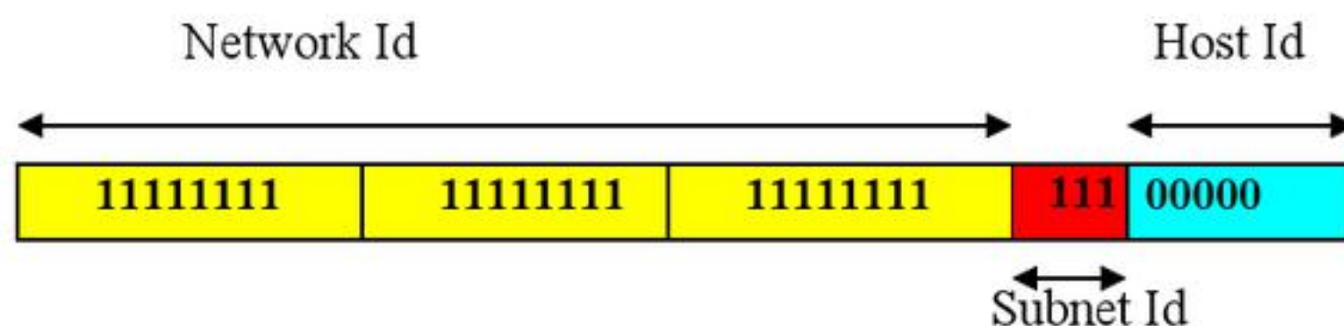
H6.34 Mặt nạ mạng con khi phân mạng con
