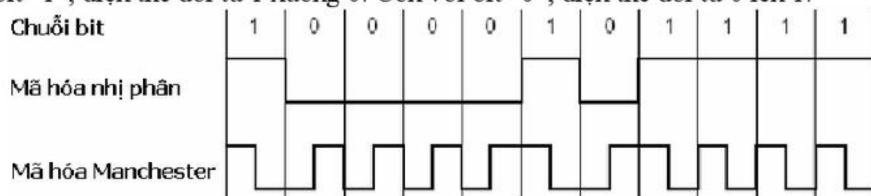
H5.30 Mã hóa Manchester
