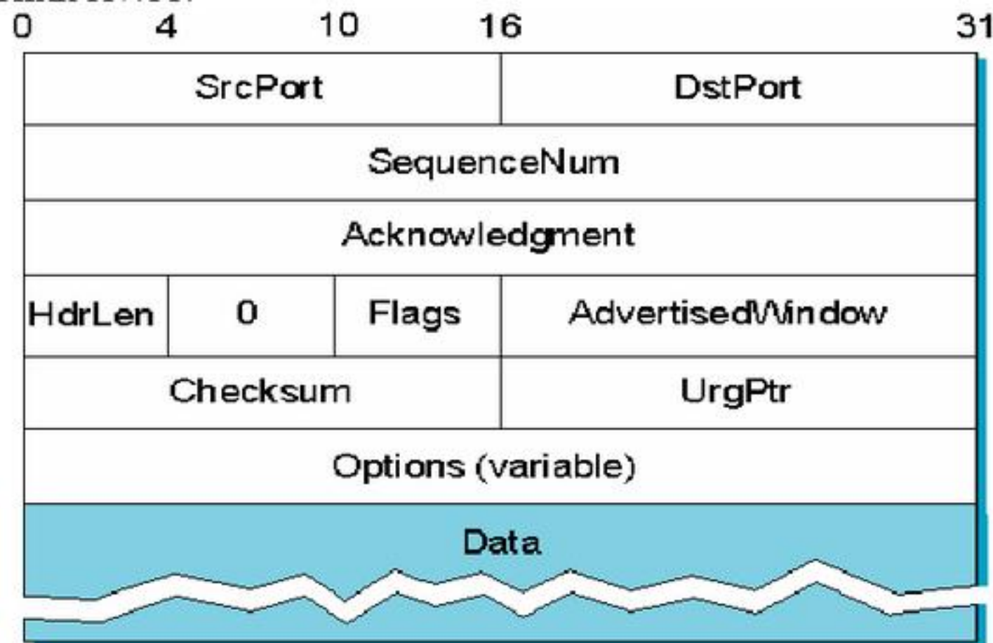
H.11 Khuôn dạng TCP header
