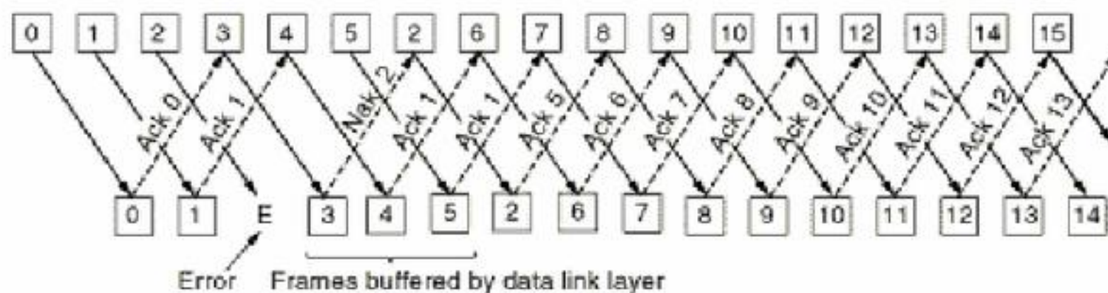
H4.11 Giao thức Selective Repeat với cửa sổ trượt lớn hơn 1
