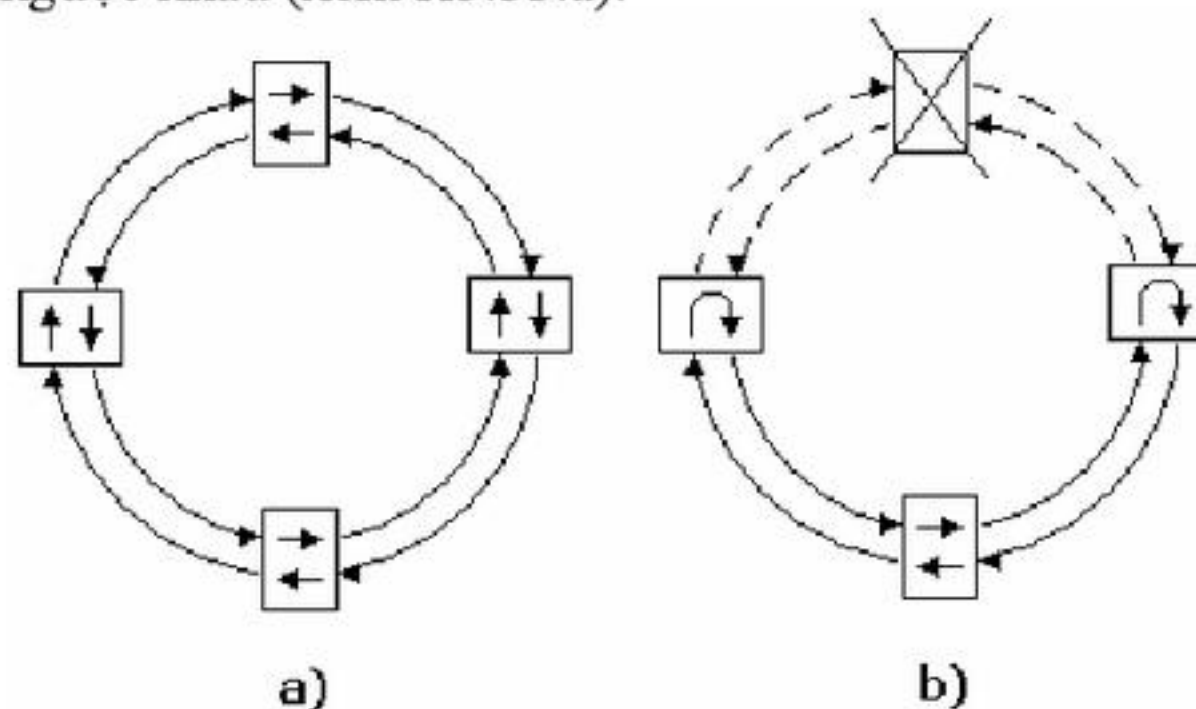
H5.33 Vòng quang đôi: a) hoạt động bình thường; b) vòng chính bị hỏng
