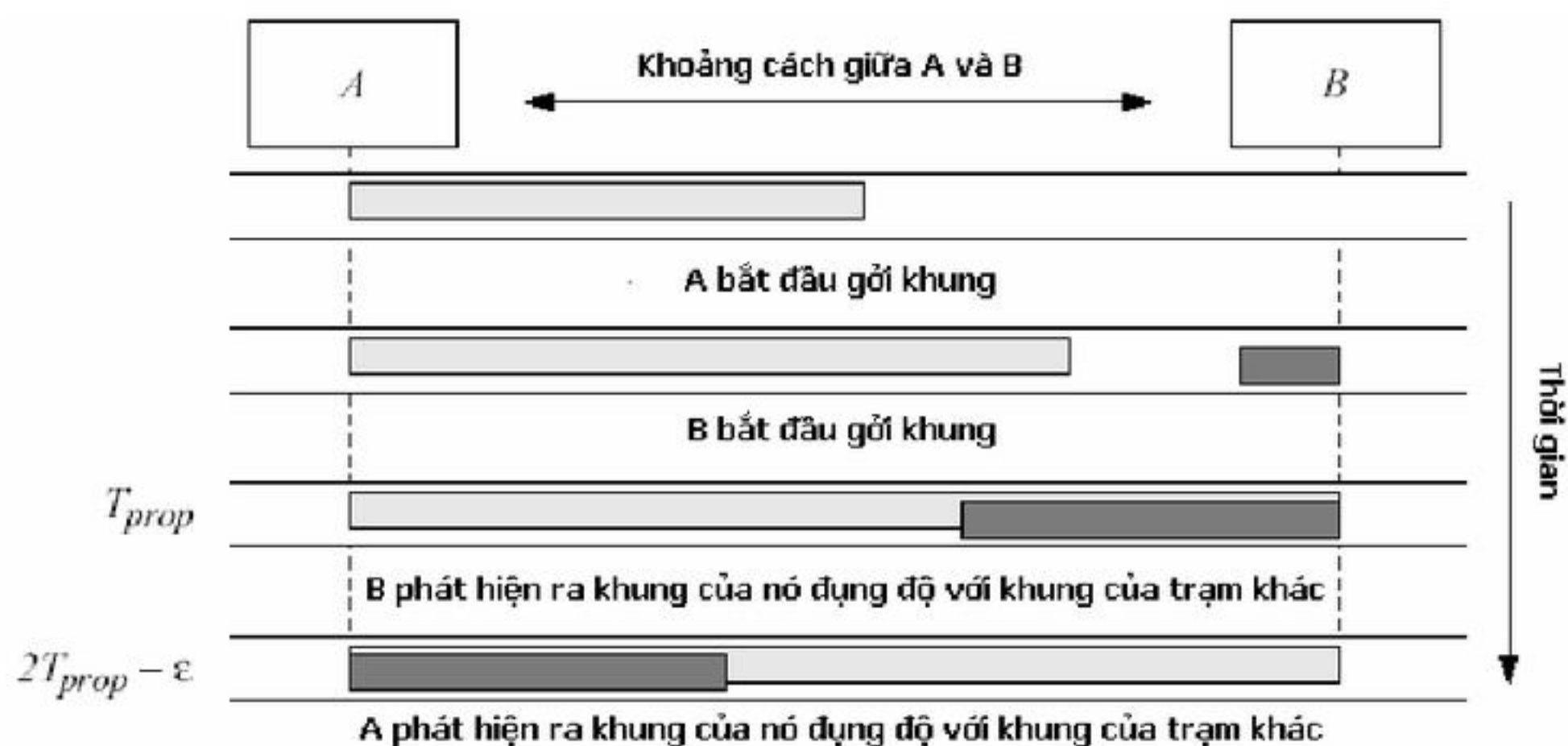
H5.12 Phát hiện đụng độ khi truyền tin
