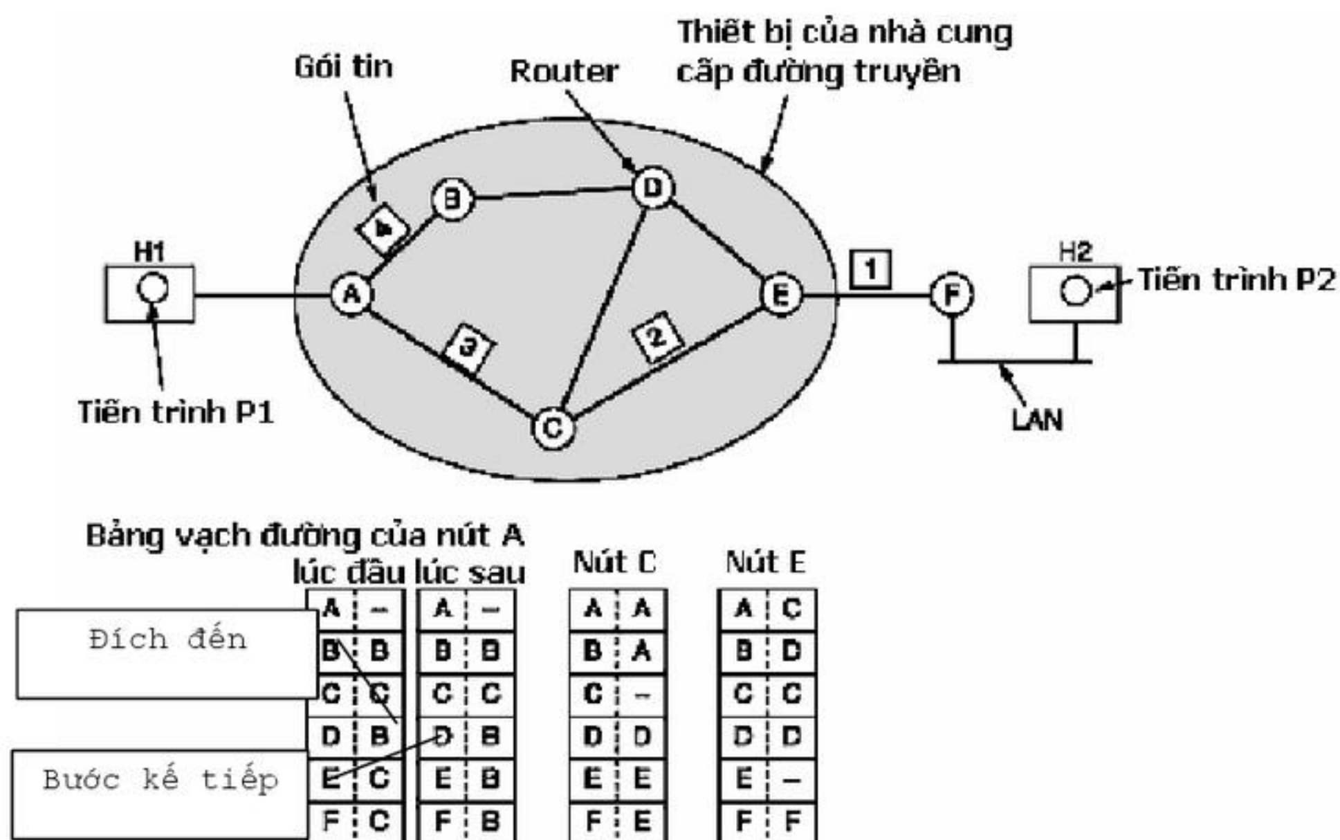
H6.2 Hoạt động của Datagram subnet
