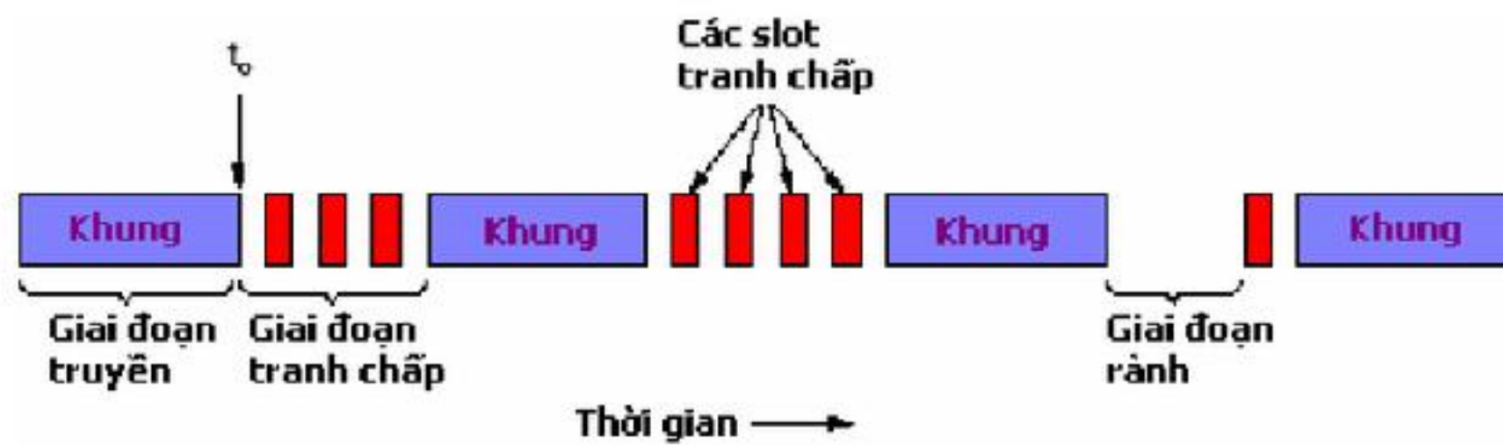
H5.10 CSMA/CD có thể ở một trong ba trạng thái: tranh chấp, truyền, rảnh
