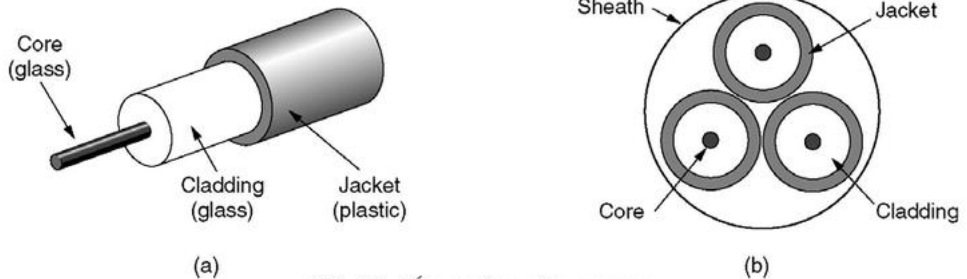
H3.13 Cấu trúc cáp quang
