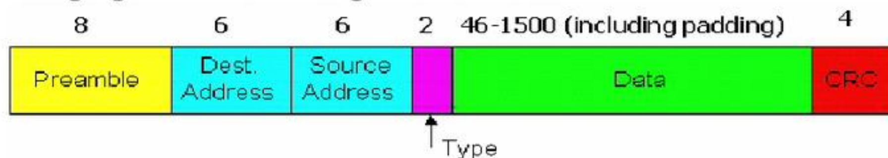
H5.29 Khuôn dạng khung thông tin Ethernet
