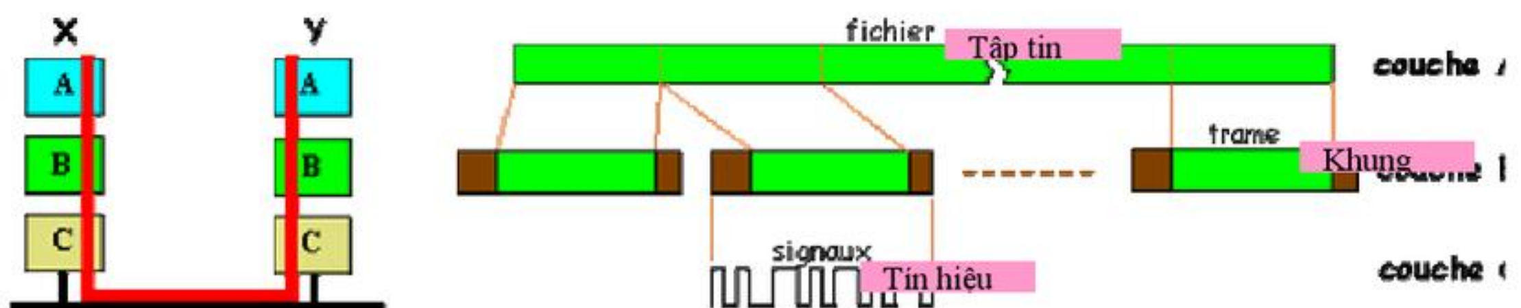
H2.12 Đơn vị truyền dữ liệu qua các tầng
