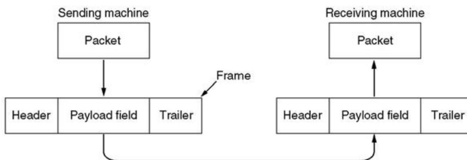
H4.1 Vị trí và chức năng của tầng liên kết dữ liệu
