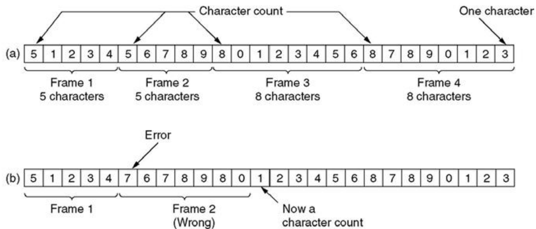
H4.2 Định khung bằng phương pháp đếm ký tự
