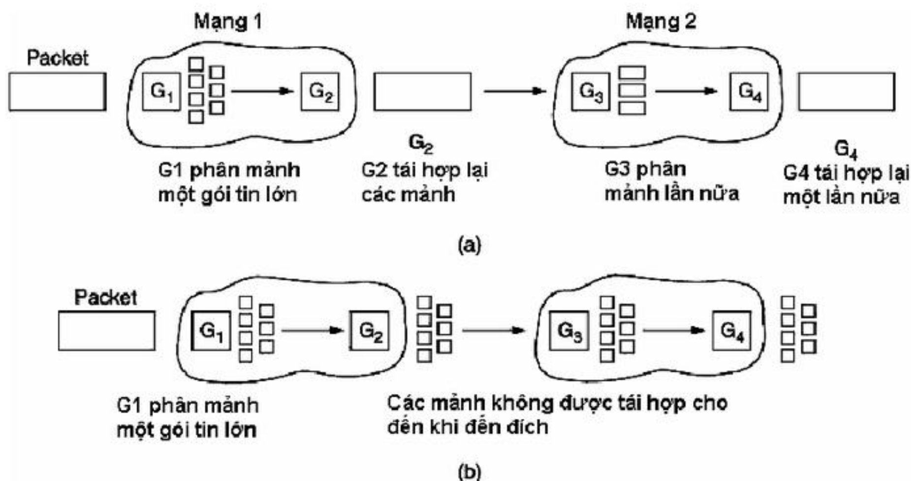
H6.27. (a) Sự phân mảnh trong suốt. (b) Sự phân mảnh không trong suốt
