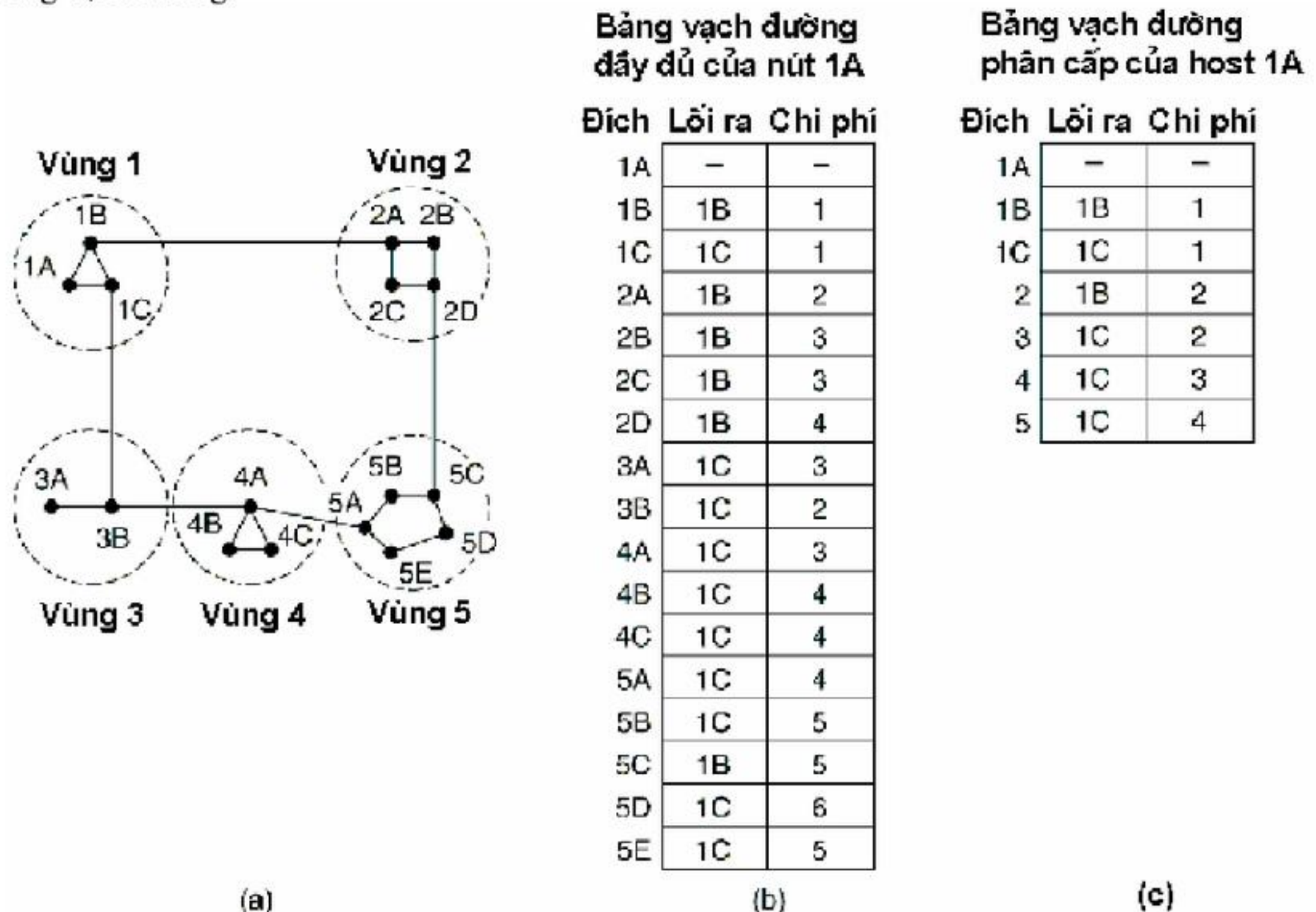
H6.16 Vạch đường phân cấp
