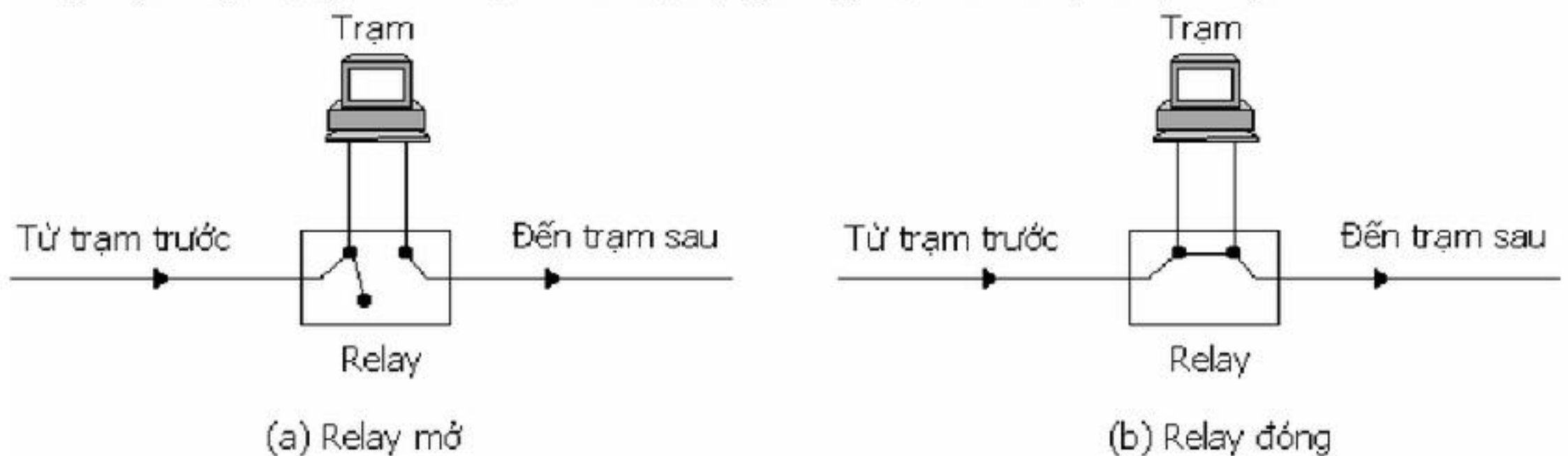
H5.17 Sử dụng relay để tránh đứt vòng
