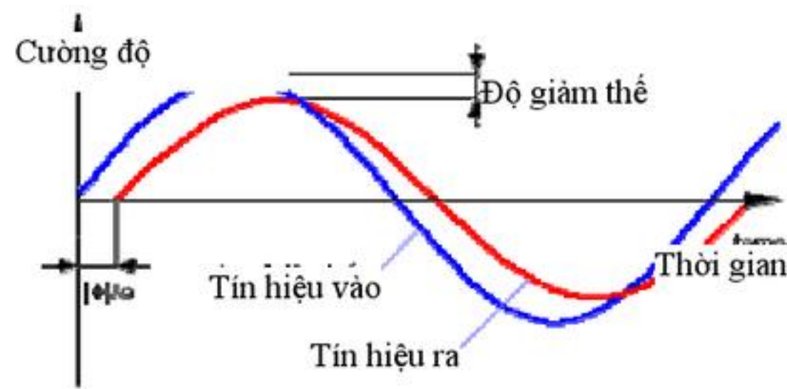
H3.19 Sự trễ pha và giảm thế của tín hiệu ngõ ra
