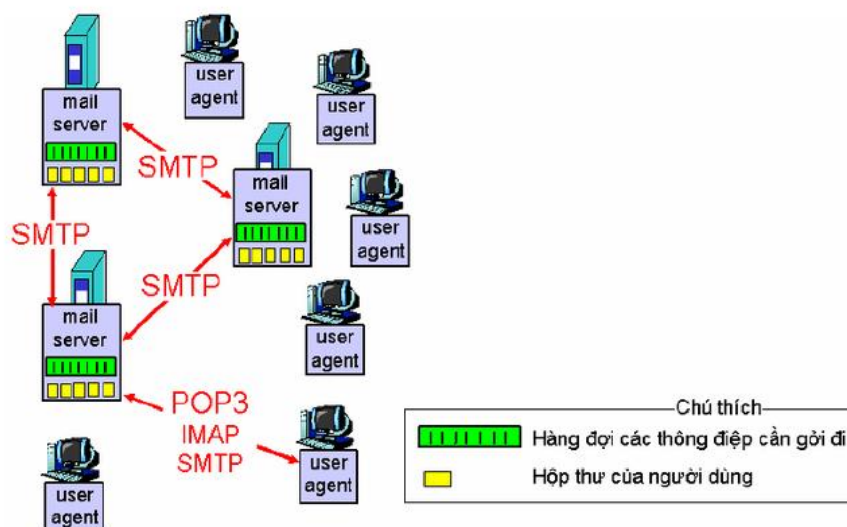
H8.6 Các thành phần của hệ thống email
