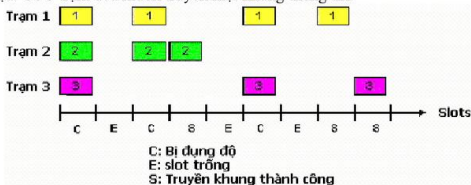
H5.7 Minh họa giao thức Slotted ALOHA
