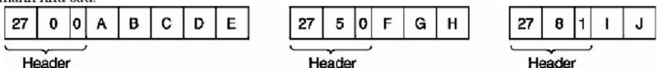
H6.28(c) Gói tin bị phân làm 3 mảnh.
