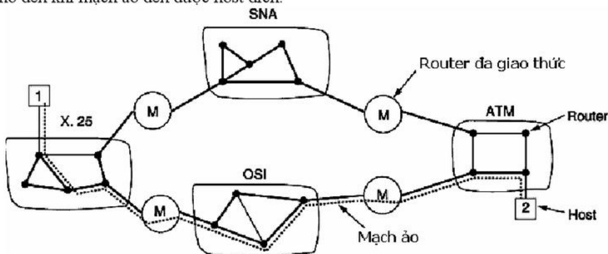
H6.24 Liên mạng dạng mạch ảo
