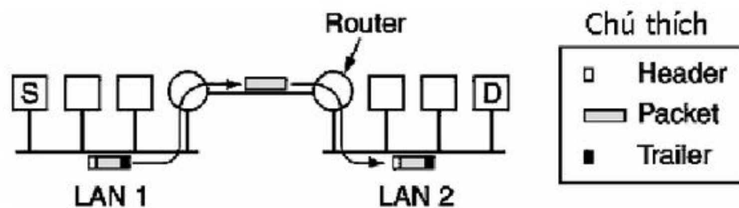
H6.23. Hai mạng Ethernet được nối kết bằng các routers
