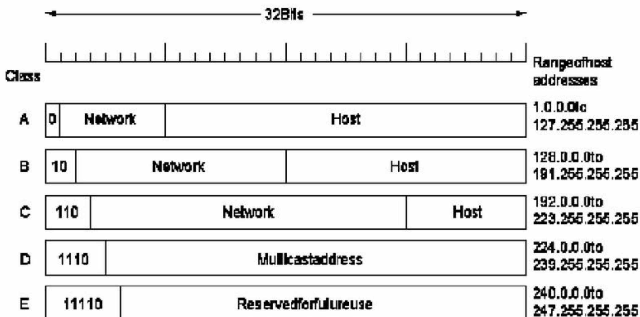
H6.32 Phân lớp địa chỉ IP
