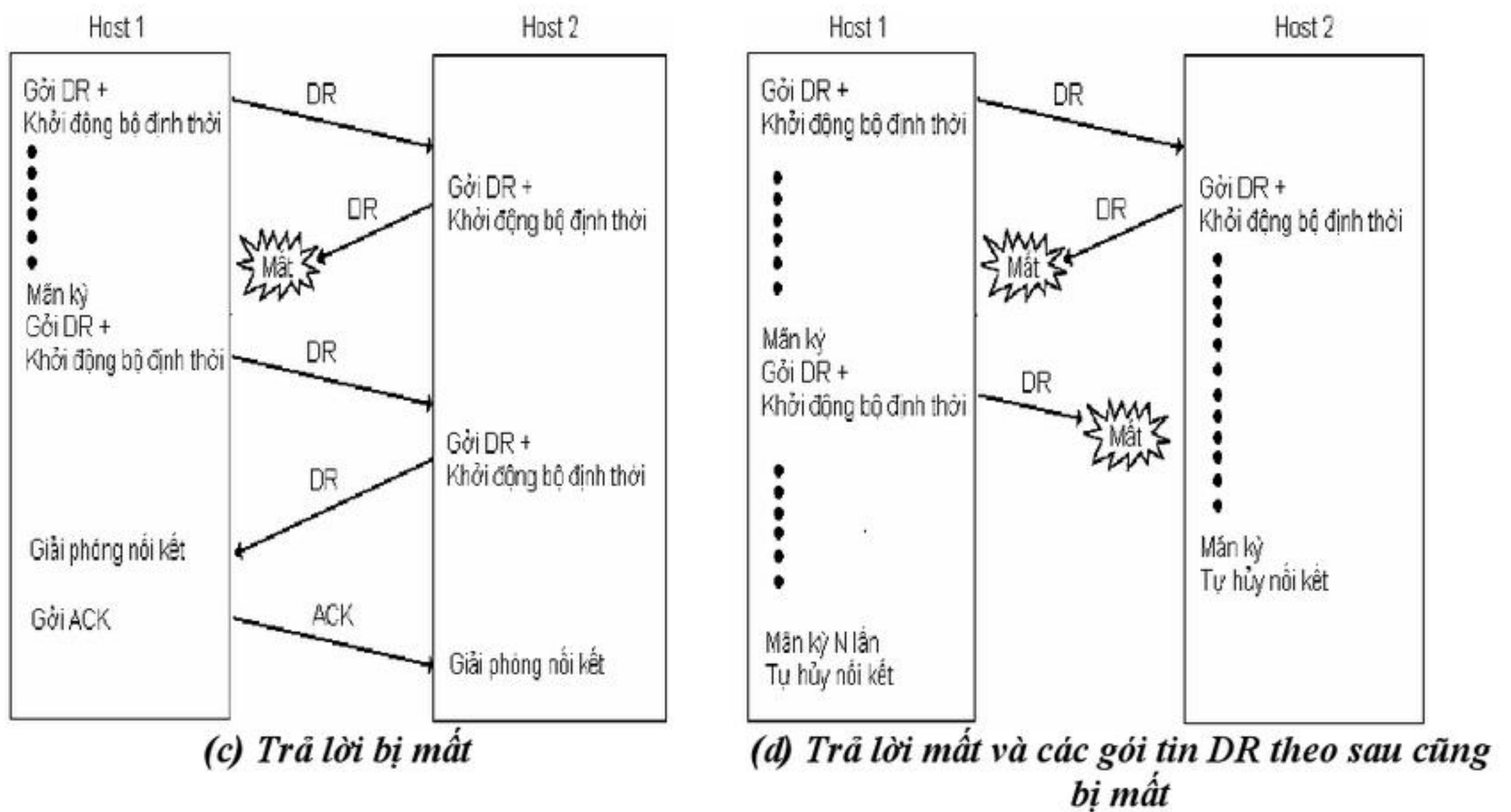
H7.7 Một số tình huống hủy nối kết theo phương pháp 3 chiều
