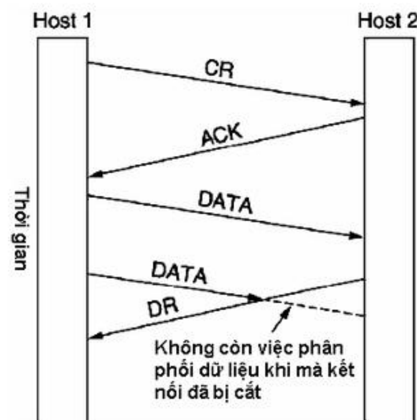
H7.5 Sự cắt kết nối một cách thô lỗ sẽ dẫn đến mất dữ liệu
