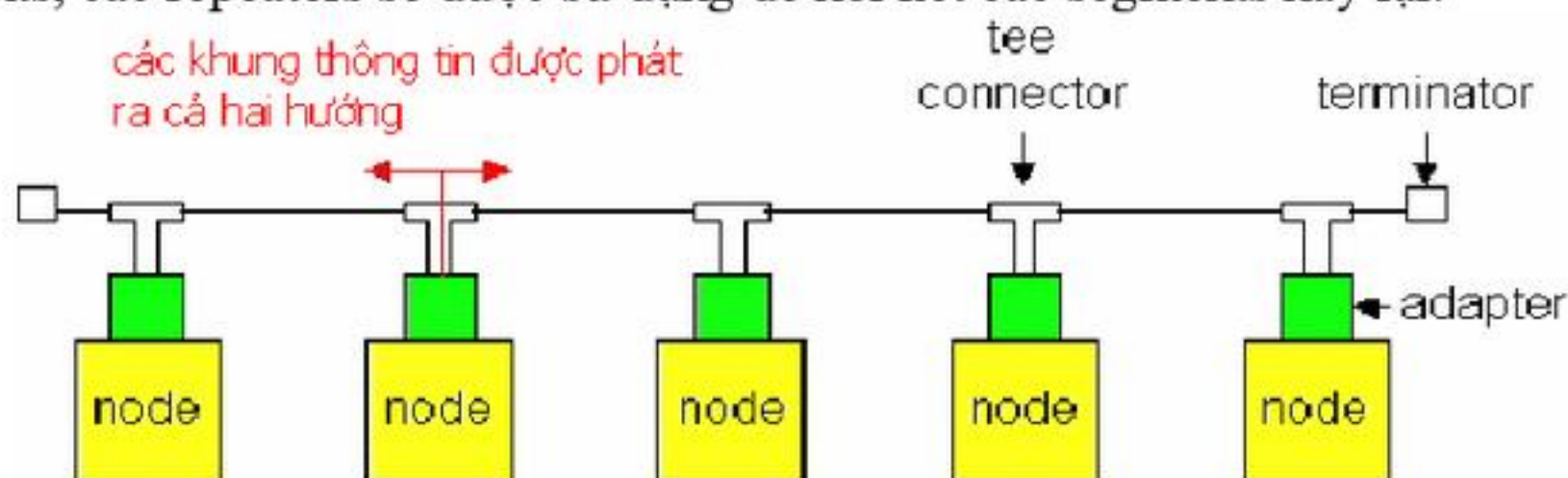
Hình 2.31 Mô hình mạng 10BASE2
