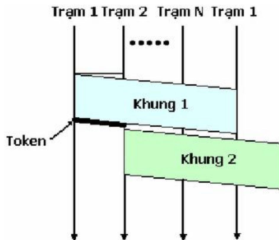
H5.21 Mô phỏng kỹ thuật RAT
