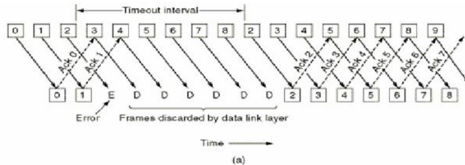
H4.10 Giao thức Go-Back-N
