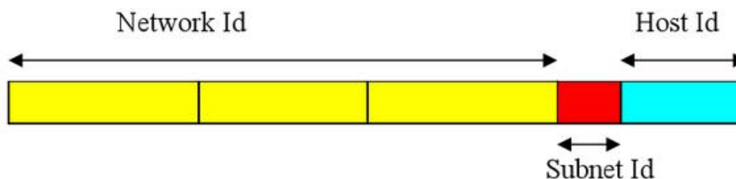
H6.33 Cấu trúc địa chỉ IP khi phân mạng con
