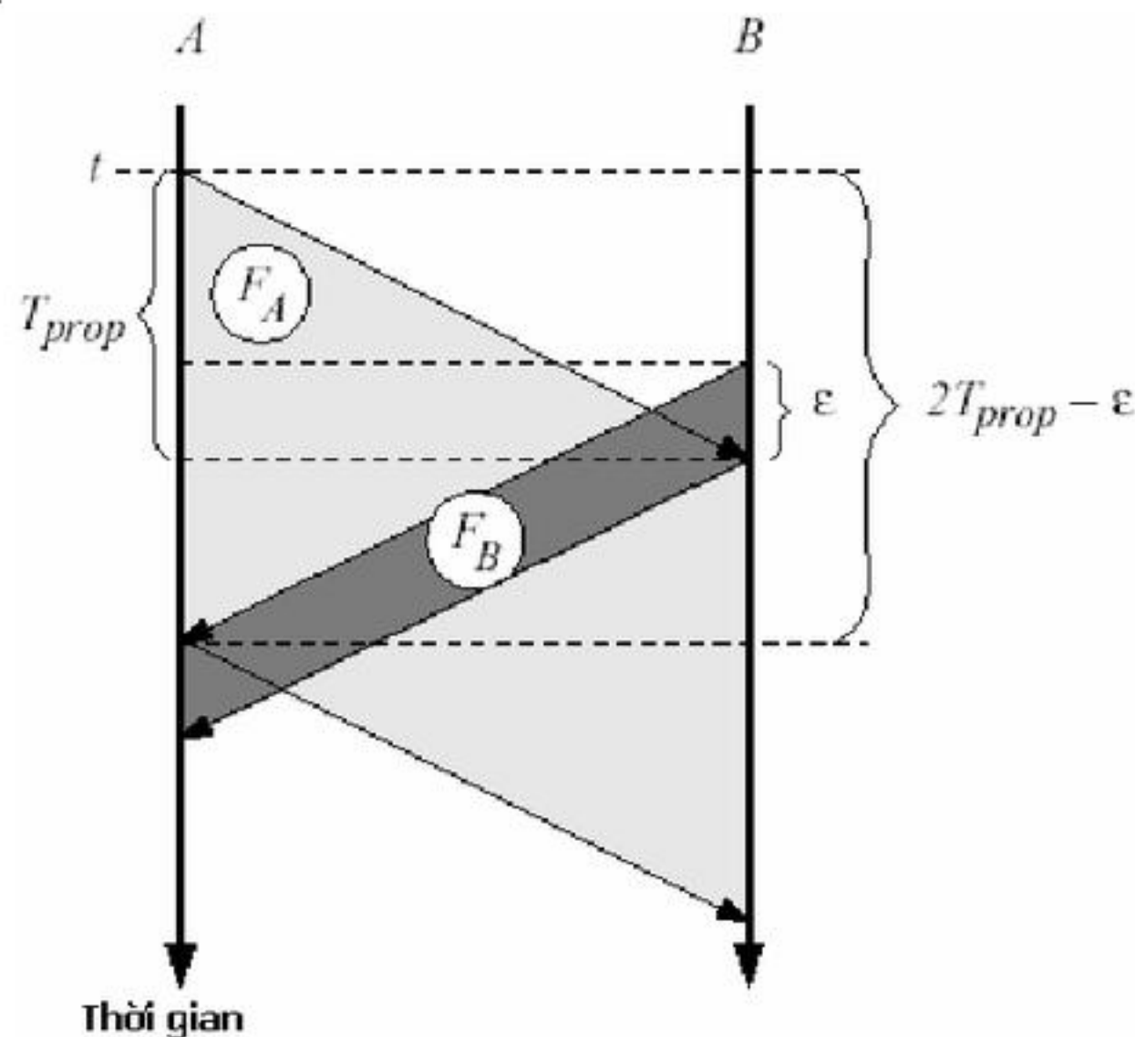
H5.11 Thời gian cần thiết để truyền một khung
