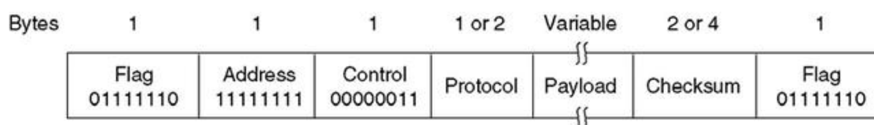
H4.16 Cấu trúc khung của giao thức PPP
