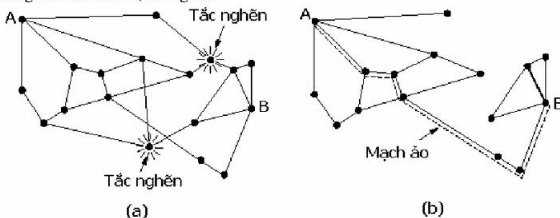
H6.20 (a) Một mạng con bị tắc nghẽn. (b) Mạng con được vẽ lại sau khi loại trừ các điểm gây tắc nghẽn.
