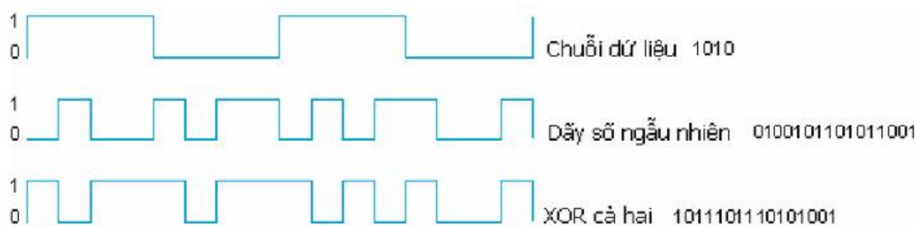
H5.36 Ví dụ về mã cắt lát 4 bit.
