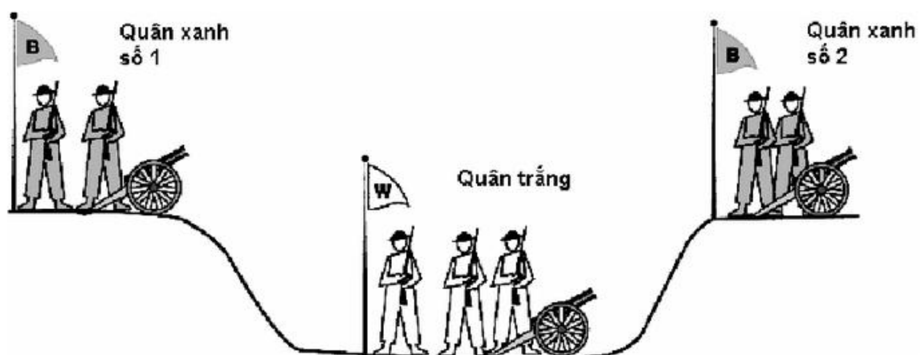
H7.6 Bài toán hai sứ quân
