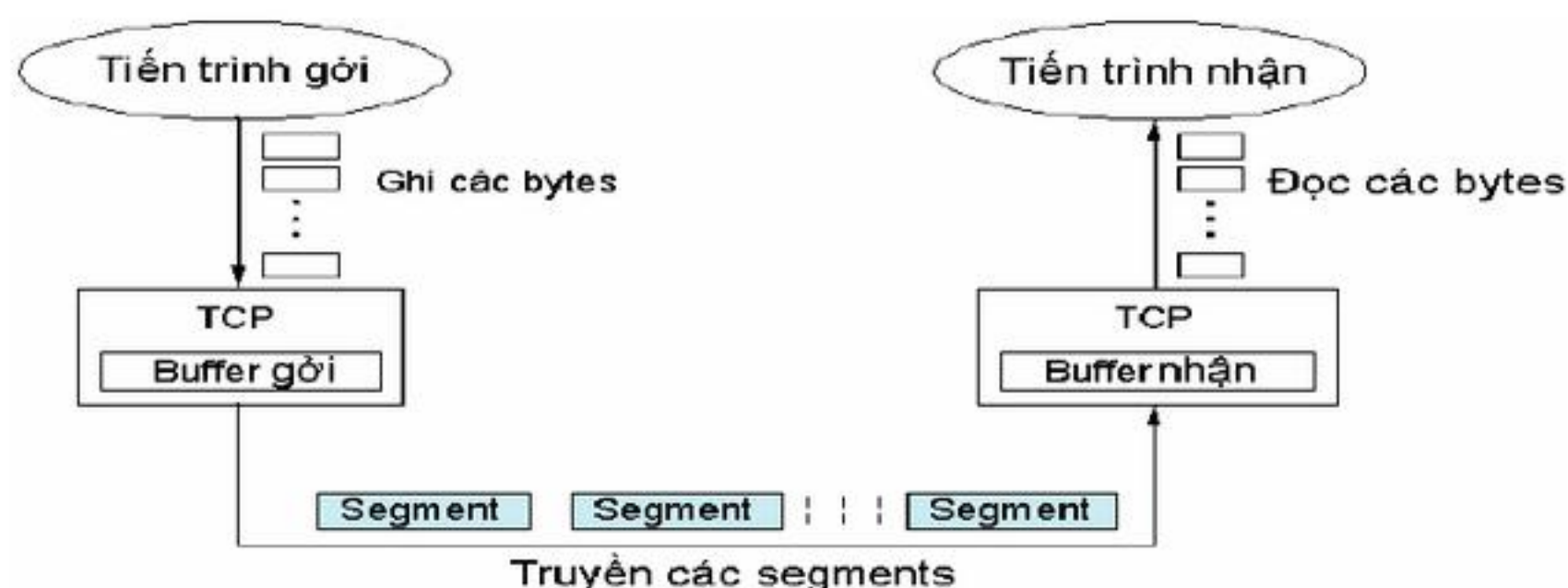
H7.10. Cách thức TCP quản lý luồng các bytes
