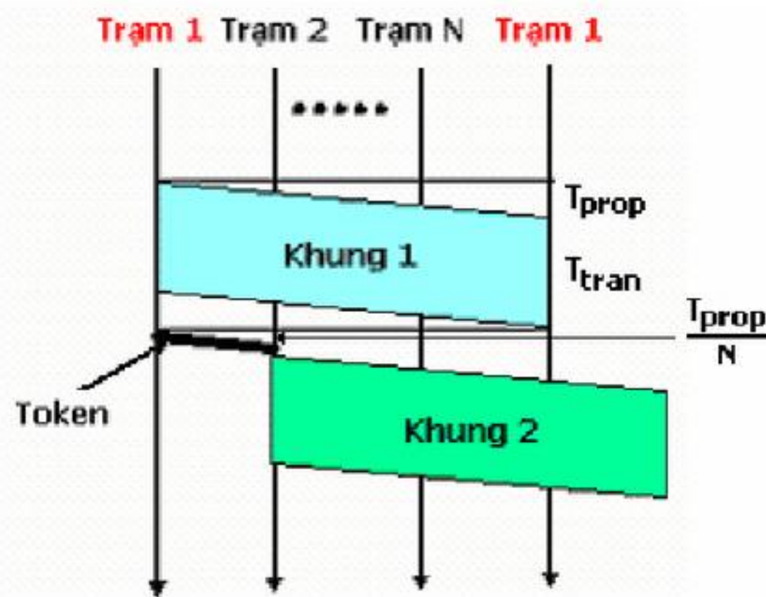
H5.20 Các khoảng thời gian một trạm phải trải qua khi gửi dữ liệu và chuyển thẻ bài
