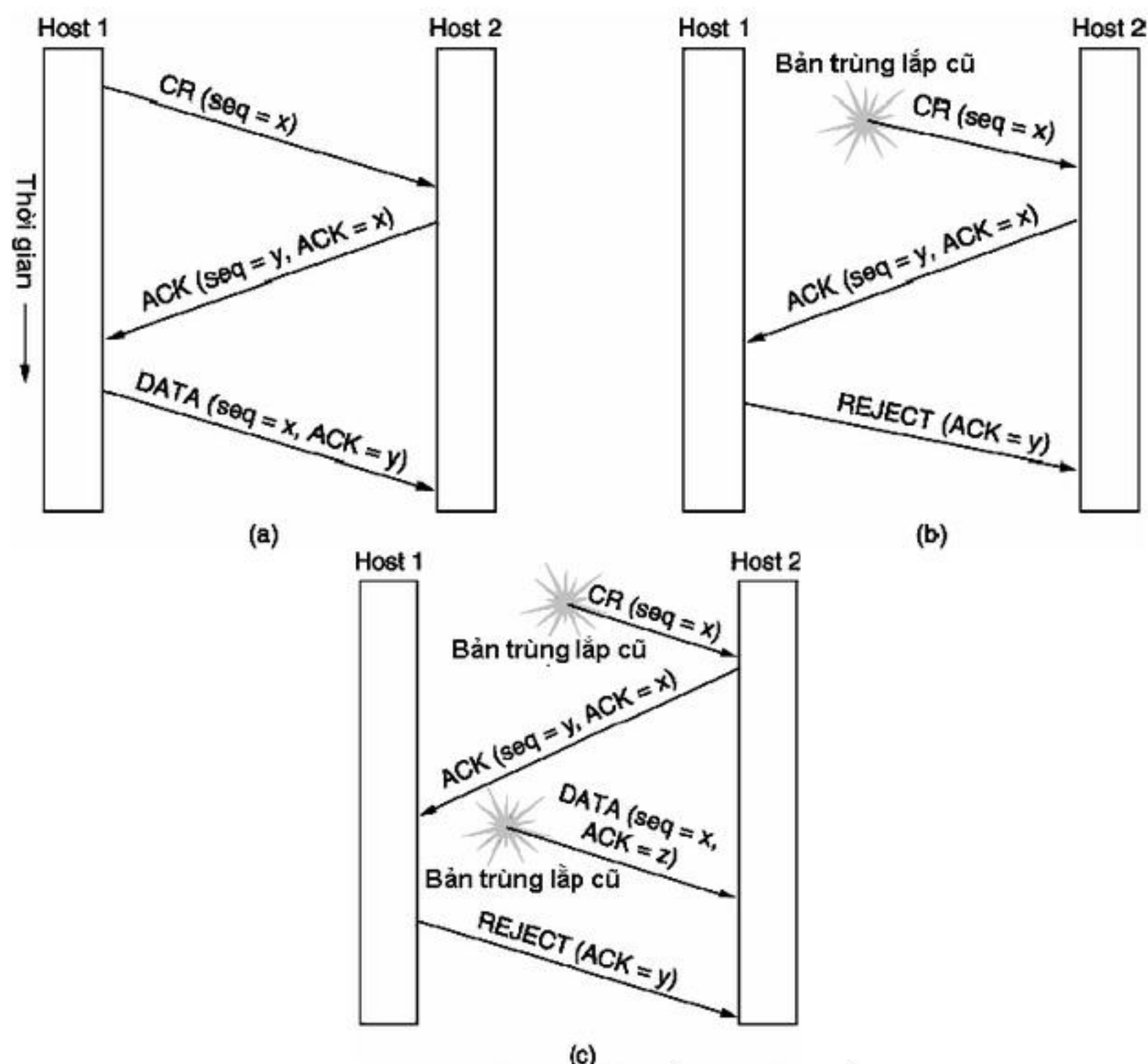
H7.4 Khung cảnh việc bắt tay 3 chiều.
