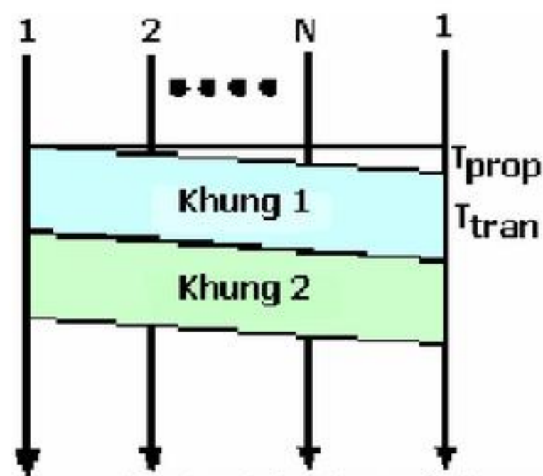
H5.22 Thời gian phát và lan truyền khung
