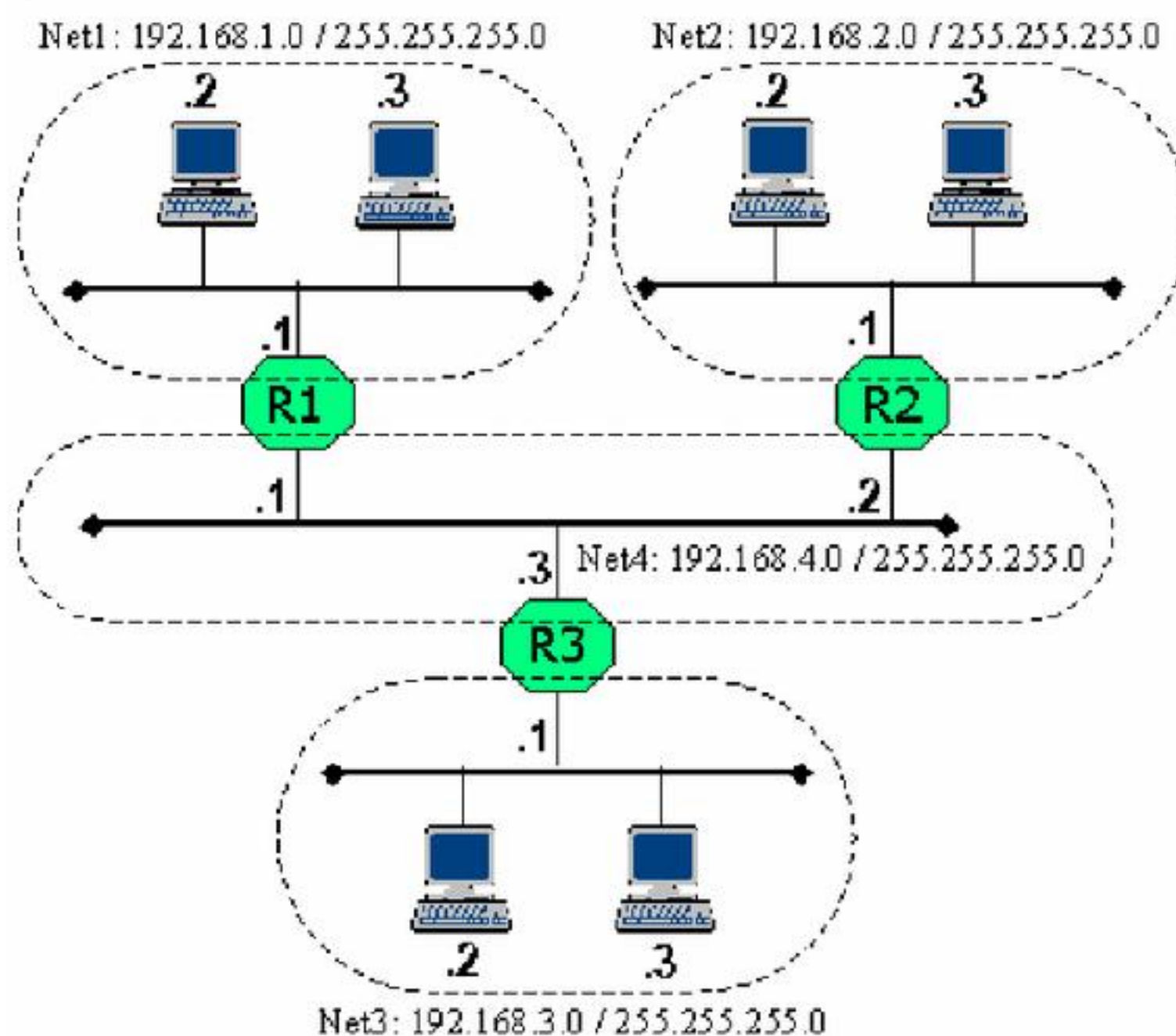
H6.36 Ví dụ về liên mạng một liên mạng sử dụng giao thức IP
