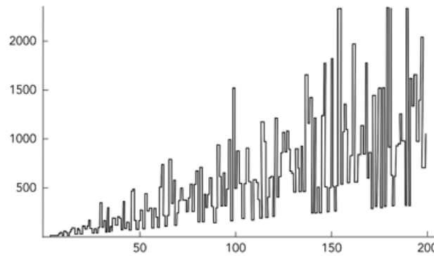
Зависимость числа простых чисел между p_n^2 и p_{n+1}^2 от n (Eric W. Weisstein, «Brocard's Conjecture», с сайта MathWorld — http://mathworld.wolfram.com/BrocardConjecture.html )
