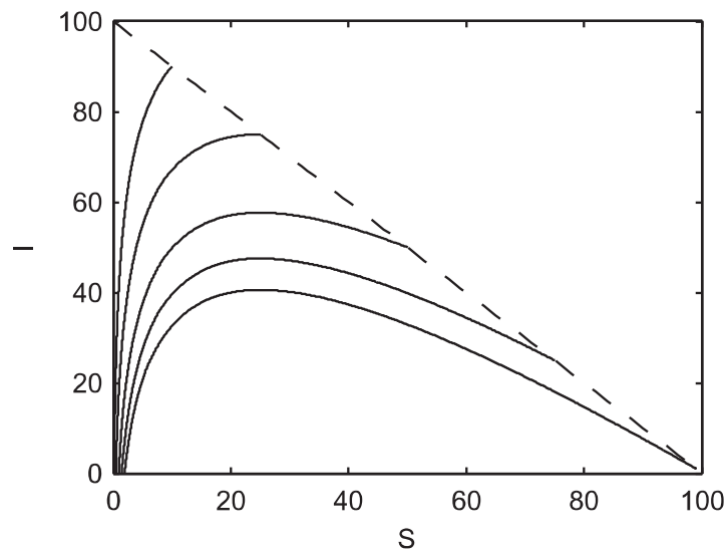
Hình 4: Nghiệm số của mô hình SIR của phương trình (6.2.1) – (6.2.3), đường nét đứt là S + I = S_0 + I_0 , đường trơn là quỹ đạo pha, r = 0.01 , a = 0.25
