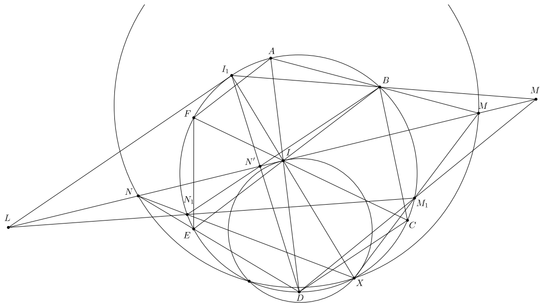
Hình 10. Tính chất 3
