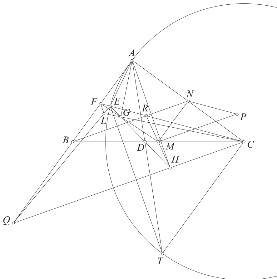
Hình 6.
