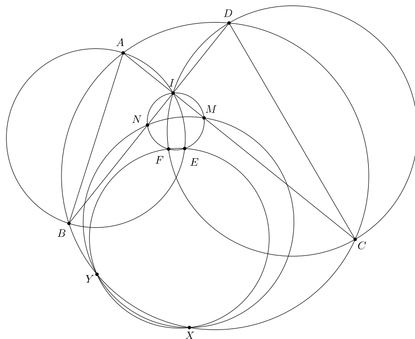
Hình 8. Tính chất 1
