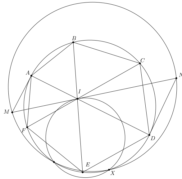
Hình 15. Bài toán 6
