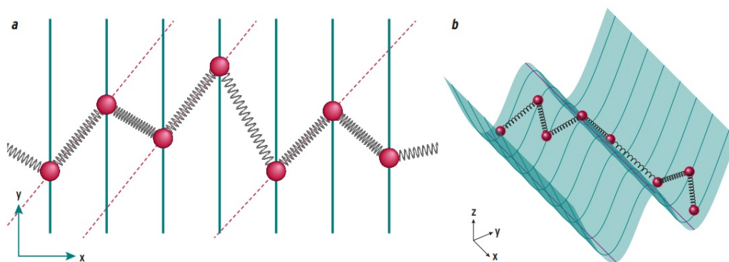
Hình 2: Chuỗi hạt cứng và mayonnaise. Các hạt gắn với nhau bởi lò xo có thể chuyển động tự do theo phương y nhưng bị cố định theo phương x với một khoảng cách đều nhau (a). Khi chiều dài lò xo ngắn lại, ngắn hơn khoảng cách nhỏ nhất giữa các hạt, chúng sẽ có xu hướng xếp thành hàng (đường nét đứt). Đặt chuỗi hạt này lên một tấm tôn (b). Mỗi hạt cứng sẽ bị thu hút bởi các hạt lân cận của nó và bởi rãnh tấm tôn. Khi số hạt tăng lên vô hạn, sự chuyển động của chuỗi hạt được mô tả bởi phương trình Allen - Cahn một chiều.
