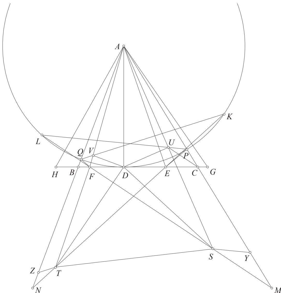
Hình 13.
