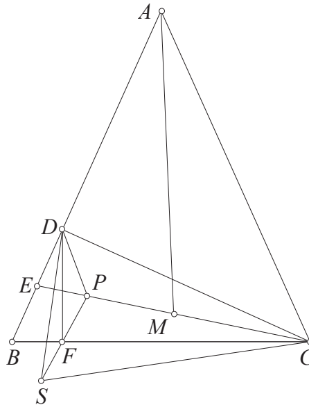
Hình 4.
