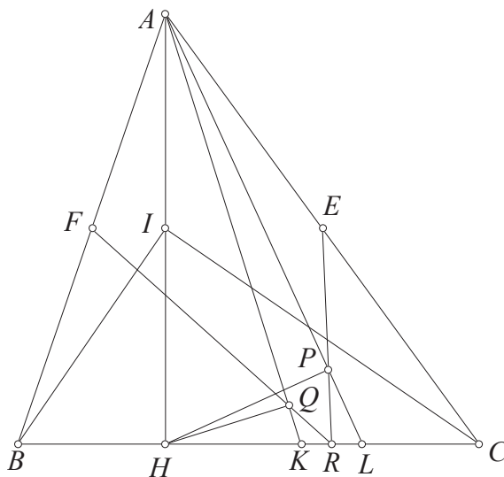
Hình 16.
