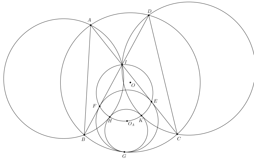
Hình 13. Bài toán 4
