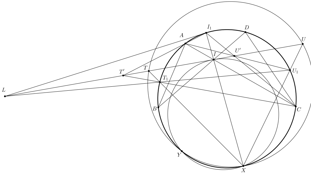
Hình 9. Tính chất 2
