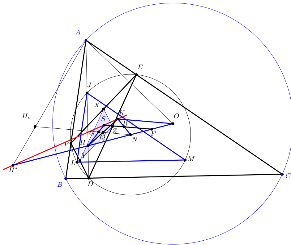
Hình 11.6: Định lý 3.1
