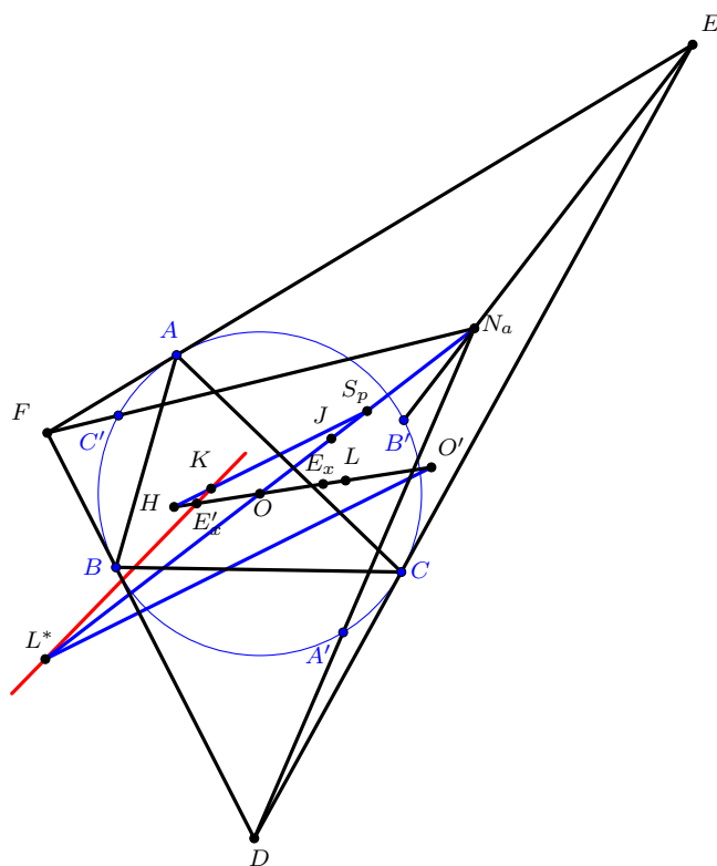
Hình 11.12: Định lý 5
