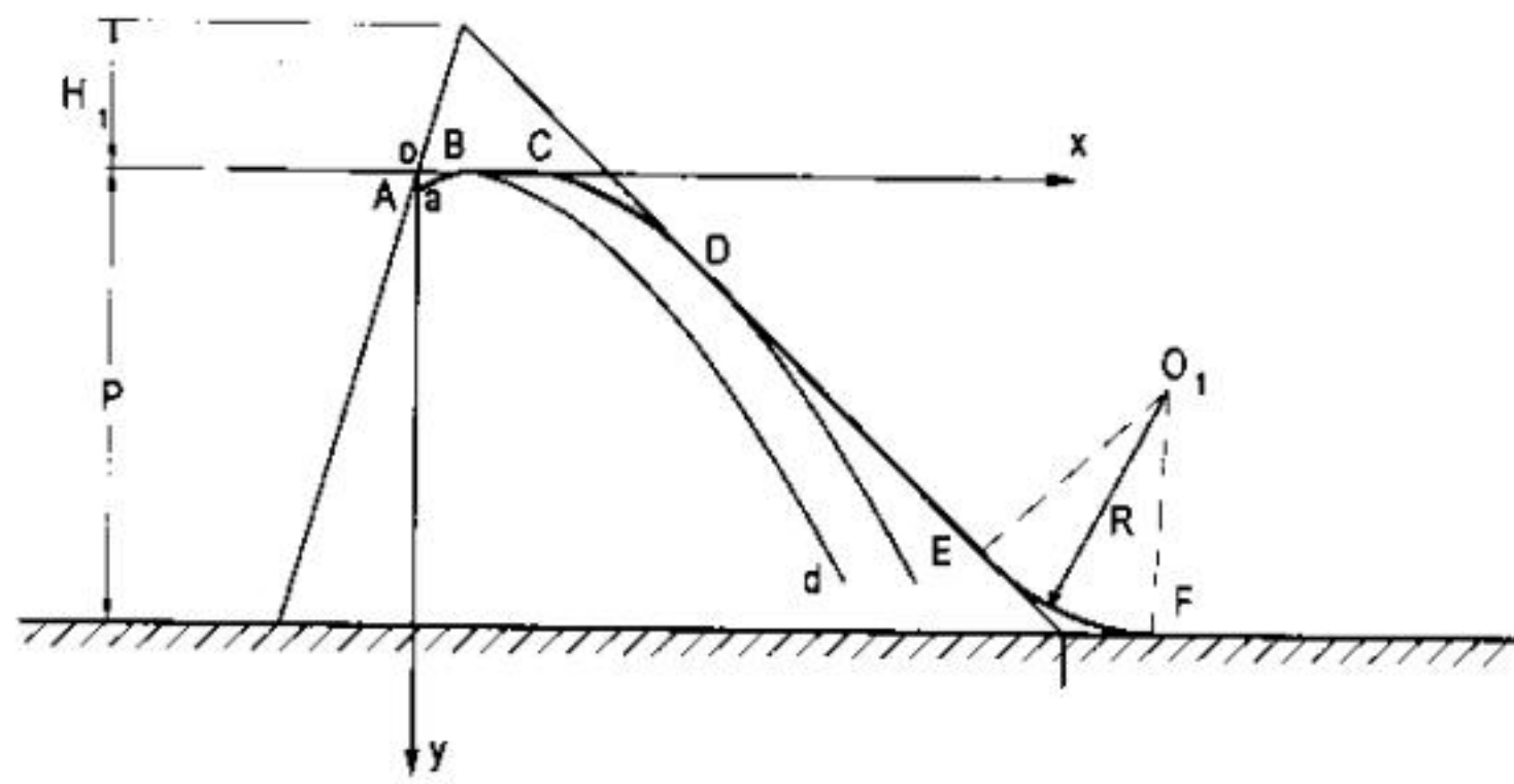
Hình 4-2. Xây dựng mặt cắt đập tràn
