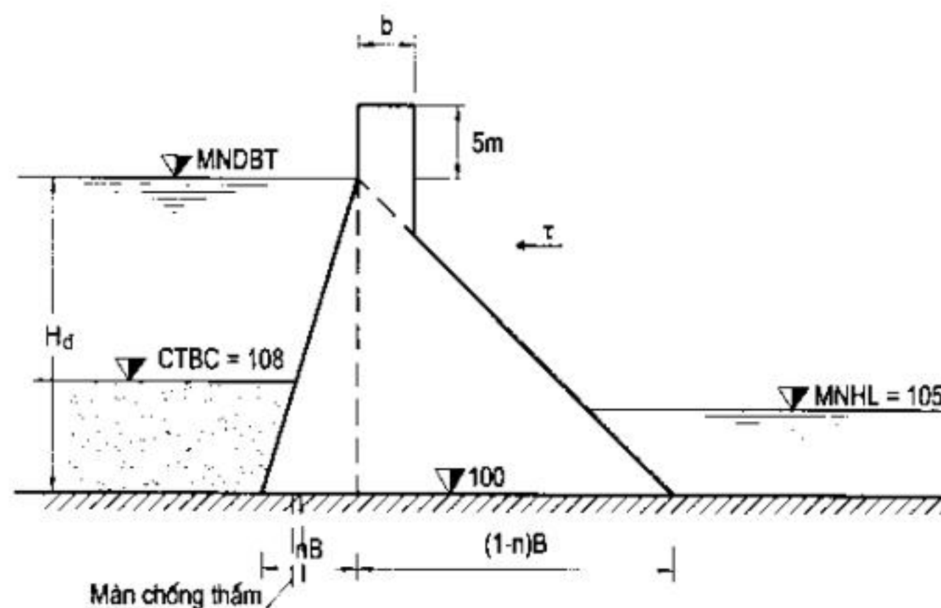
Hình A: Sơ đồ mặt cắt đập
