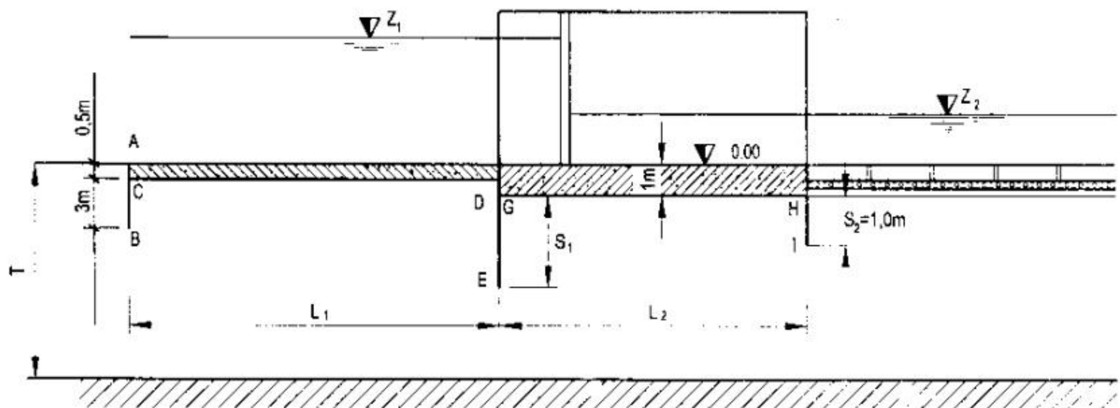
Hình C: Sơ đồ cắt dọc cống C
