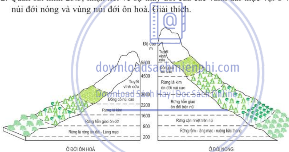
Hình 23.3 - Phân tầng thực vật theo độ cao ở đới ôn hoà và đới nóng
