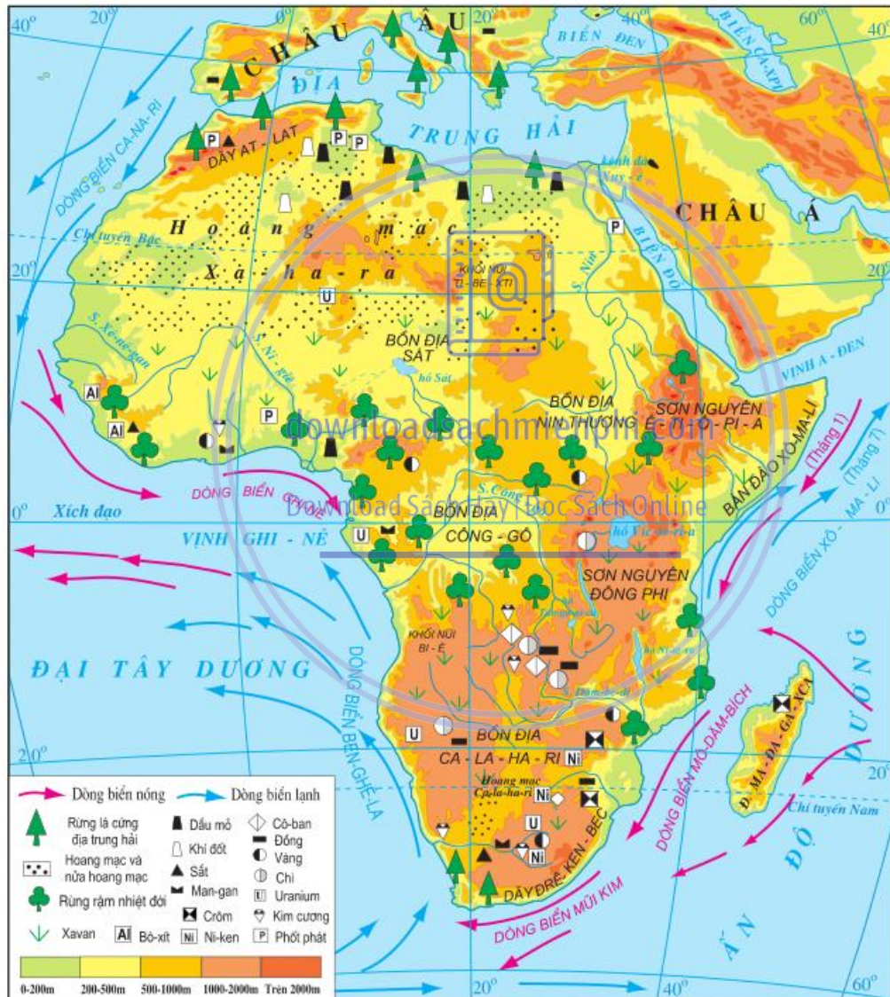
Hình 26.1 - Lược đồ tự nhiên châu Phi
