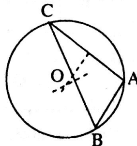
\triangle ABC có \hat{A} > 90^\circ
