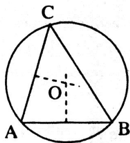
\triangle ABC nhọn
