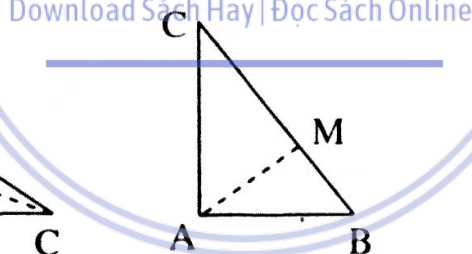
\triangle ABC vuông tại A
