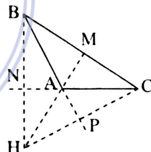
\triangle ABC có \hat{A} > 90^\circ
