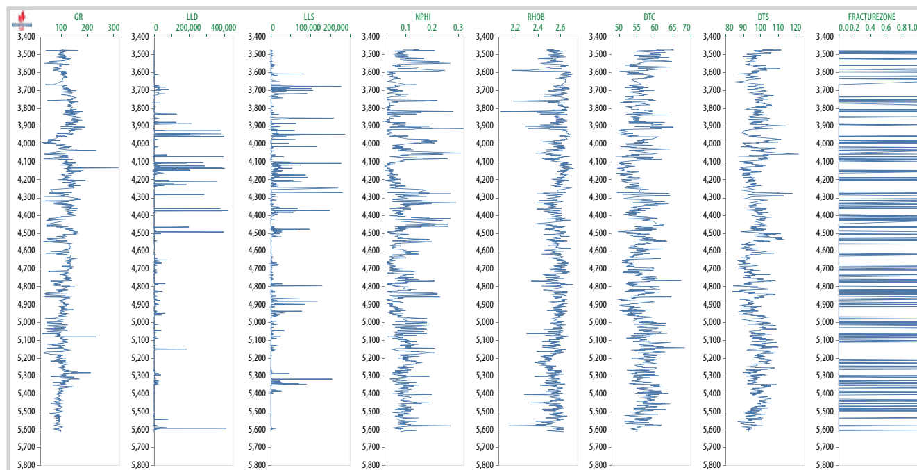
Hình 1. Kết quả dự báo đối nút nê được hiển thị cùng các đường đo ghi giếng khoan trên ứng dụng VPI-Mlogs.
