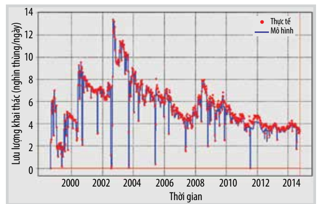
Hình 7. So sánh lịch sử khai thác dầu giữa mô hình và thực tế.
