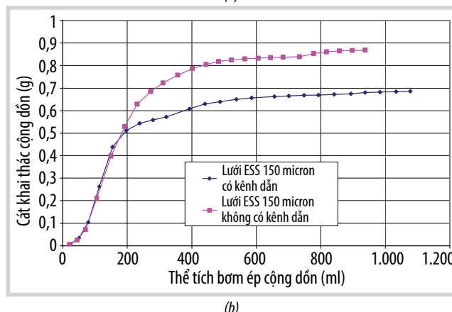
Hình 8. Hiện tượng tạo kênh dẫn (channelling) (a) và biểu đồ thể hiện sự ảnh hưởng (b) [4].
