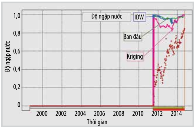
(a) (b) Hình 18. Kết quả phục hồi lịch sử giếng 1P: Độ dẫn động ban đầu (a) và sau khi điều chỉnh độ dẫn động (b).
