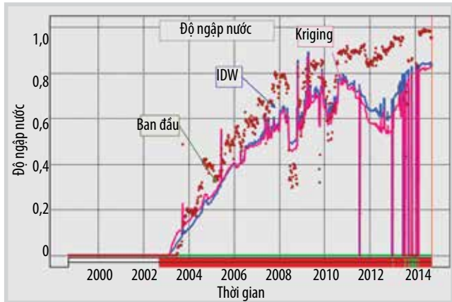
(a) (b) Hình 19. Kết quả phục hồi lịch sử giếng 6P (a) và 9P (b).
