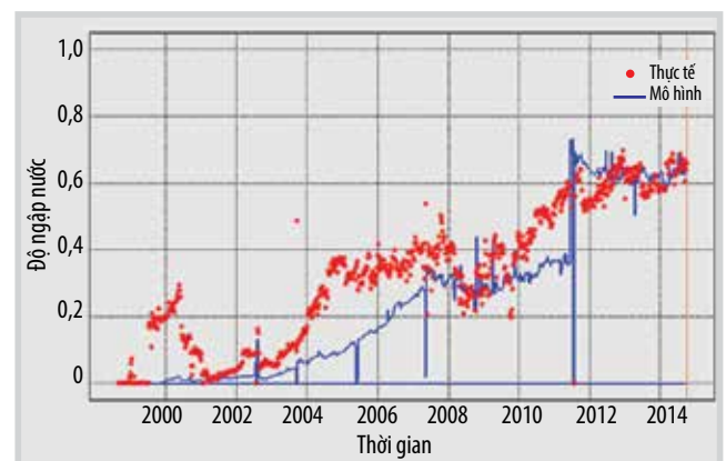
Hình 8. So sánh độ ngập nước giữa mô hình và thực tế.
