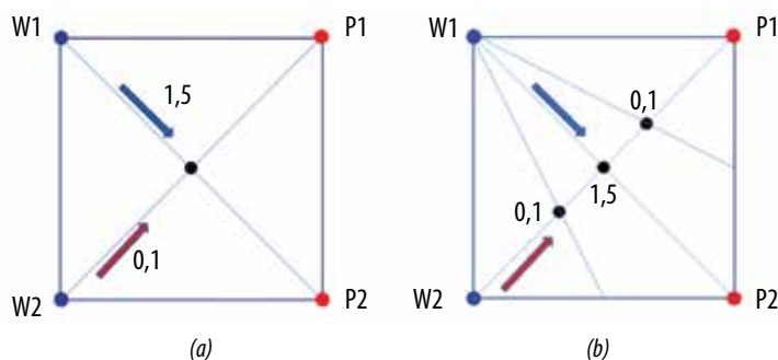
Hình 3. Mạng lưới kết nối giếng trong trường hợp điểm giả lập trùng nhau.
