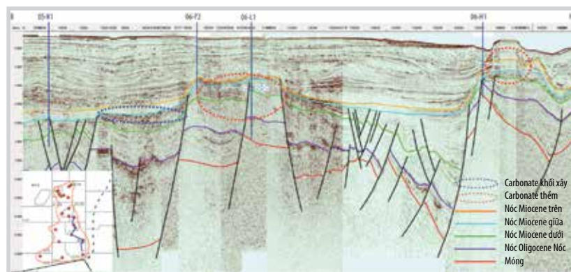
Hình 11. Các dạng đá vôi khối xây và đá vôi rìa khối xây (thềm) trên mặt cắt địa chấn qua các giếng khoan 05-K1, 06-P2, 06-L1 và 06-H1, khu vực Đông Nam bể Nam Côn Sơn [12].
