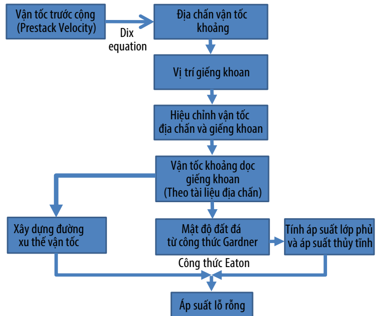
Hình 6. Các bước tiến hành xác định áp suất lỗ rỗng từ tài liệu vận tốc khoảng.
