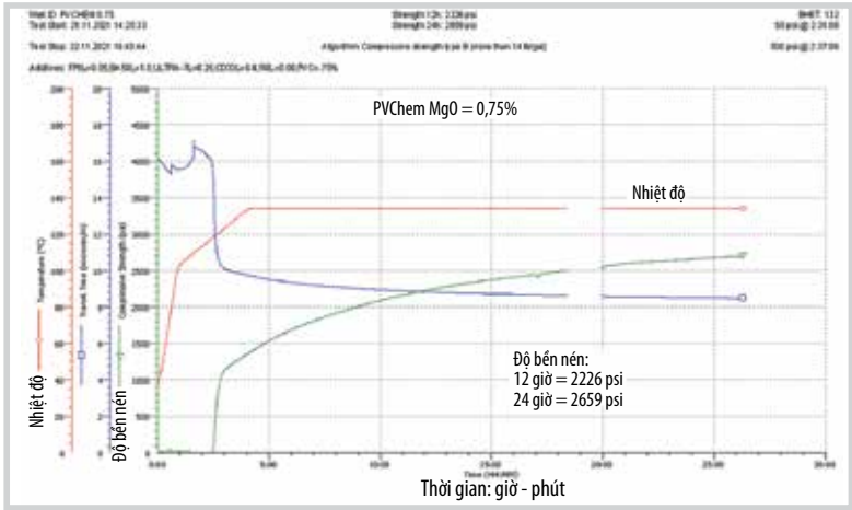
Hình 11. Biểu đồ độ bền nén của đơn vũ xi măng chứa 0,75% phụ gia PVChem MgO.
