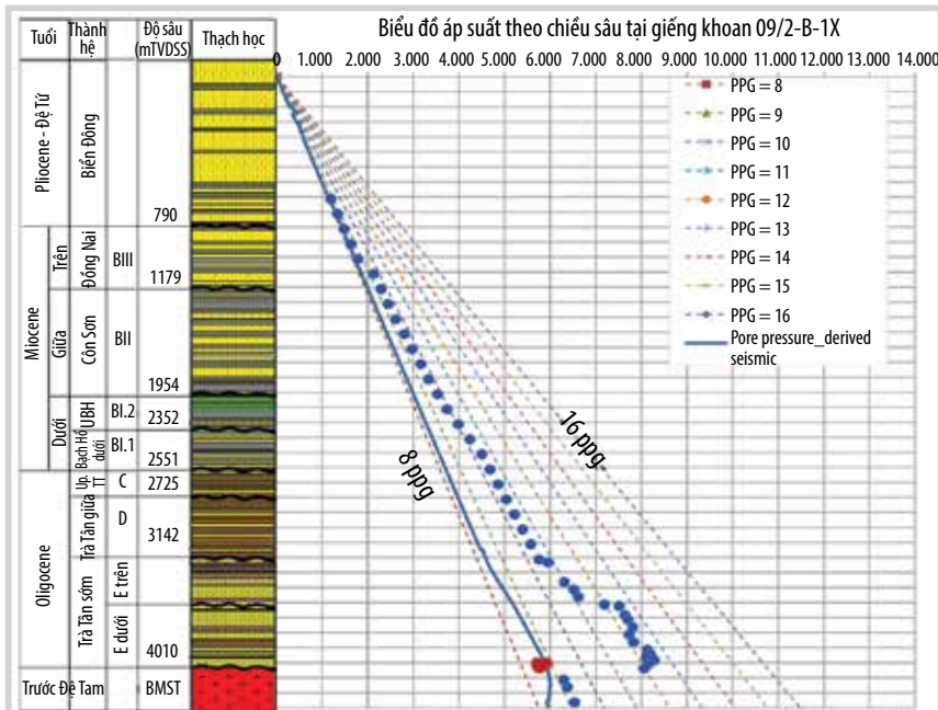
Hình 11. Biểu đồ áp suất và cột thạch học tại giếng khoan Lô 09/2, bể Cửu Long.
