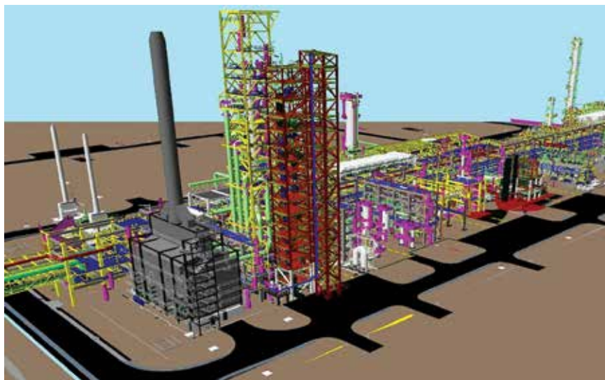
Hình 1. Mô hình 3D Cụm phân xưởng naphtha của Nhà máy Lọc dầu Dung Quất
