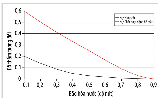
Hình 2. Độ thấm dầu tương đối của mẫu core Wolfcamp [3].
