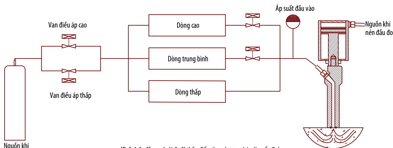
Hình 4. Sơ đồ nguyên lý đo độ thấm điểm theo phương pháp dòng ổn định.
