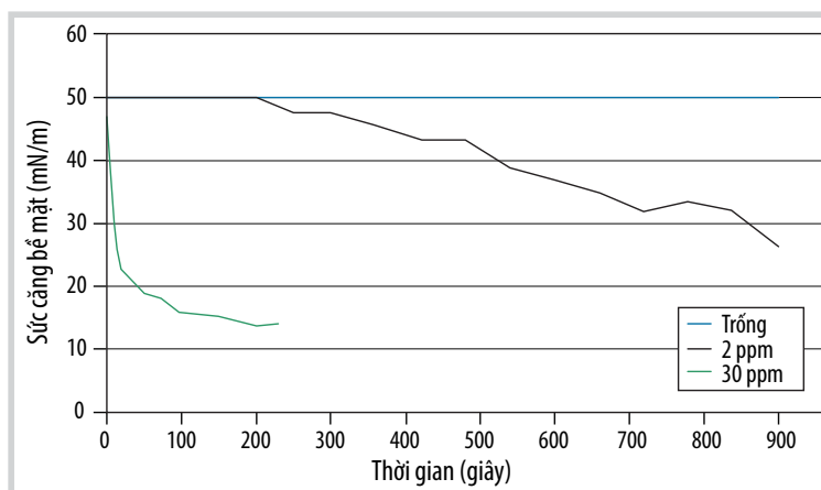
Hình 7. Độ nhay sức căng bề mặt của chất hoạt động bề mặt vi sinh [4].
