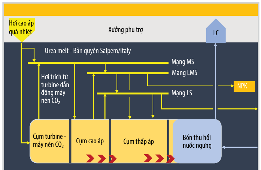
Hình 2. Mạng hơi-nước ngưng hơi xưởng urea Nhà máy Đạm Cà Mau.
