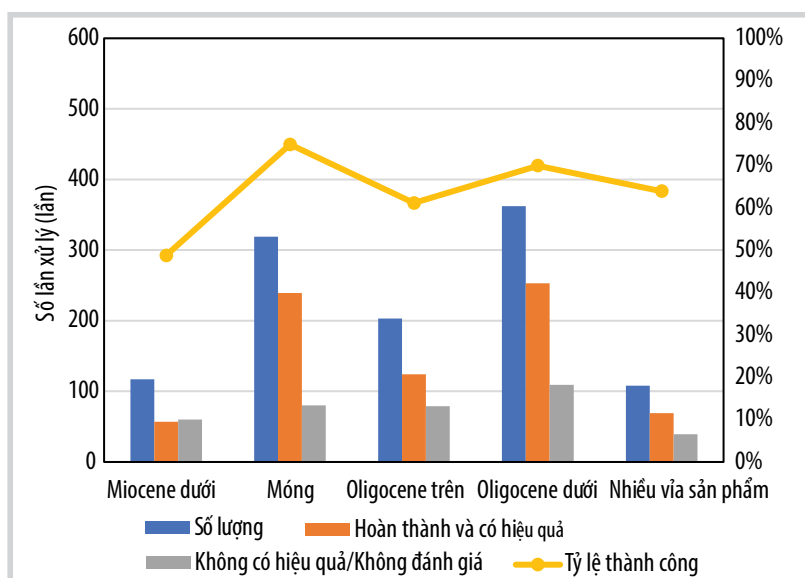
Hình 10. Đánh giá hiệu quả của phương pháp xử lý acid theo các đối tượng khai thác tại các mỏ bể Cù Long.
