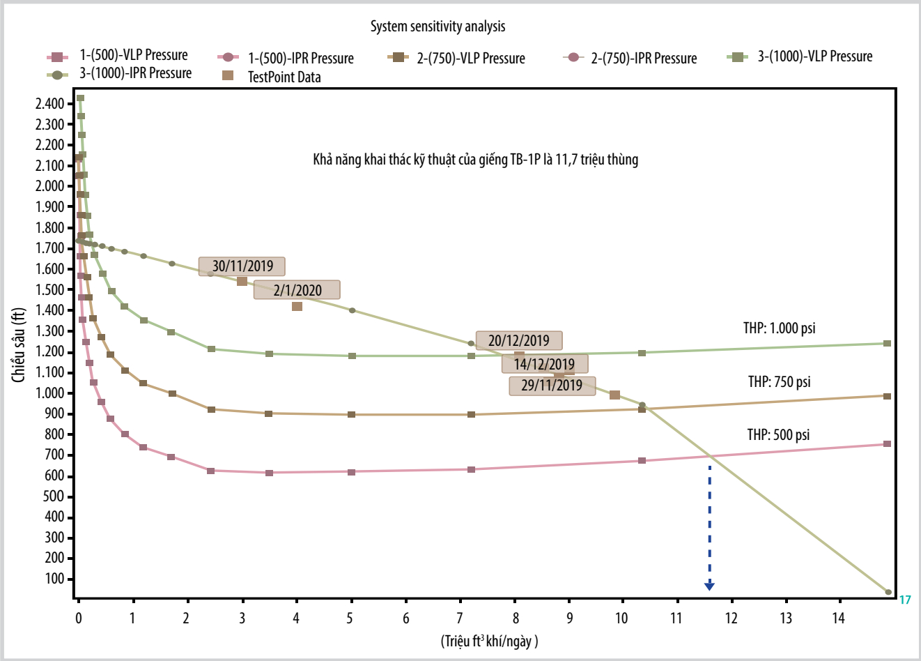
Hình 7. Khả năng khai thác của giếng TB-1P, mỏ Thái Bình sau khi xử lý.
