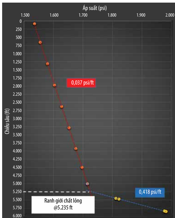
Hình 2. Kết quả phân tích gradient áp suất giếng TB-1P, mỏ Thái Bình.
