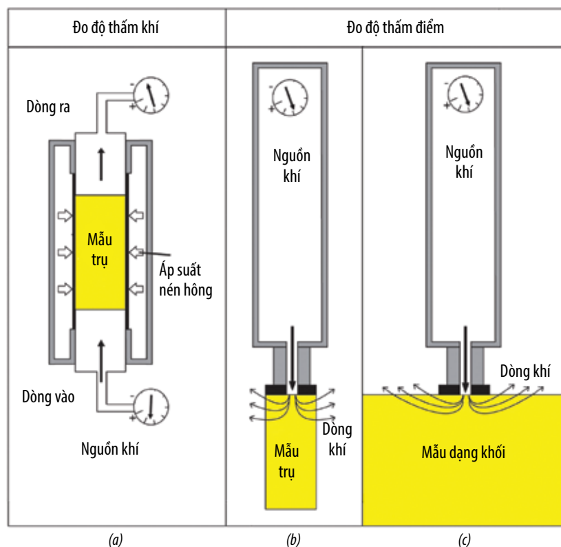
Hình 1. Mô hình dòng chảy qua mẫu khí đo độ thấm khí (a) và khí đo độ thấm điểm (b, c) [2].
