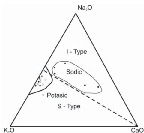
Hình 4. Biểu đồ \text{Na}_2\text{O} - \text{K}_2\text{O} - \text{CaO} (%wt) phân chia loại sodic, potasic (theo Poldervart, 1953) tương ứng với loạt sodic là trường granite kiểu I và với loạt potasic là trường granite kiểu S (theo A.J.White và B.W.Chappell, 1974); ký hiệu như Hình 1
