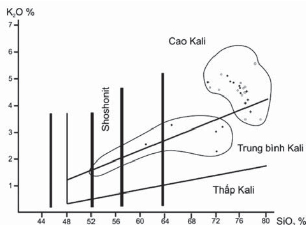
Hình 3. Biểu đồ phân chia các đá bazan (với SiO_2 > 48\% ), andesitobazan, andesit, dacit và ryolit theo các kiểu thấp kali, trung bình kali và cao kali (theo Peccerillo và Taylor, 1976); ký hiệu như Hình 1
