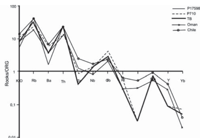
Hình 8. Biểu đồ phân bố các nguyên tố không tương hợp chuẩn hóa với granite sống núi đại dương (ORG) cho các đá phun trào hệ tầng Nha Trang - phụ hệ tầng dưới ( \text{Knt}_1 ). Giá trị granite cung núi lửa kiểu Chi Lê và granite đồng va chạm kiểu Oman (theo Pearce, 1984)
