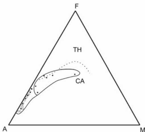
Hình 5. Biểu đồ AMF phân chia loạt tholeiit (TH) và loạt kiềm - vôi (CA) (Theo Irvine và Baragar, 1968) A = \text{Na}_2\text{O} + \text{K}_2\text{O} ; F = \text{FeO}^* ; M = MgO; Ký hiệu như Hình 1
