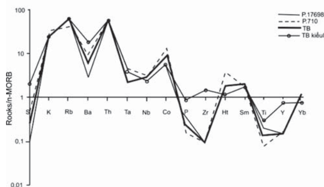
Hình 7. Biểu đồ phân bố các nguyên tố không tương hợp chuẩn hóa với N-MORB của các đá phun trào hệ tầng Nha Trang - phụ hệ tầng dưới ( \text{Knt}_1 ) (theo Condie, 1989). Giá trị N-MORB (theo Wood, 1979); giá trị trung bình kiểu I (theo Whalen, 1987)
