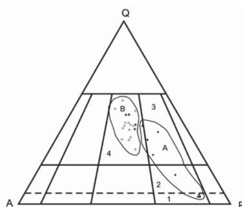
Hình 1. Biểu đồ QAP (phân loại - gọi tên đá) theo thành phần khoáng vật modal (theo Streckeisen, 1976); 1: Trường các đá monzodiorit; 2: Trường các đá monzodiorit thạch anh, monzogabro thạch anh bazan và andesit; 3: Trường các đá granodiorit; 4: Trường các đá granite và ryolit; \Delta : Hệ tầng Nha Trang; ( \bullet ): Phụ hệ tầng dưới; ( \circ ): Phụ hệ tầng trên; (+): Phụ hệ tầng Đèo Cả
