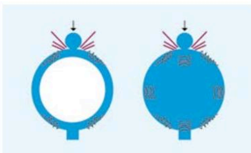
Hình vẽ mô tả cách thức truyền của sóng âm. Hình trái: Sóng âm truyền trong một kết cấu rỗng. Hình phải: Sóng âm truyền trong khối đặc.
