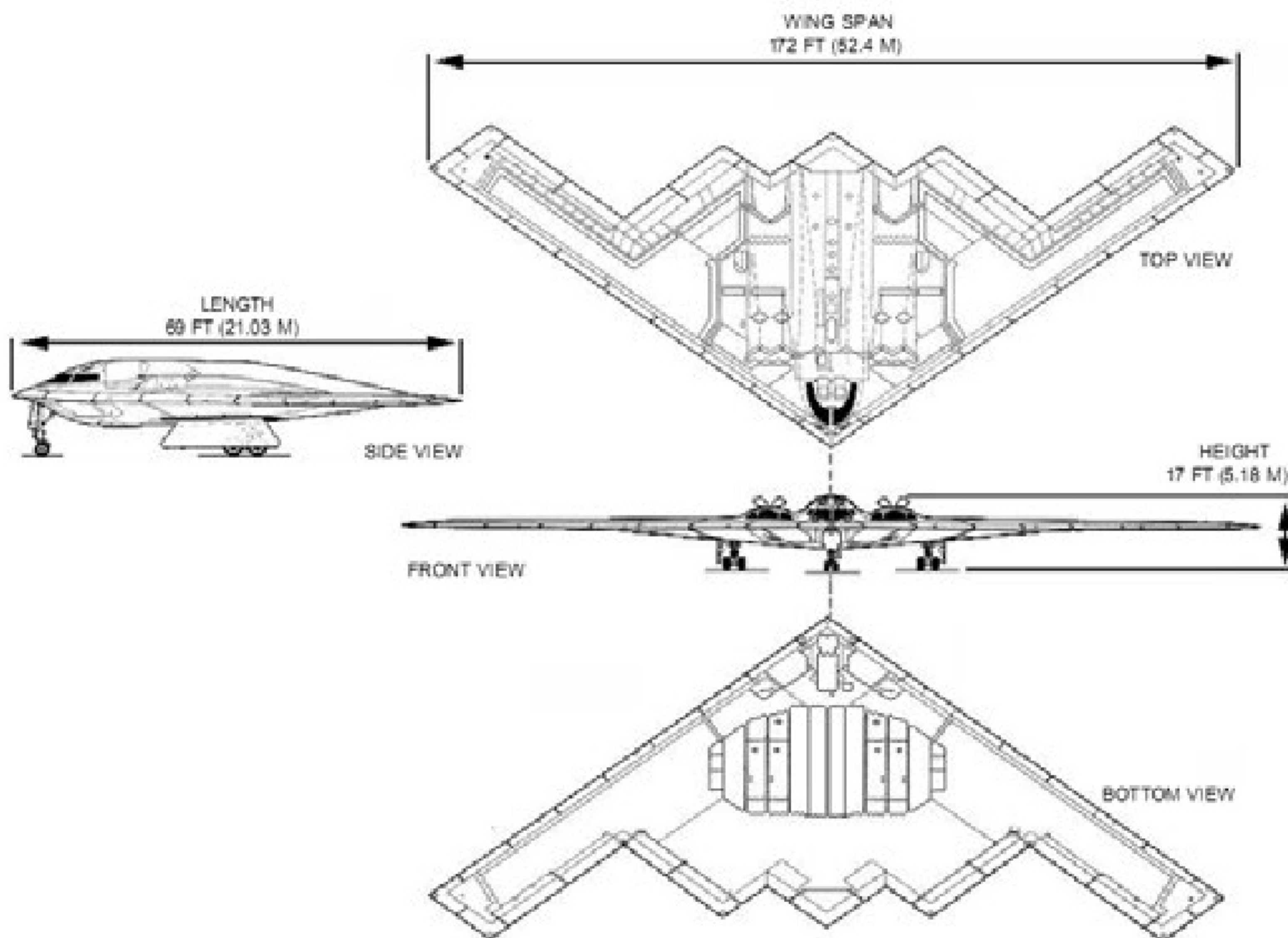
Hình chi tiết kỹ thuật Northrop B-2 Spirit.
