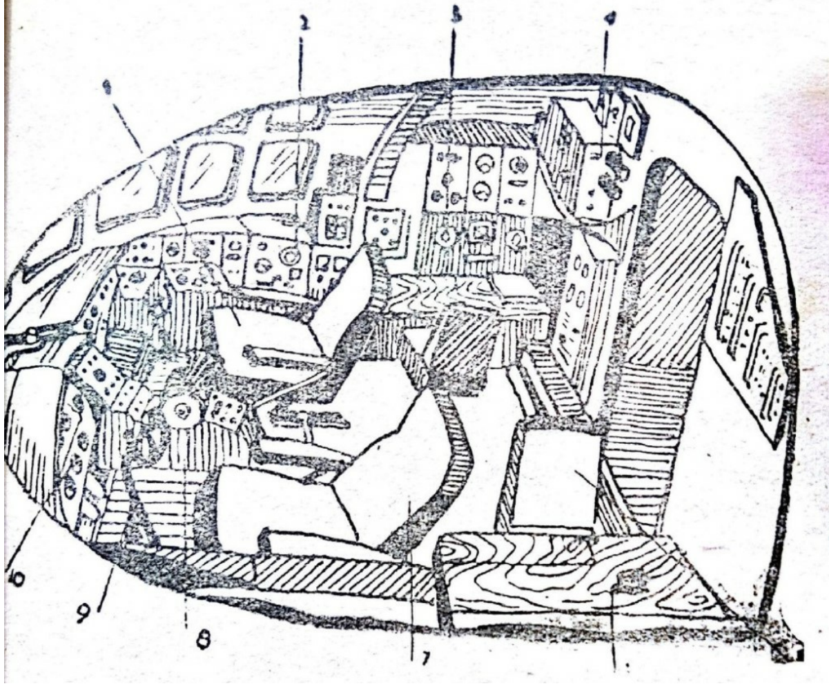
Buồng lái máy bay hành khách : 1 - ghế người lái phải. 2 - bảng điều khiển phải. 3 - nơi làm việc của hoa tiêu. 5. 6 - nơi làm việc của nhân viên vô tuyến. 7 - ghế người lái trái. 8 - bảng điều khiển giữa. 9 - cần lái trái. 10 - bảng điều khiển trái.
