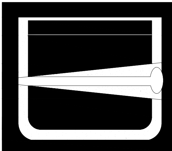
Hình 8.7 : Hiệu ứng Tindan
