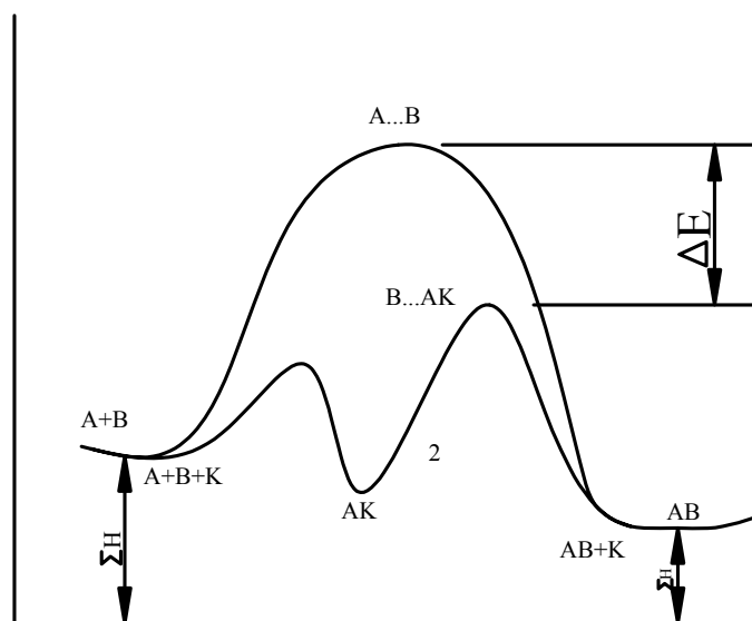
Hình 6.2. Biểu đồ năng lượng của phản ứng có xúc tác dương
