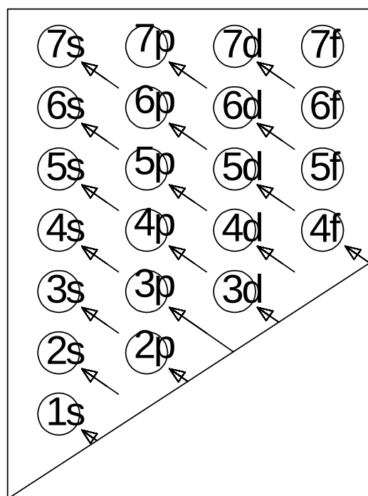
Hình 2.4. Quy tắc sắp xếp năng lượng Klexcopxki
