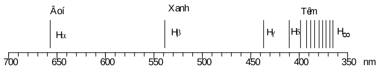
Hình 2.2 Phổ của nguyên tử hydro
