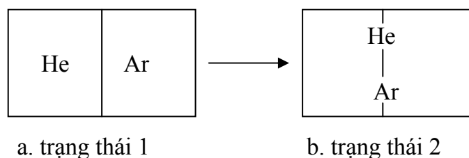
Hình 5.5. Sự tự trộn lẫn của chất khí
