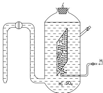
Hình 9.3 : Điện cực Hydro
