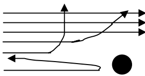
Hình 2.1. Sự tán xạ của tia \alpha
