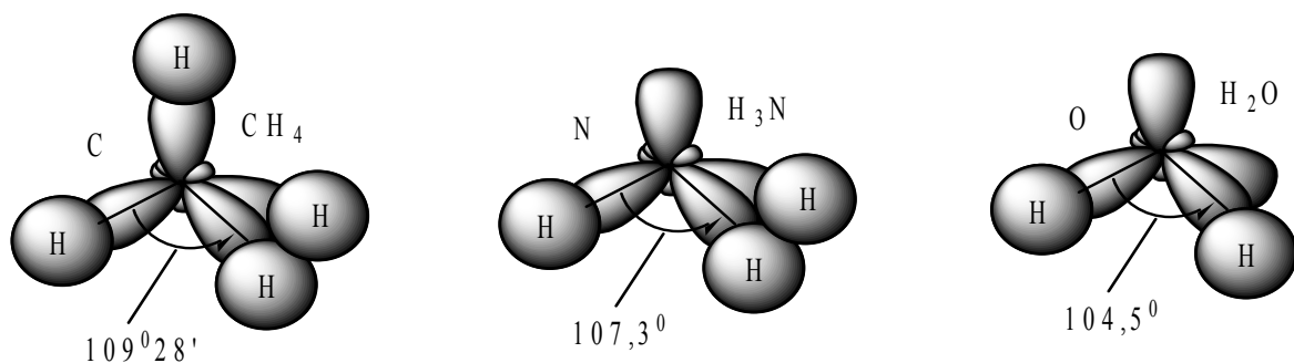
Hình 4.6 Sự xen phủ orbital trong phân tử \text{CH}_4 , \text{NH}_3 , \text{H}_2\text{O}
