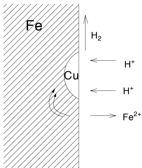
Hình 9.8 : Sơ đồ hoạt động cặp nguyên tố gavanhi
