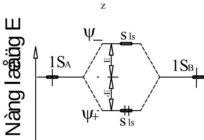
Hình 4.12. Giản đồ năng lượng của nguyên tử và phân tử hydro
