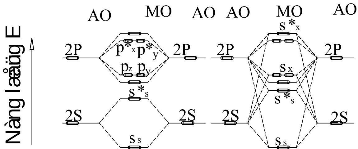
Hình 4.13. Biểu đồ năng lượng nguyên tử và phân tử của các nguyên tố chu kỳ 2
