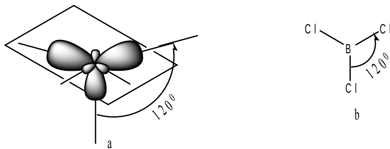
Hình 4.7. Phân tử \text{BCl}_3
