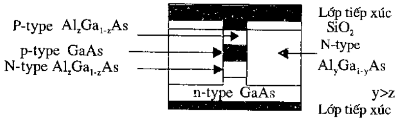
Hình 3.18. Mặt cắt ngang của diode Laser kiểu dị thể chôn.
