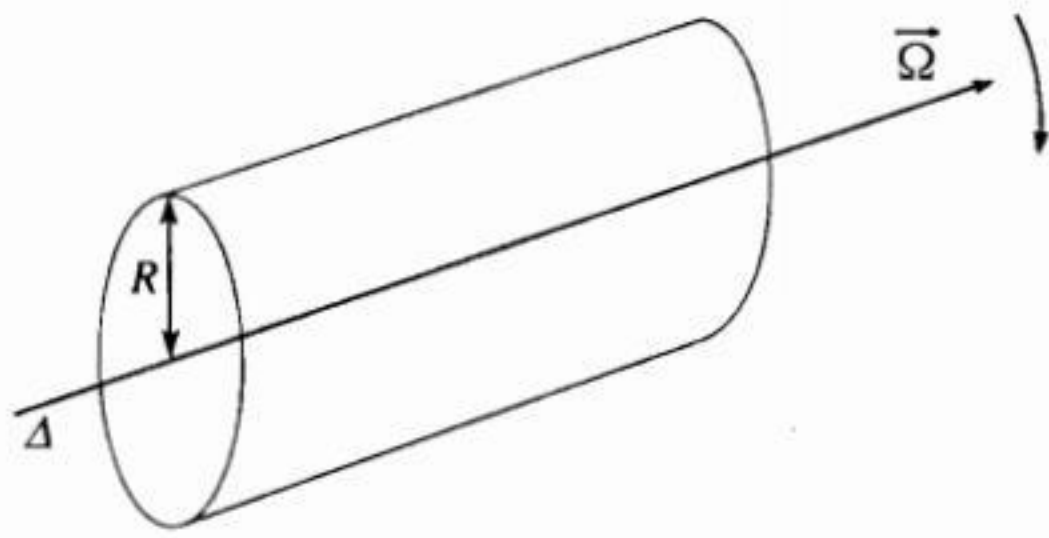
H.26. Momen động lượng của hình trụ đồng nhất là đồng tuyến với \vec{\Omega} .
