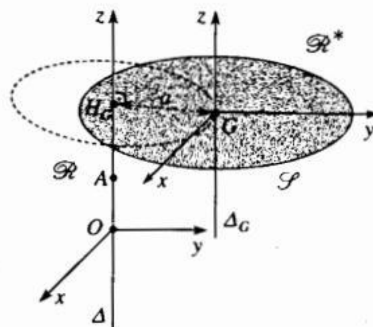
H.29. Định lý HUYGENS.
