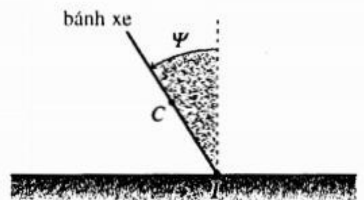
H.16. Nhìn từ đằng sau bánh xe.
