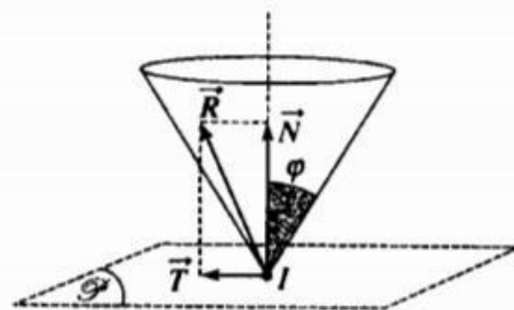
H.11. Hình nón ma sát.
