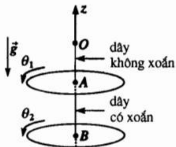
H.10. Hai đĩa nối với nhau bằng một dây xoắn.
