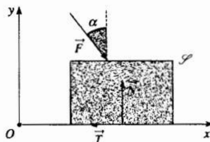
H.16. Hiệu ứng kẹt.
