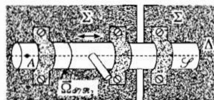
H.5. Thí dụ về liên kết trụ quay trượt.
