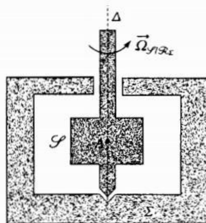
H.3. Các thí dụ về liên kết trụ quay.
