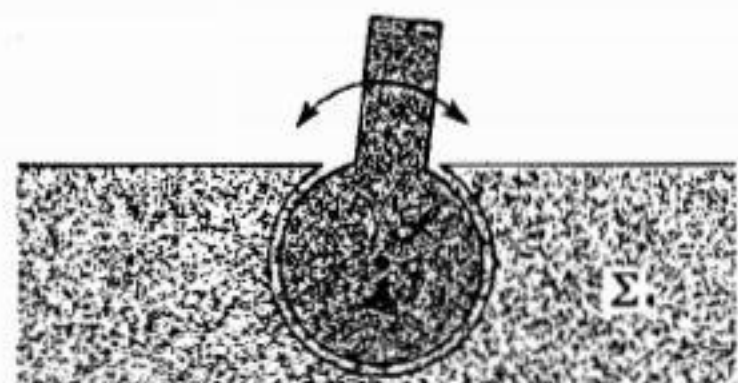
H.2. Thí dụ về liên kết khớp cầu : A là tâm của hình cầu chung ở \mathcal{S} và ở \Sigma
