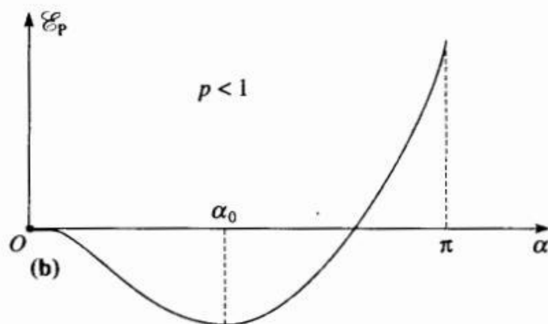
b. Đối với p < 1 , \alpha_e = 0 là một vị trí cân bằng không bền và \alpha_e = \alpha_0 là một vị trí cân bằng bền.
