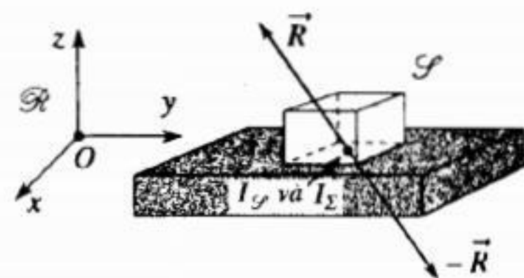
H.19. Hình lập phương \mathcal{P} tịnh tiến trên bề mặt \Sigma
