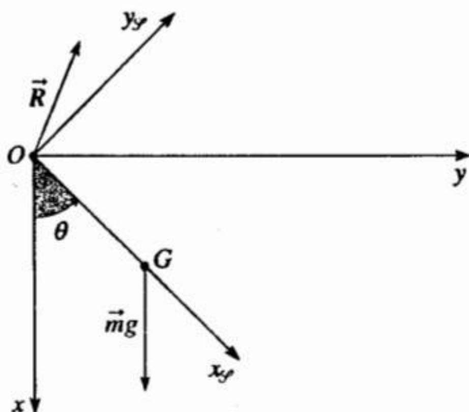
H.11. Phân lực \vec{R} lên con lắc.
