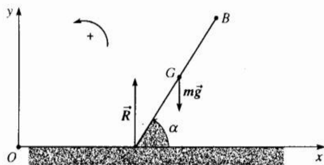
H.4. Các lực tác dụng lên thanh.
