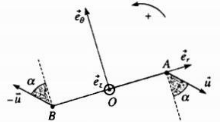
H.23 b. Sơ đồ hóa thiết bị nhìn từ trên xuống.
