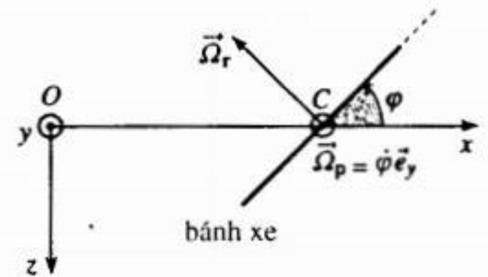
H.15. Bánh xe nhìn từ trên xuống.
