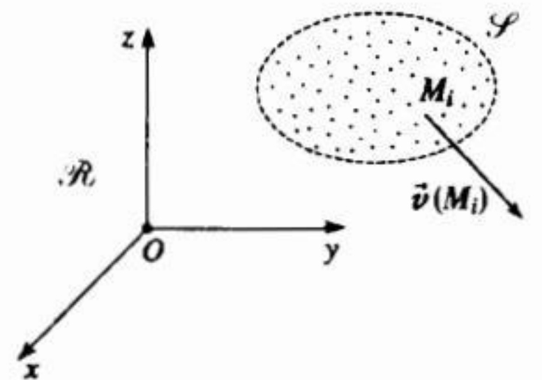
H.6. Hệ \mathcal{S} của các chất điểm.
