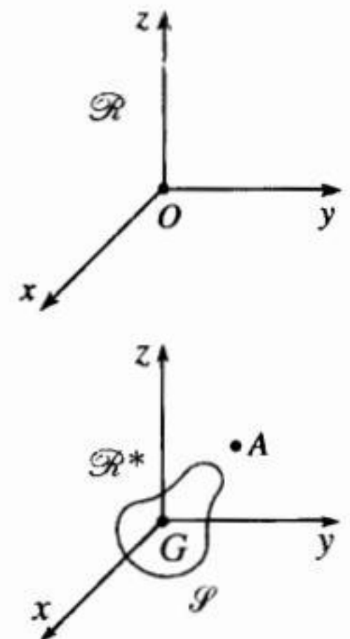
H.13. Hệ quy chiếu trọng tâm.
