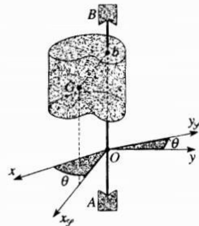
H.6. \mathcal{P} quay quanh trục (Oz) .
