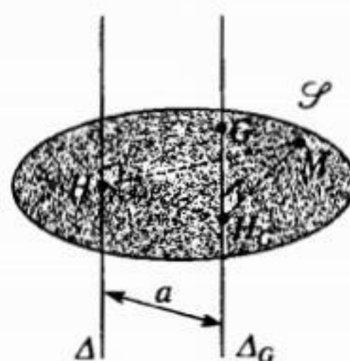
H.30. Quan hệ giữa J_A và J_{AG} .
