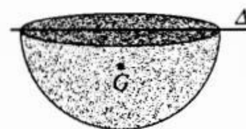
H.22. Momen quán tính của một bán cầu.
