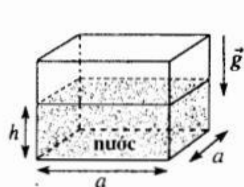
H.5. Lực nén lên thành bình.
