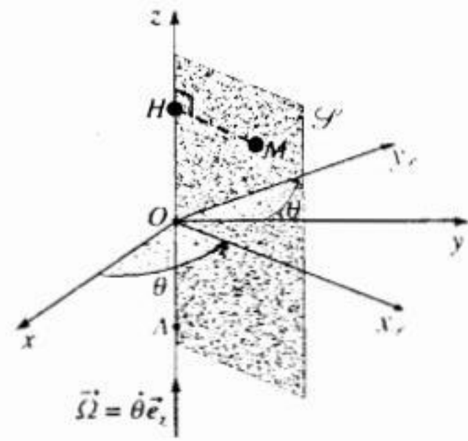
H.17. Cánh cửa quay quanh bản lề.
