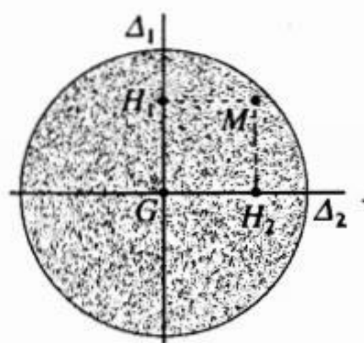
H.21. Momen quán tính của một đĩa.
