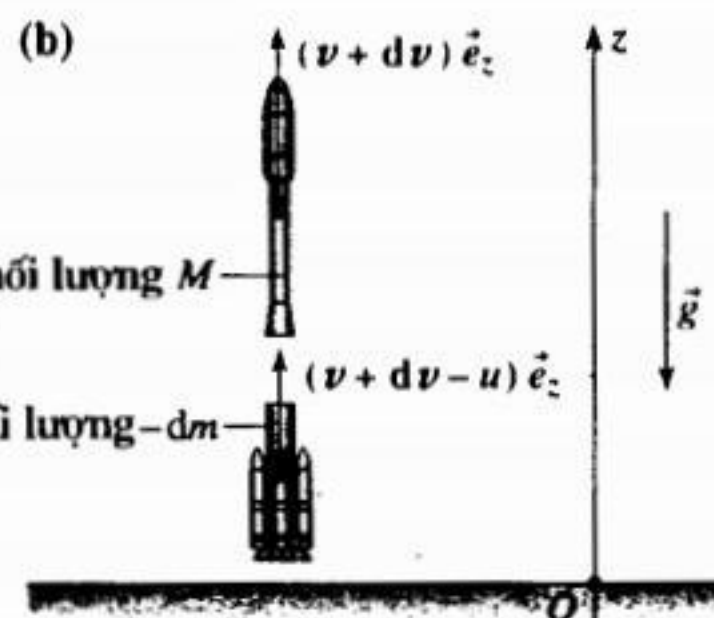
H.22. Hệ có khối lượng tổng cộng M = M_0 + m trải qua hai thời điểm t và t + dt (chú ý là dm < 0 ).
