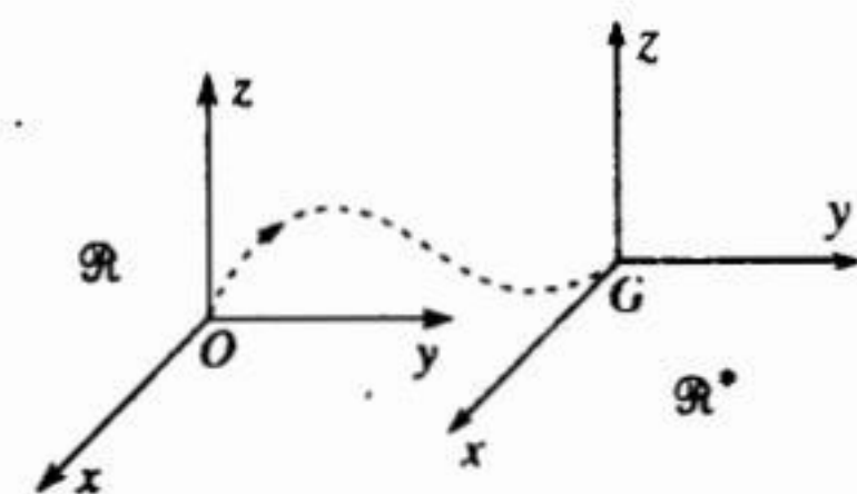
H.11. Hệ quy chiếu trọng tâm \mathcal{R}^* là tịnh tiến đối với hệ quy chiếu nghiên cứu \mathcal{R} .
