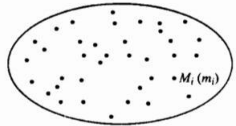
H.7. Hệ các chất điểm.
