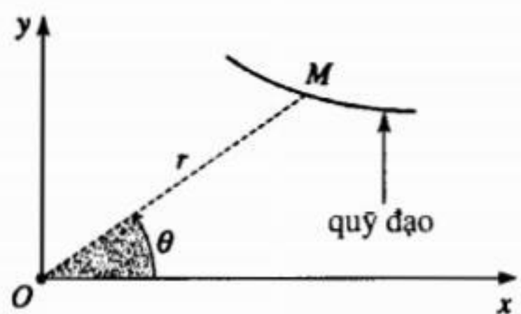
H.12. Hạt M trong trường các lực xuyên tâm.
