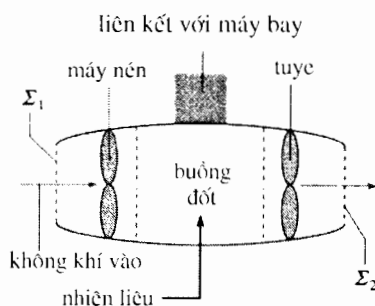
H.11. Tuabin phản lực.
