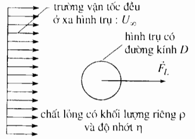
H.76. Lực F_L tác dụng lên một đơn vị dài của hình trụ là hàm của U_\infty (vận tốc đều của chất lỏng ở vô cùng), \rho khối lượng riêng của chất lỏng), \eta (độ nhớt của chất lỏng) và D (đường kính của trụ tròn).
