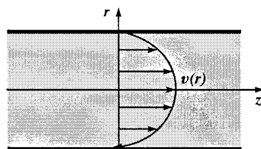
H.29. Phân bố parabol của vận tốc trong một dòng chảy POISEUILLE. Hệ có tính đối xứng tròn xoay xung quanh trục ( Oz ).
