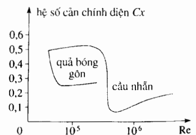
H.51. Sự khác nhau giữa các hệ số cản chính diện Cx(Re) của một quả bóng nhẵn và của một quả bóng gôn trong một chuyển động có số REYNOLDS lớn.
