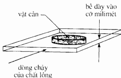
H.45. Ống HELE-SHAW được cấu tạo bởi hai tấm cách nhau khoảng 1 mm, giữa chúng có một chất lỏng dịch chuyển với vận tốc nhỏ, cỡ \text{mm.s}^{-1} .
