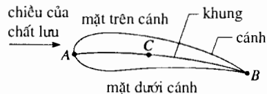
H.43. Ta nhận được sự mô phỏng bằng cách phân bố các nguồn từ A đến C và các giếng từ C đến B. Một dòng xoáy, áp đặt ở lân cận điểm A, là cần thiết để tạo ra một lực nâng.
