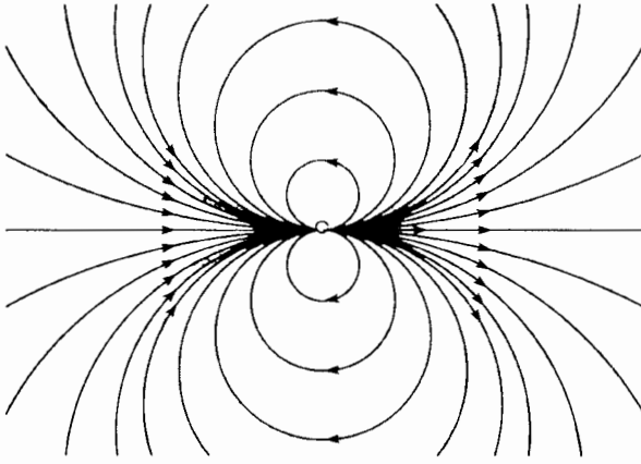
H.35. Trường các vận tốc liên quan đến dòng chảy của một lưỡng cực thủy động lực.
