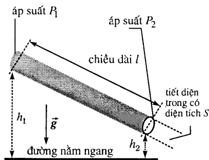
H.30. Lưu lượng thể tích của chất lỏng đang ở dòng chảy tầng trong ống tiết diện S và chiều dài l này có dạng:
