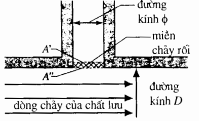
H.32. Nếu tiết diện ống (đường kính \phi ) nhỏ so với tiết diện của dòng chảy (đường kính D ), thì miền chảy rối sẽ có kích thước giảm nhỏ đi, và ta có P_{A'} = P_{A''} .
