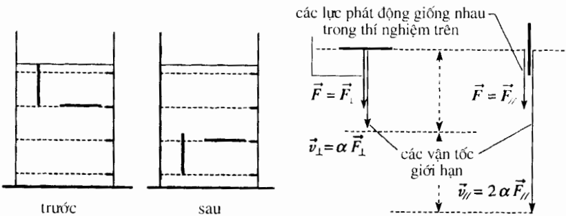
H.41. Ở số REYNOLDS rất nhỏ, vận tốc rơi giới hạn phụ thuộc vào hướng của nó. Các vận tốc này nằm trong tỉ lệ 2: v_{//} = 2v_{\perp} .
