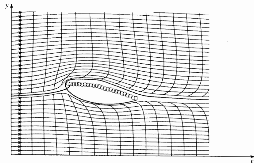
H.41. Sự thể hiện hình dạng cánh với cách mô phỏng này.
