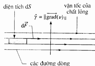
H.54. Độ nhớt \eta của một chất lỏng thực được xác định bởi hệ thức sau :
