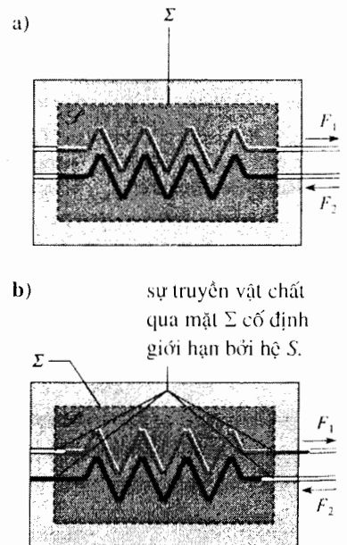
H.3. Hệ mở \mathcal{P} được giới hạn bởi mặt kiểm tra cố định \Sigma – vẽ chấm chấm. a. Hệ mở \mathcal{P} và hệ kín trùng với \mathcal{P}^* lúc t_0 . b. Lúc t_0 + dt , các hệ này không còn trùng với nhau nữa.
