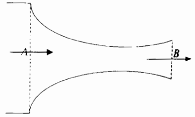
H.24. Ống tuye.
