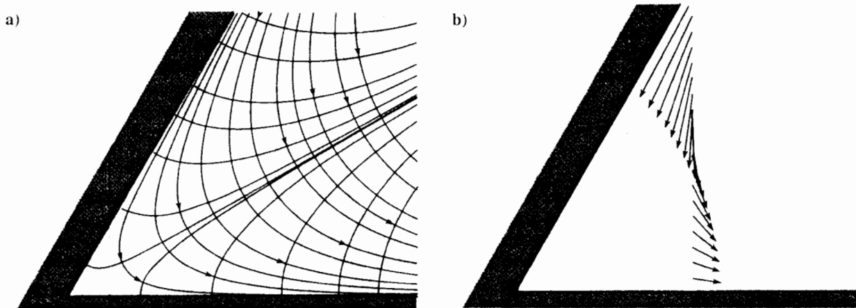
H.30. Dòng chảy thế trong một nhị diện góc \frac{\pi}{4} . a. Các đường dòng và các đường \phi = \text{cte} trực giao nhau. b. Các đường đi của vận tốc.
