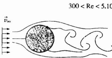
H.32. Sự tách ra của lớp giới hạn thành lớp được thực hiện ngày càng ra phía sau của hình trụ.
