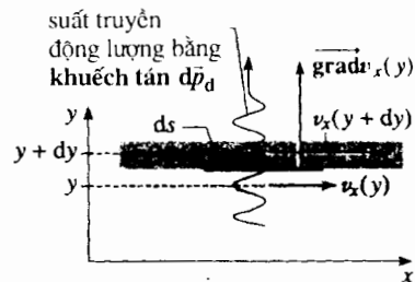
H.8b. Sự truyền động lượng bằng khuếch tán :
