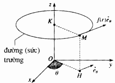
H.61a. Sự nghiên cứu một trường trục xuyên tâm dạng f(r)\vec{e}_\theta .
