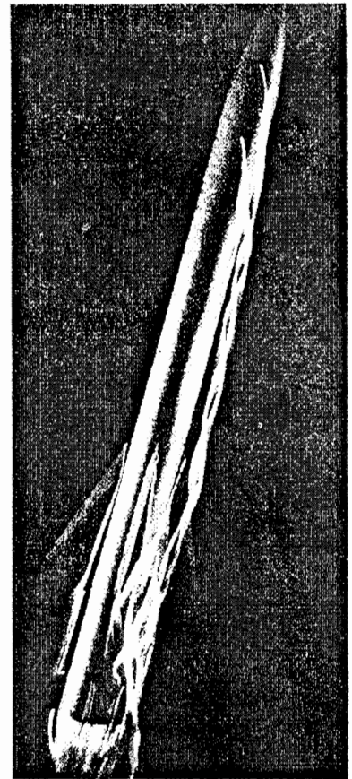
H.19. Sự thể hiện các đường phát xạ. Các chỗ nước xoáy trên một vật thể hình thoi đang đi với. Sự làm hiện rõ bằng các tia phát xạ nhuộm màu.
