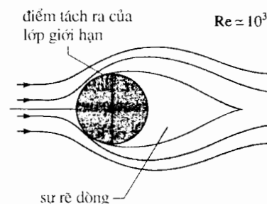
H.26. Dòng chảy không còn đều đặn nữa. Lớp giới hạn là thành lớp, nhưng một miền rối được phát triển ở phía sau quả cầu. Điểm cắt trượt của lớp giới hạn nằm ở "phía trước".
