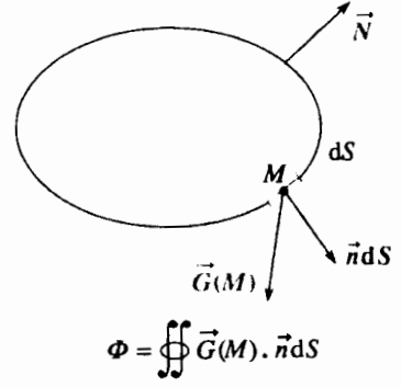
H.22. Định nghĩa thông lượng của một vector.
