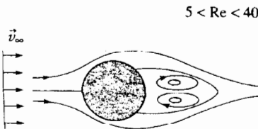
H.30. Các cuộn xoáy bên xuất hiện ở phần sau trụ. Dòng chảy có dạng hình trụ.
