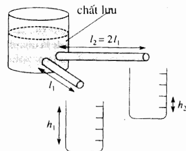
H.31. Đối với hai dòng chảy POISEUILLE này, nếu l_2 = 2l_1 thì lúc đó h_2 = \frac{h_1}{2} .
