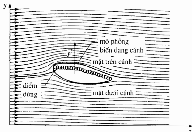
H.41. Sự thể hiện hình dạng cánh với cách mô phỏng này.
