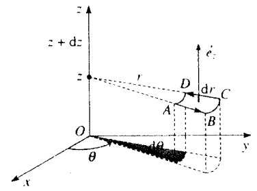
H.63. Sự lựa chọn diện tích nguyên tố để có thể tính thành phần của \text{rot} \vec{G} hướng theo (Oz) trong tọa độ trụ.
