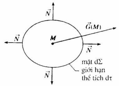
H.34. Thông lượng đi ra d\Phi của \vec{G} , qua diện tích nguyên tố d\Sigma giới hạn thể tích d\tau tâm M , thì bằng: d\Phi = \text{div} \vec{G} d\tau .
