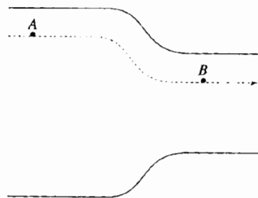
H.26a. Ống dẫn có một chỗ hẹp lại : chất lỏng ở chế độ ổn định được tăng tốc.
