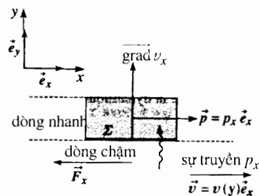
H.13. Động lượng dp_x đi qua mặt \Sigma trong thời gian dt được biểu thị theo F_x bởi:
