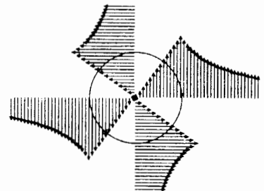
H.22. Sự thể hiện trường các vận tốc của một cơn lốc.
