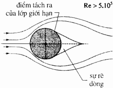
H.27. Lớp giới hạn thành lớp trước đây trở thành rối : nó được tháo ra ở "phía sau" quá cầu.
