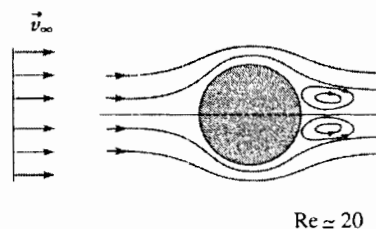
H.23. Cuộn xoáy xuất hiện ở phía sau quả cầu là hình xuyên.
