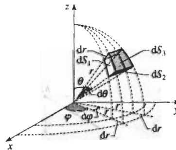
H.9. Các diện tích nguyên tố (và thể tích nguyên tố) trong tọa độ cầu:
