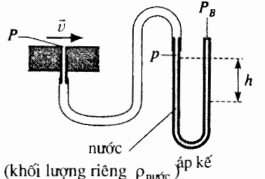
H.33. Áp suất là liên tục ở ngang mức lỗ hở, và P = P_B - \rho_{\text{nước}} g h .
