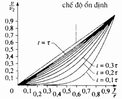
H.24. Sự biến đổi của vận tốc rút gọn \left(\frac{v}{v_2}\right) theo chiều dài rút gọn \left(\frac{y}{e}\right) ở các thời điểm khác nhau: 0, 0,1 \tau; 0,2 \tau; 0,3 \tau; \dots; 0,9 \tau; \tau .
