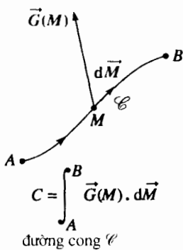
H.21. Định nghĩa lưu thông của một vector.
