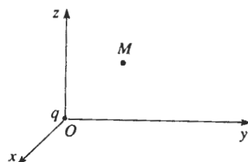
H.41. Cho một điện tích "điểm" trong không gian
