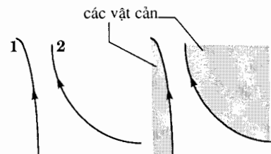
H.12. Sự cụ thể hóa các đường dòng.
