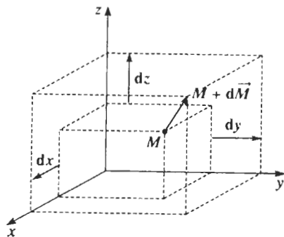
H.2. Vector d\vec{M} có các thành phần dx , dy , dz , nghĩa là:
