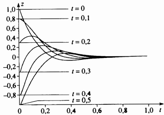
H.19. Màng dao động nằm ngang trong một chất lưu nhớt.
