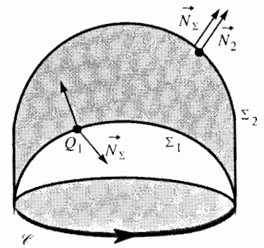
H.56. Cho dù các mặt \Sigma_1 và \Sigma_2 giới hạn một thể tích V như thế nào, thì ta vẫn có:
