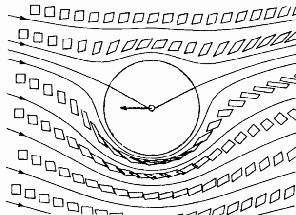
H.8. Dòng chảy của một chất lỏng xung quanh một hình trụ đang quay: Ta làm thấy rõ các biến dạng của các phần tử khác nhau.
