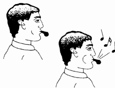
H.5. Phải có một lưu lượng tối thiểu để cuộn xoáy xuất hiện và một âm được phát ra.
