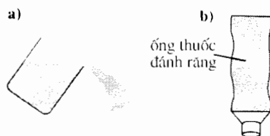
H.1. Dầu và thuốc đánh răng nhão là hai chất lưu "khác nhau". a. Dầu (hay nước) chảy ra khỏi cốc. b. Mặc dù lộn ngược, (bột nhão) thuốc đánh răng vẫn không trút ra khỏi ống.
