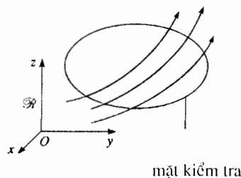
H.2a. Chất lỏng đi qua mặt kiểm tra cố định trong hệ quy chiếu nghiên cứu.
