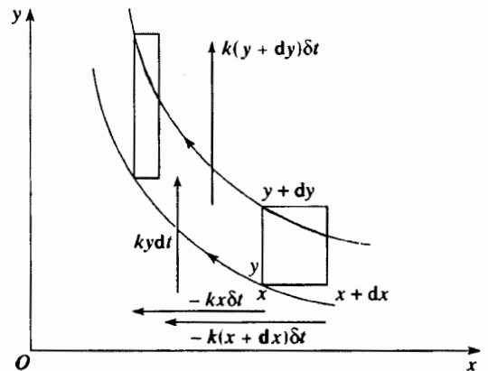
H.5. Sự biến dạng của một phần tử chất lỏng trong một dòng chảy hai chiều (nhị diện vuông).
