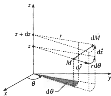
H.5. Trong tọa độ trụ:
