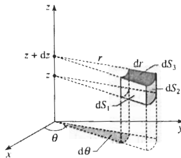
H.6. Sự thể hiện các diện tích (và thể tích) nguyên tố trong trường hợp các tọa độ trụ:
