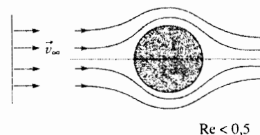
H.22. Với một số REYNOLDS nhỏ, dòng chảy là thành lớp và gần như tuyến tính.
