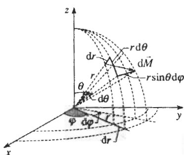
H.8. Tọa độ cầu:
