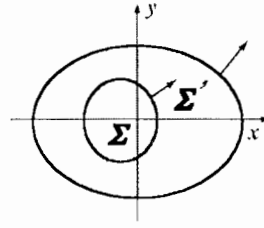
H.13a. Các lưu lượng khối (đi ra) qua các mặt \Sigma và \Sigma' đều như nhau (tồn tại một nguồn ở 0)
