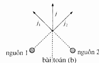
H.45. Tính tương đương giữa các bài toán (a) và (b) trong nửa không gian 1.
