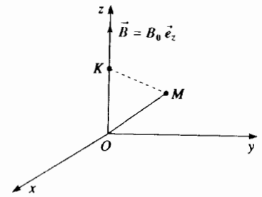
H33. Các mặt phẳng sao cho \vec{B} \cdot \vec{OM} không đổi, là các mặt phẳng trực giao với (Oz) . Vậy \text{grad}(\vec{B} \cdot \vec{OM}) được mang bởi \vec{B} .
