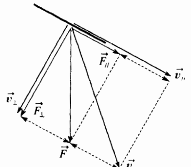
H.43. Lực ("phát động") \vec{F} có thể được phân tích thành hai lực \vec{F}_{//} và \vec{F}_{\perp} :
