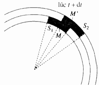
H.7c. Có sự trượt của S_2 đối với S_1 , vậy có sự dịch chuyển tương đối của S_2 đối với S_1 ; nên tồn tại các lực nhớt.
