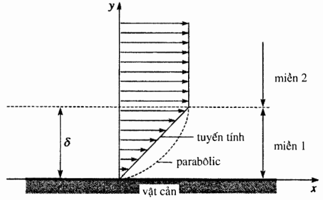
H.18. Vận tốc của chất lỏng trong miền 1 có thể mô hình hóa bằng một prôfin tuyến tính (vector cuộn xoáy \Omega đều) hay một prôfin parabolíc (vector \Omega thay đổi tuyến tính theo y ) hoặc theo hàm mũ.
