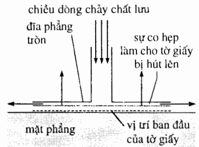
H.24. Tờ giấy tự nâng lên.
