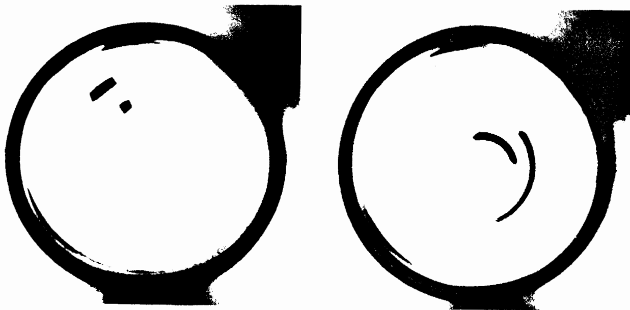
H.3. Đo vận tốc. Bình chứa có đường kính d = 9,5 cm và chiều cao h = 14 cm. Vận tốc quay của nó là \omega_0 = 45 vòng.phút -1 . Hai bức ảnh được chụp lần lượt lúc 30 giây và 150 giây sau khi bắt đầu quay. Thời gian lộ sáng là \frac{1}{2} s. Một chỉ tiết gắn với bình chứa vẽ một cung tròn có độ mở 135^\circ .
