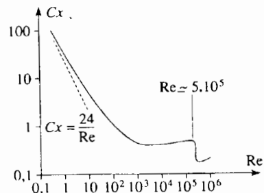
H.21. Hệ số cản chính diện C_x(Re) đối với một quả cầu nhẵn.
