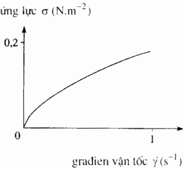
H.59. Sự biến thiên của ứng lực \sigma theo gradient vận tốc \dot{\gamma} đối với việc sơn bóng mịn, lúc dòng chảy có gradient vận tốc thấp.
