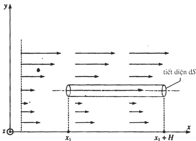
H.39. Trường các vector dạng v_x(y)\vec{e}_x có div triệt tiêu, nhưng rota không triệt tiêu.
