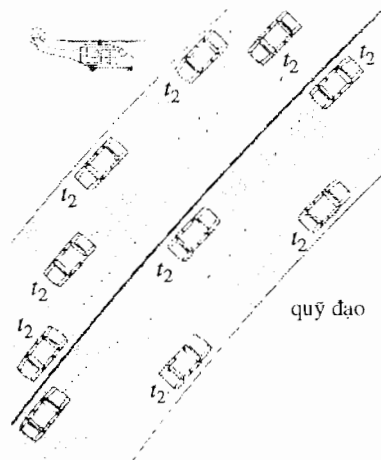
H.9. Khi ta quan sát các quỹ đạo của các xe cộ khác nhau (giữa t = t_1 và t = t_2 ), thì ta đứng trên hình thức luận của Lagrange.
