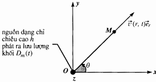
H.14. Một nguồn dạng chỉ chiều cao h trùng với trục ( Oz ) phát ra một chất lỏng với lưu lượng khối D_m(t) .
