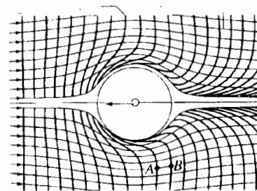
H.17c. Minh họa sự biến dạng của một "đường chất lỏng". Khoảng thời gian mà một hạt chất lỏng cần để đi từ A đến B là một bất biến trên hình này.
