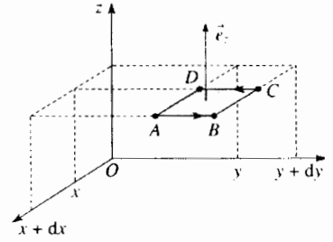
H.62. Sự lựa chọn diện tích để có thể tính toán thành phần của \vec{\text{rot}} \vec{G} hướng theo trục (Oz) .
