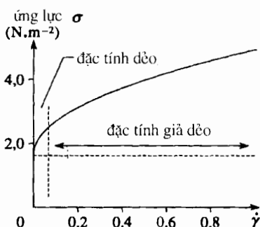
H.65. Ứng suất \sigma biến thiên theo gradient vận tốc \dot{\gamma} đối với việc trát hơi dày, khi một dòng chảy có gradient vận tốc hạ thấp, không thể mô hình hóa được bởi định luật OSTWALD:
