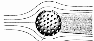
H.49. Xung quanh một quả bóng gôn có một lớp giới hạn rối.
