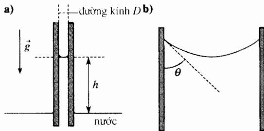
H.8a. Chất lỏng dâng lên trong một ống đường kính D nhỏ so với D_c . b. \theta là góc nổi bề mặt của chất lỏng với thành ống.
