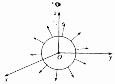
H.47. Sự vẽ topo của trường \frac{\vec{e}_r}{r^2} trong tọa độ cầu. \operatorname{Div} của vector này triệt tiêu \left(\operatorname{div}\frac{\vec{e}_r}{r^2} = 0\right) , mặc dù thông lượng đi ra qua một mặt cầu bán kính r lại khác không và bằng 4\pi .
