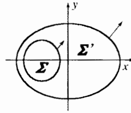
H.13b. Lưu lượng khối (đi ra) qua mặt \Sigma bằng không, trong khi lưu lượng khối qua mặt \Sigma' lại bằng lưu lượng khối của nguồn ở tại 0.
