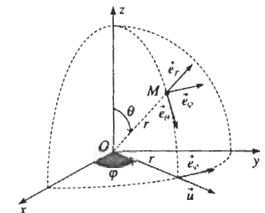
H.7a. Trường hợp các tọa độ cầu.
