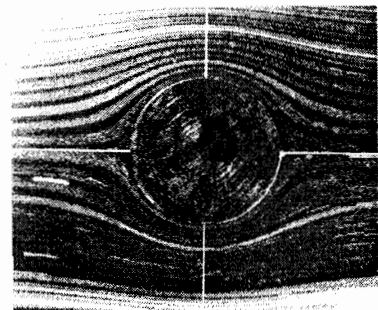
H.17b. Dòng chảy xung quanh một hình trụ chiều dày nhỏ và ở vận tốc nhỏ. Sự thể hiện rõ dòng chảy nhờ các tia dầu lạnh trong dầu vazolin.
