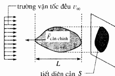
H.10. Hệ số cản chính C_x là một số không thứ nguyên xác định bởi :
