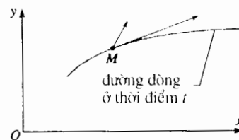
H.17. Phần tử chiều dài d\vec{l} (ở M) được chọn tùy ý.
