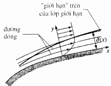
H.14. Một lớp giới hạn không nhất thiết là không đối.
