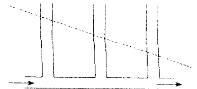
H.25. Sự tổn hao áp suất trong một dòng chảy của chất lỏng thực không chịu nén trong một ống có tiết diện không đổi.
