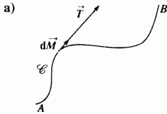
H.14a. Đường cong \mathcal{C} được định hướng từ A đến B .
