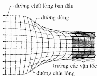
H.26b. Sự biến đổi các đường chất lỏng của một chất nước khi có chỗ hẹp lại.
