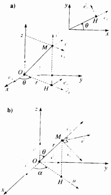
H.25. Các hệ trục được sử dụng.
