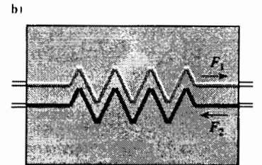
H.5. Biến đổi của hệ kín \mathcal{H}^* ;
