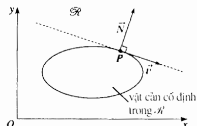
H.16. Trong một hệ quy chiếu \mathcal{R} , vận tốc của một chất lỏng nhất thiết phải tiếp tuyến với một vật cản cố định trong hệ quy chiếu này.
