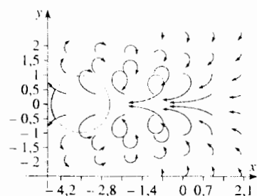
H.15. Sự thể hiện rõ các quỹ đạo của các hạt chất lỏng khi có sự dịch chuyển của một hình trụ: "xa" hình trụ này, chất lỏng đứng im.
