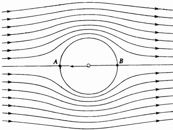
H.42. Dòng chảy thể xung quanh một hình trụ. Các điểm A và B là các điểm vận tốc triệt tiêu.
