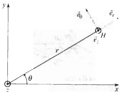
H.4c. Trong mặt phẳng (xOy) , ta lại tìm thấy hệ tọa độ cực.
