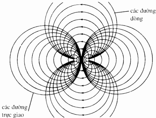
H.38. Các đường dòng liên quan đến sự chống chập của một giếng và một nguồn (lưu lượng bằng nhau về môđun) là những vòng tròn.
