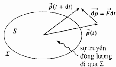
H.12. Động lượng d\vec{p} đi qua mặt kín \Sigma trong thời gian dt được biểu thị theo D_p = \vec{F} bởi:
