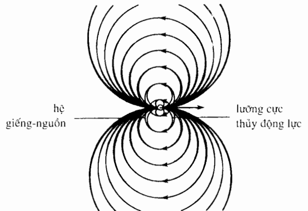
H.39. Các đường dòng của lưỡng cực thủy động lực và các đường dòng của một hệ giếng – nguồn khác nhau rất ít.
