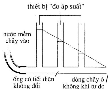
H.28. Các mức cực đại trong các ống thẳng đứng khác nhau đều sắp thẳng hàng.
