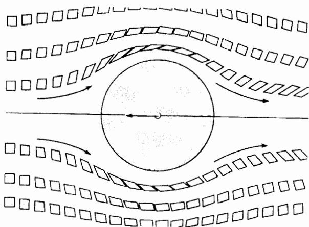
H.1b. Sự mô phỏng số học dòng chảy này cho thấy rõ sự vận động của một thể tích nguyên tố.
