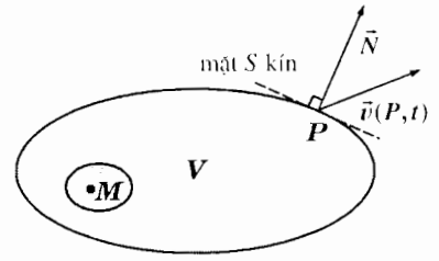
H.10. Sự cân bằng khối lượng kết hợp với một thể tích kiểm tra V cố định.
