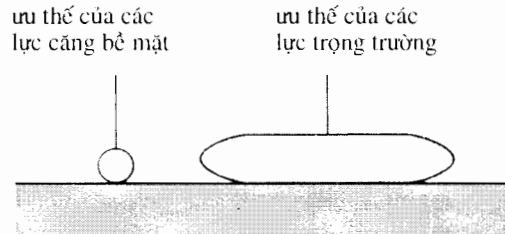
H.9. Giọt thủy ngân trên mặt đất nằm ngang.
