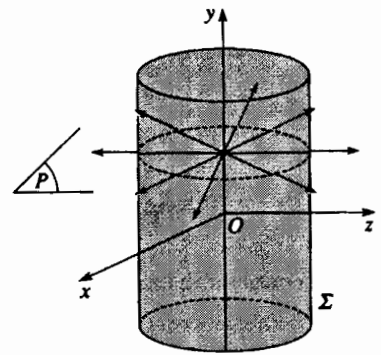
H.45. Sự vẽ topo của trường \frac{\vec{e}_r}{r} trong tọa độ trụ. Đi về của vector này triệt tiêu \left(\text{div}\frac{\vec{e}_r}{r} = 0\right) mặc dù thông lượng đi ra qua một hình trụ bán kính r và chiều cao h lại khác không và bằng 2\pi h !
