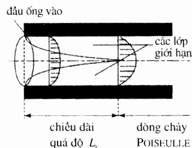
H.32. Ở đầu ống, tồn tại một chiều dài quá độ mà trên đó dòng chảy tiến đến trở thành một dòng chảy POISEUILLE.
