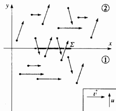
H.17a. Lưu lượng phân tử D_{N_{1 \rightarrow 2}} đi qua mặt \Sigma tương ứng với các hạt mà vận tốc \vec{u} song song với y và cùng chiều.
