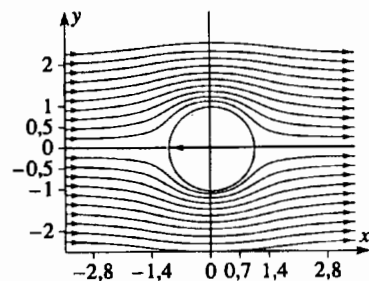
H.17a. Sự mô phỏng cho thấy dòng chảy của một chất lỏng xung quanh một hình trụ.
