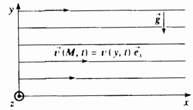
H.18. Dòng chảy của một chất lưu nhớt không thể nén được, do vậy các đường dòng song song với (Ox).
