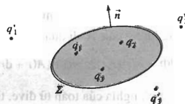
H.42. Gọi \vec{E} là trường tĩnh điện tổng cộng được tạo ra bởi các điện tích ở trong ( q_i ) và ở ngoài ( q_i' ) mặt \Sigma . Định lý Gauss cho:
