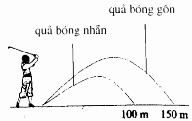
H.48. Trong cùng những điều kiện lăng bóng, quả bóng gôn (móp méo) bay xa hơn một quả bóng nhẵn.
