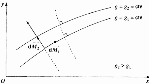
H.23. \overrightarrow{\text{grad}}g vuông góc với các mặt g = \text{cte} và hướng theo chiều các g tăng.
