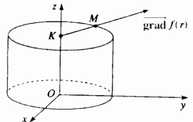
H.31. Tọa độ trụ:
