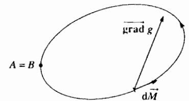
H.26. \oint_C \text{grad } g \cdot d\vec{M} = 0.
