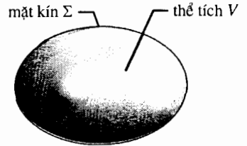
H.13. Mặt kín \Sigma giới hạn một thể tích kết hợp V .
