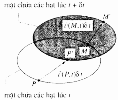
H.2b. Vận động của một mặt chứa hạt : mặt bị chất lỏng "kéo theo". Khối lượng M của chất lỏng, giới hạn bởi mặt chuyển động này, là bất biến với thời gian.
