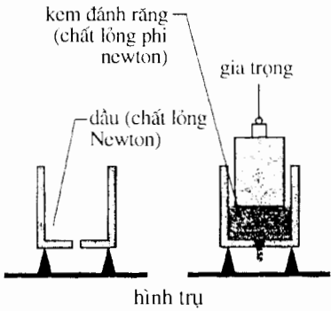
H.60. Trong khi dầu (chất lỏng Newton) chảy dưới tác dụng của chính trọng lượng của nó, thì trong trường hợp kem đánh răng (chất lỏng phi Newton) lại cần phải thêm các gia trọng, dòng chảy mới bắt đầu xảy ra.
