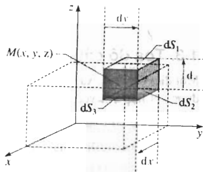
H.3. Thể tích nguyên tố d\tau = dx dy dz được giới hạn bởi sáu diện tích nguyên tố phẳng với dS_1 = dx dy , dS_2 = dy dz và dS_3 = dx dz .
