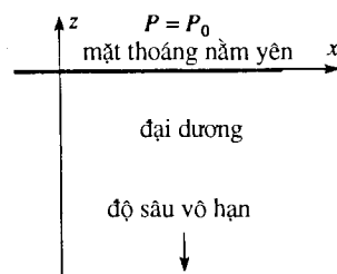
H.45. Đại dương có độ sâu "vô hạn".
