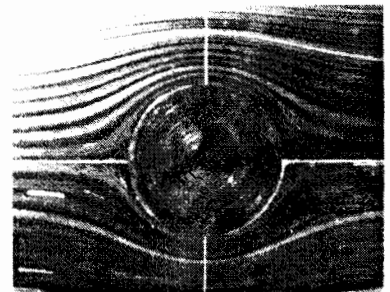
H.47. Dòng chảy xung quanh một hình trụ có bề dày nhỏ (1mm) và vận tốc nhỏ ( 1 \text{ mm.s}^{-1} ). Dòng chảy được thể hiện rõ nhờ các sợi lanh tẩm dầu trong dầu vadolin.
