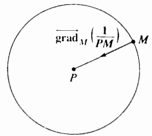
H.30. Khuynh hướng của vector: \overrightarrow{\text{grad}}_M \left( \frac{1}{PM} \right) .
