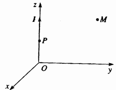
H.57. Cho một dòng điện I chạy trong một dây dẫn trùng với (Oz)
