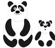
pandas
