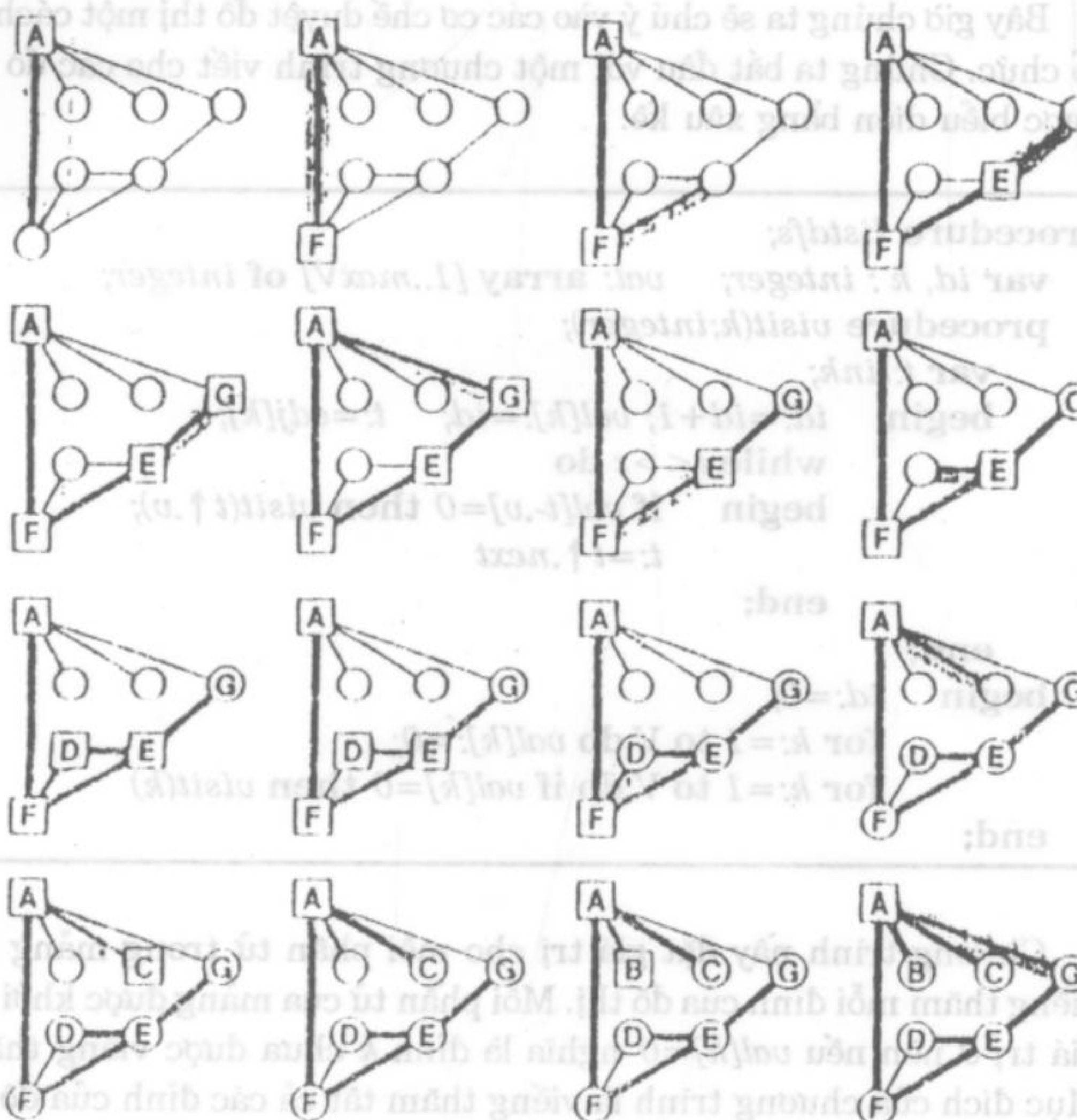
Hình 29.5 Tìm kiếm ưu tiên độ sâu bằng đệ quy
