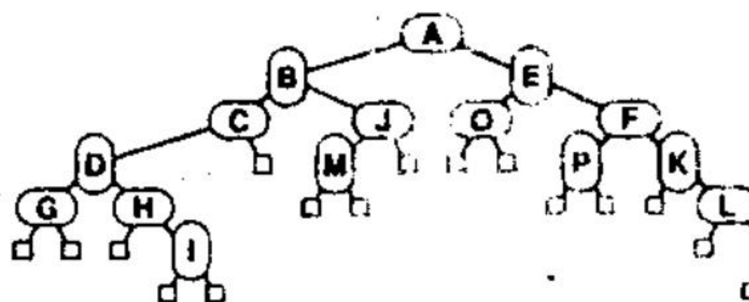
Hình 26.4 Một cây hai chiều (2D)
