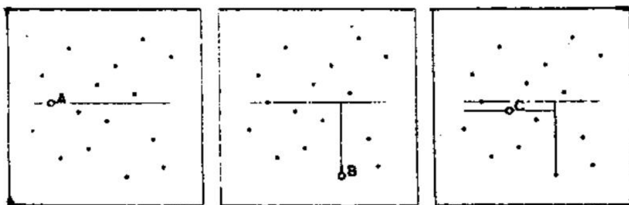
Hình 26.5 Chia nhỏ mặt phẳng bằng một cây 2D (bắt đầu)
