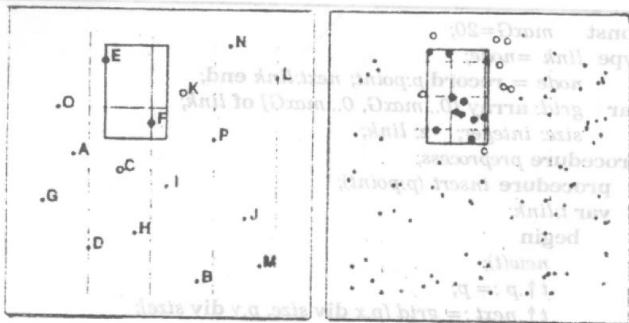
Hình 26.3 Phương pháp Lưới để tìm theo khoảng
