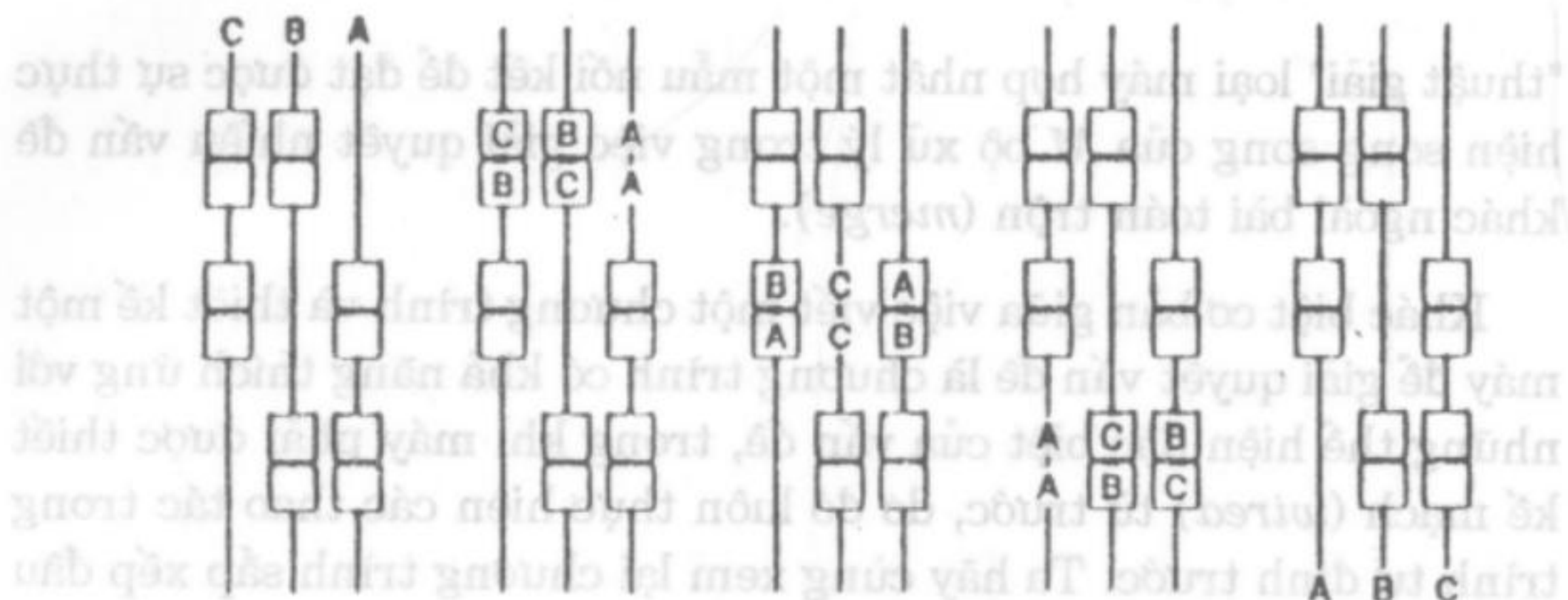
Hình 40.1 Máy sắp xếp ba phần tử
