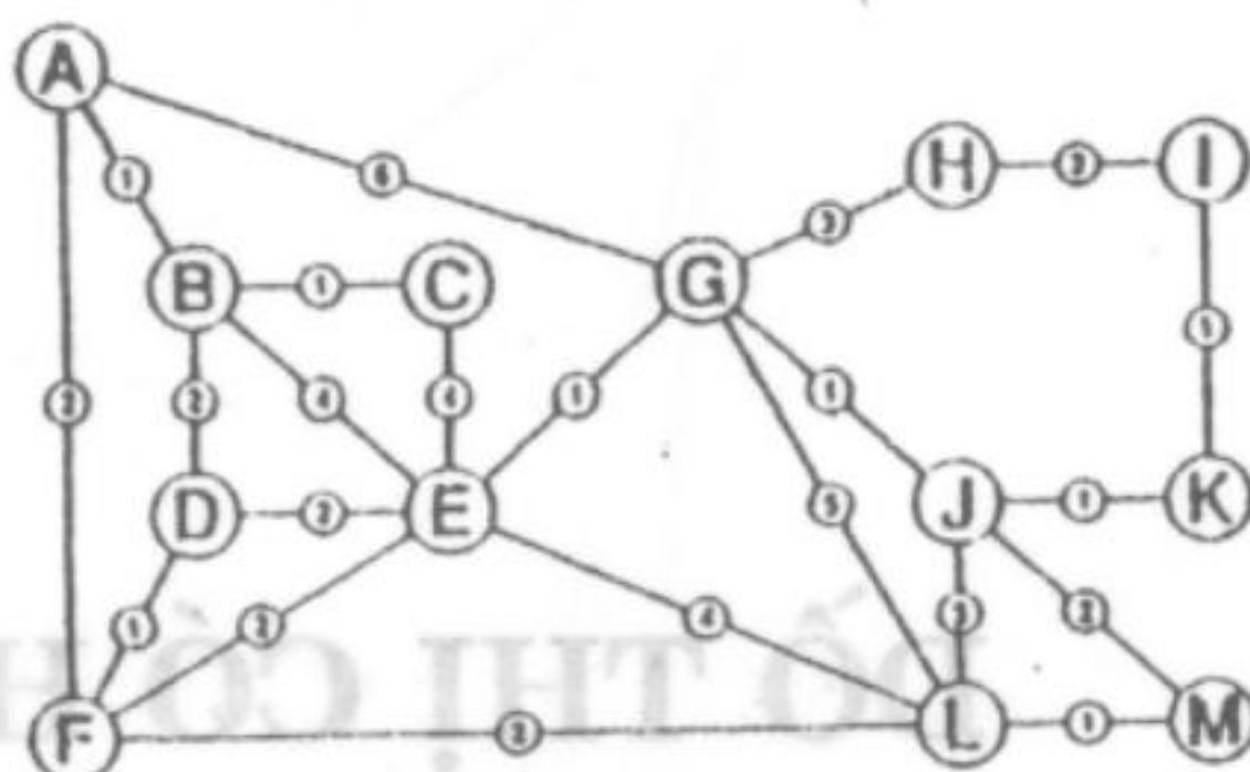
Hình 32.1 Một đồ thị có hướng
