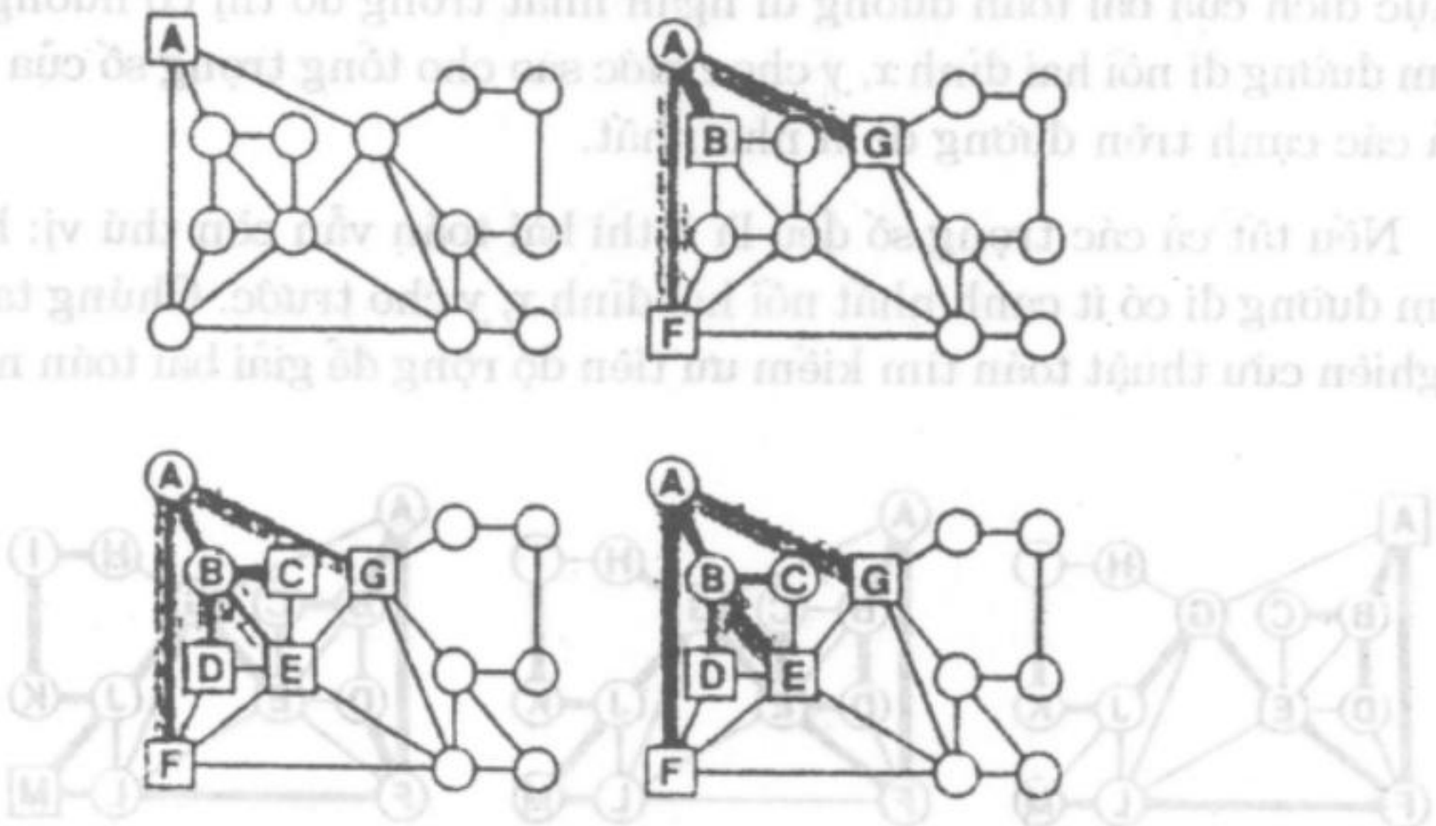
Hình 31.11 Các bước bắt đầu xây dựng một cây bao trùm đường đi ngắn nhất
