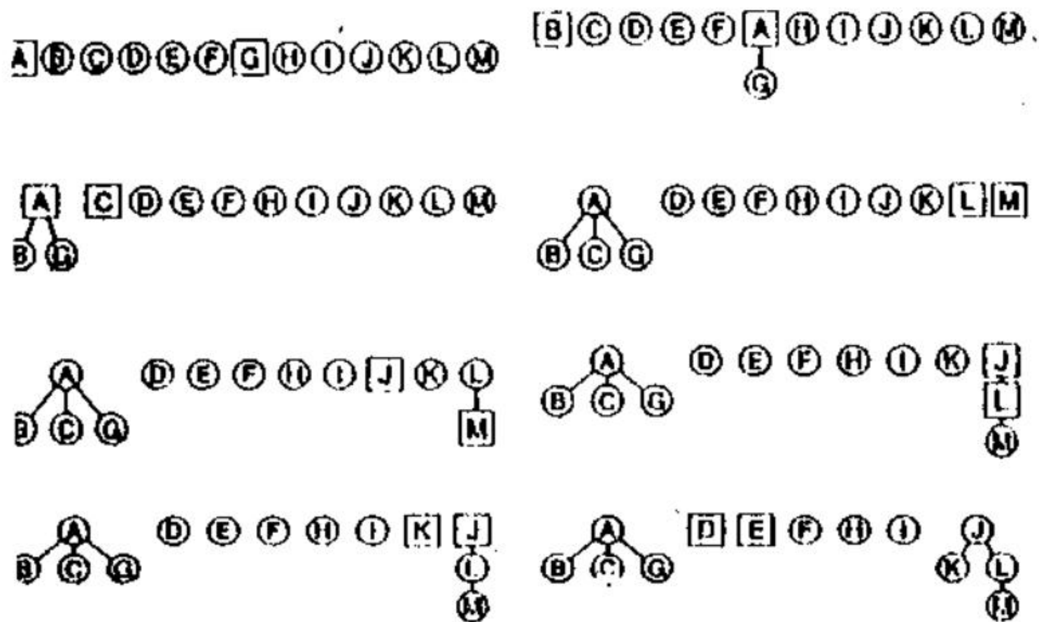
Hình 30.4 Các bước bắt đầu của việc tìm phần hợp
