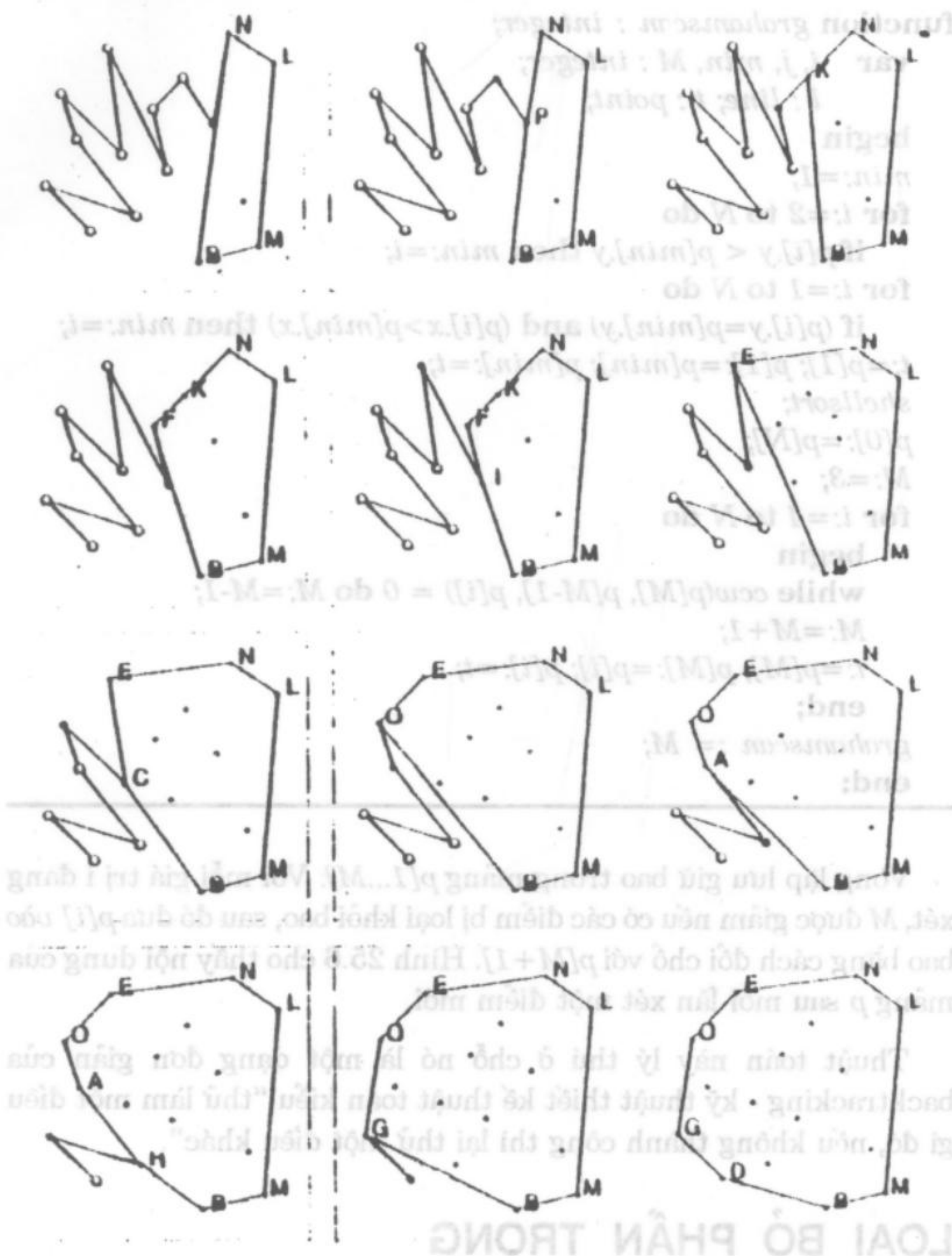
Hình 25.5 Quá trình thực hiện cách xử lý của phép quét Graham
