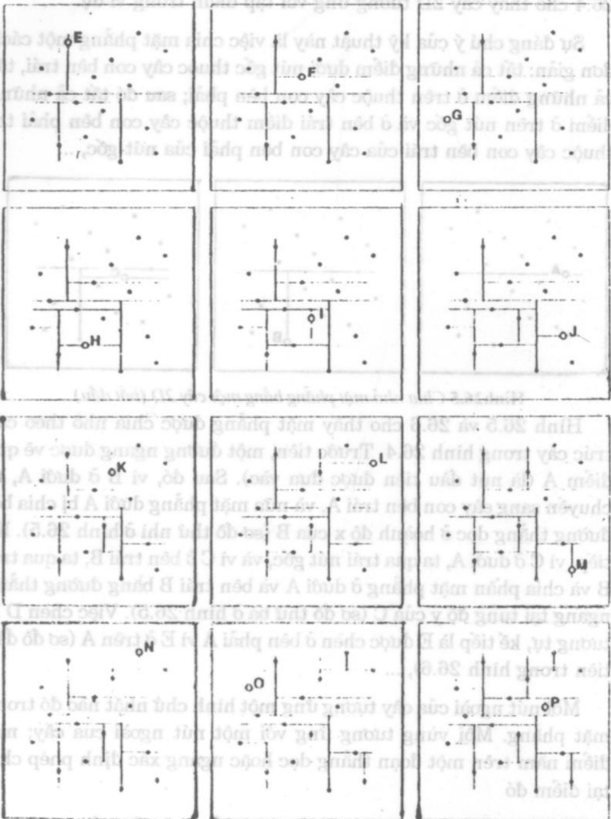
Hình 26.6 Chia nhò mặt phẳng bằng một cây 2D (các bước tiếp theo)
