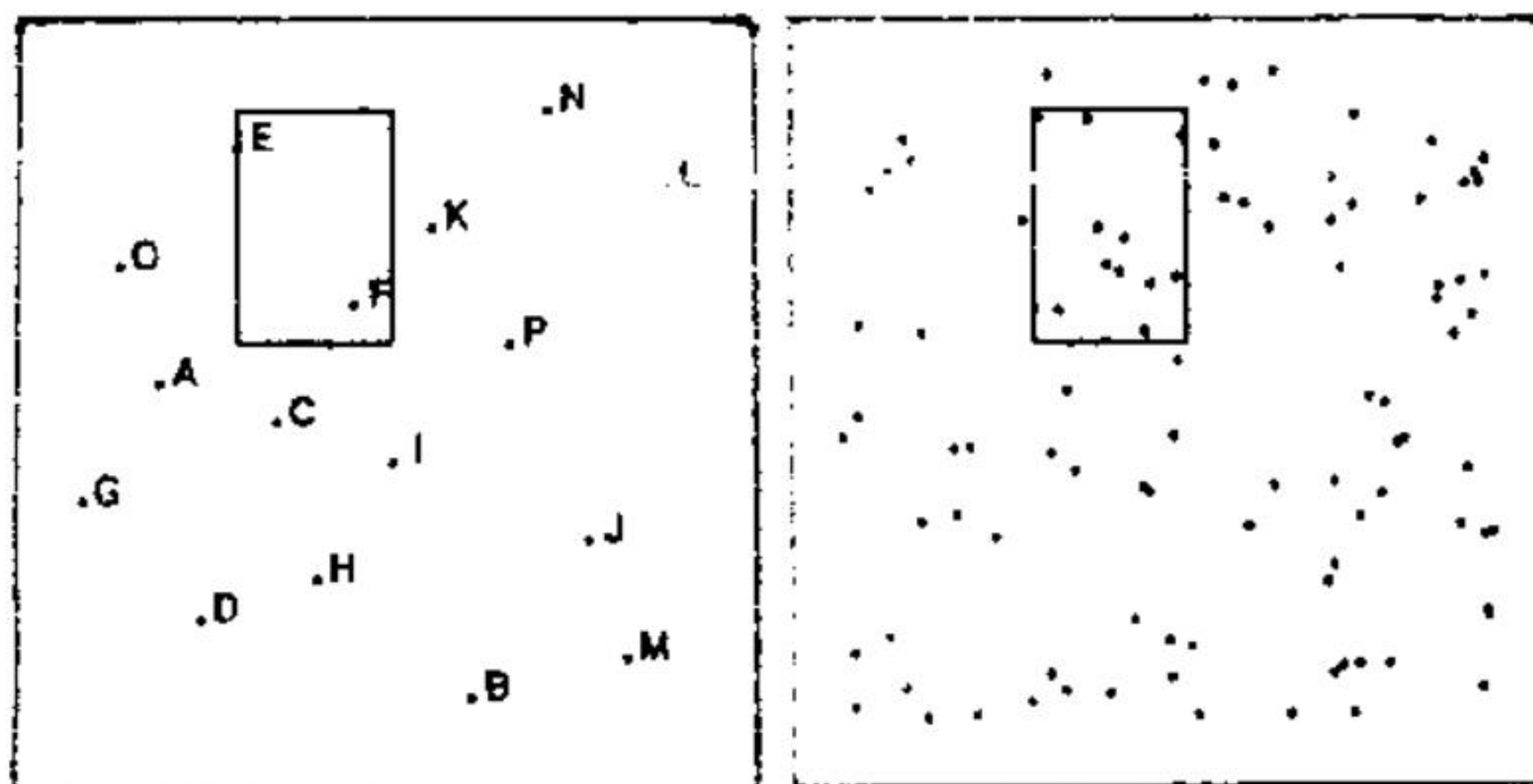
Hình 26.2 Tìm theo khoảng hai chiều
