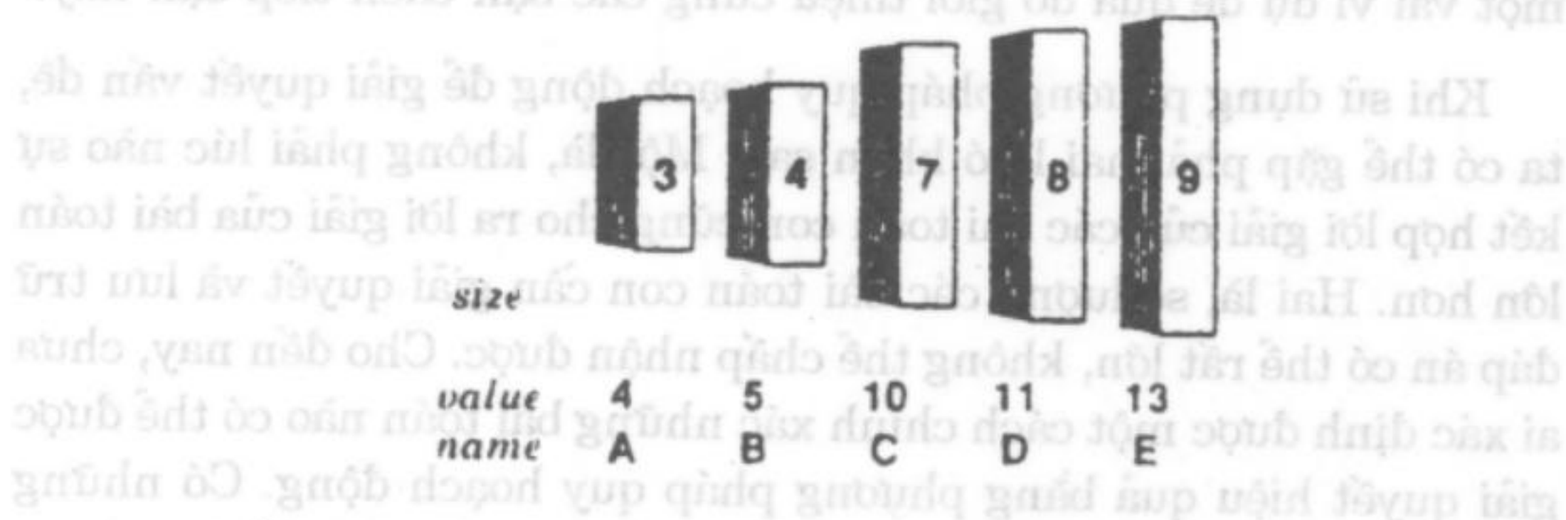
Hình 42.1 Một ví dụ về "bài toán chiếc túi xách"
