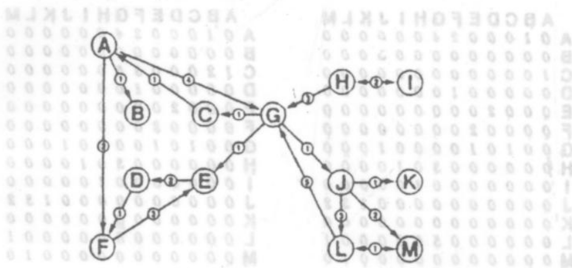
Hình 32.5 Đồ thị có hướng và có trọng
