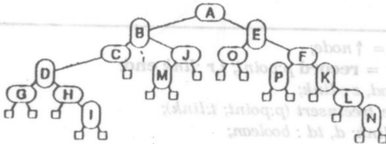
Hình 26.7 Tìm theo khoảng nhờ một cây 2D
