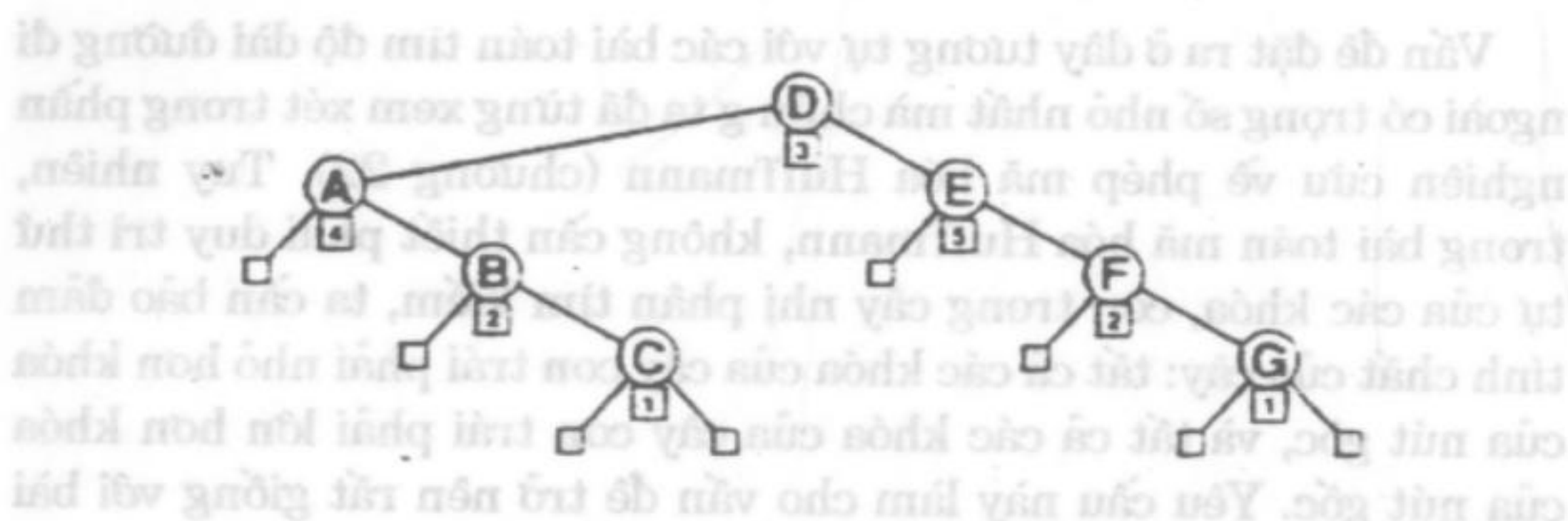
Hình 42.5 Cây nhị phân tìm kiếm tối ưu
