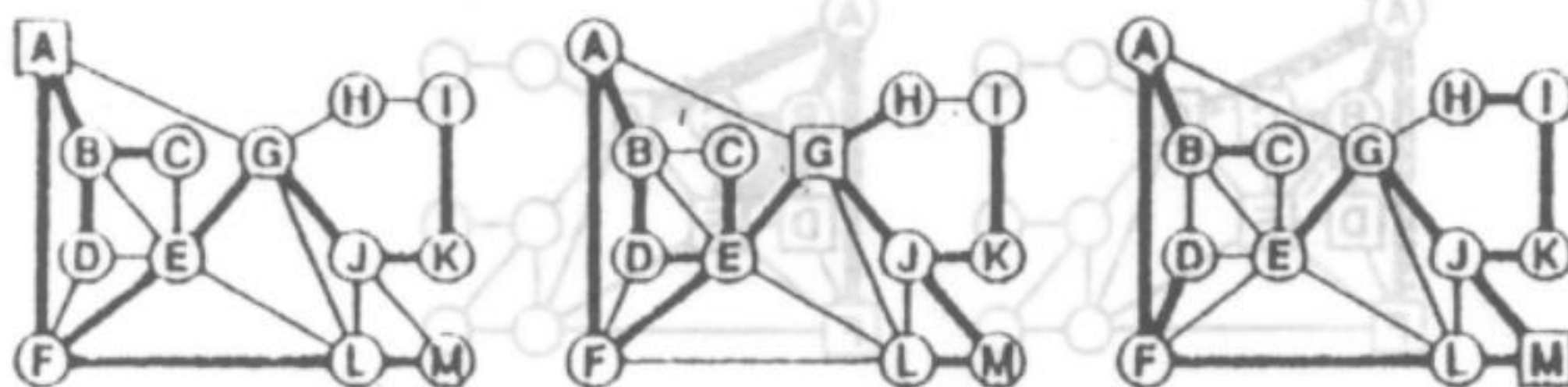
Hình 31.10 Cây bao trùm đường đi ngắn nhất
