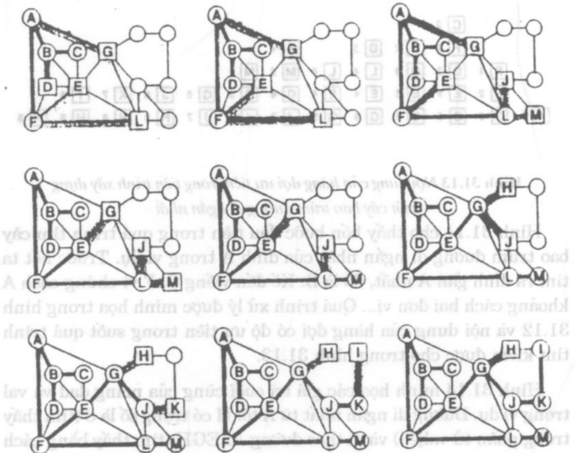
Hình 31.12 Kết quả hoàn tất xây dựng một cây bao trùm đường đi ngắn nhất
