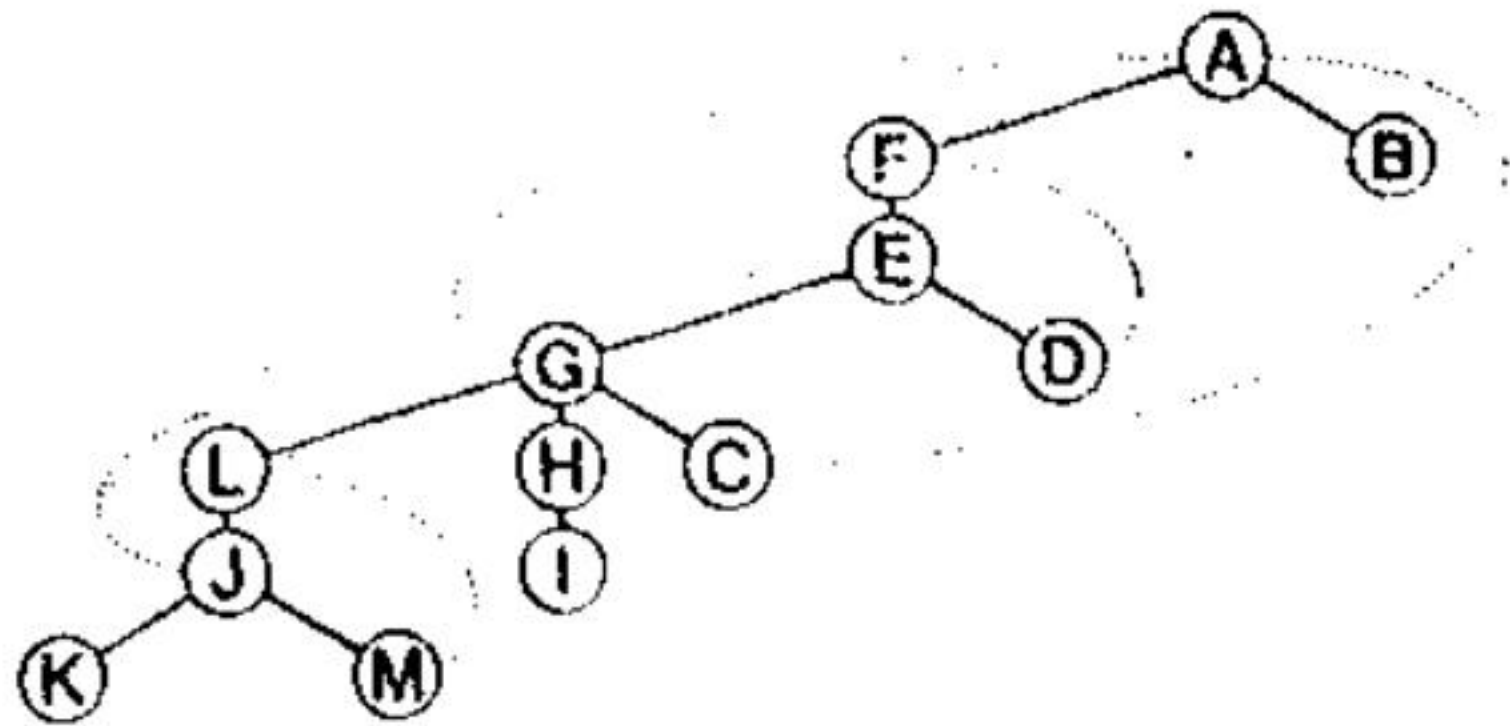
Hình 30.3 DFS để xét song liên thông
