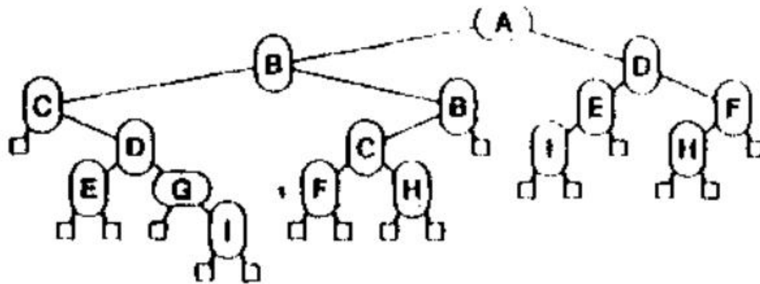
Hình 27.5 Sắp xếp để quét bằng cây y
