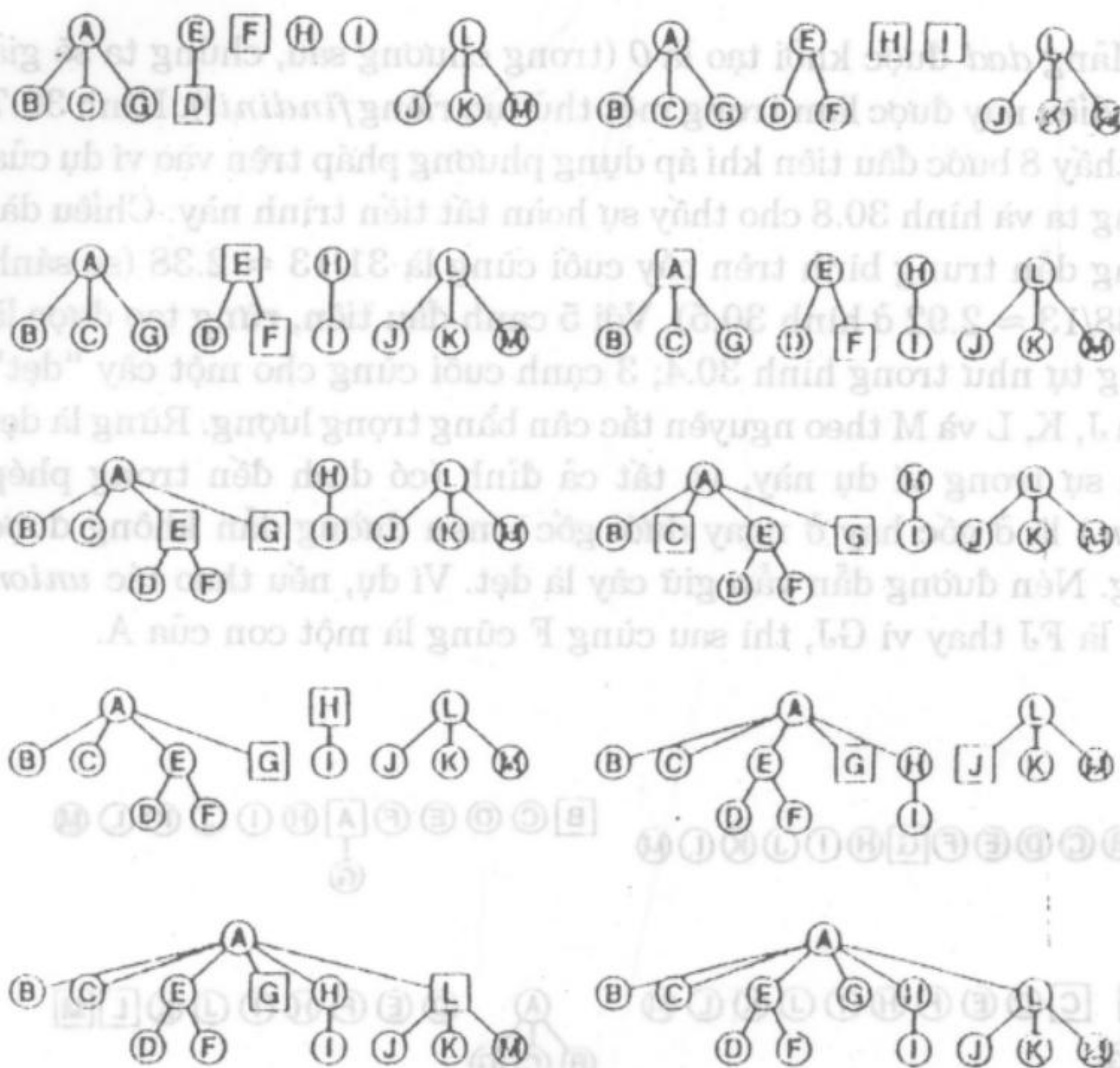
Hình 30.8 Hoàn tất tiến trình tìm phần hợp (trường hợp có trọng số và nén đường dẫn)
