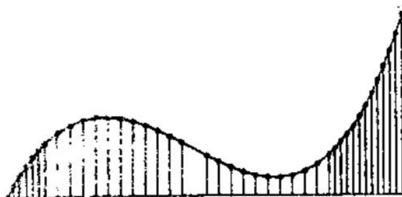
Hình 39.5 Phương pháp cầu phương thích ứng
