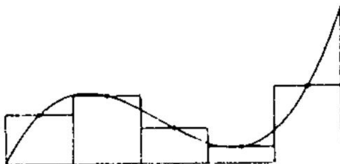
Hình 39.1 Phương pháp hình chữ nhật
