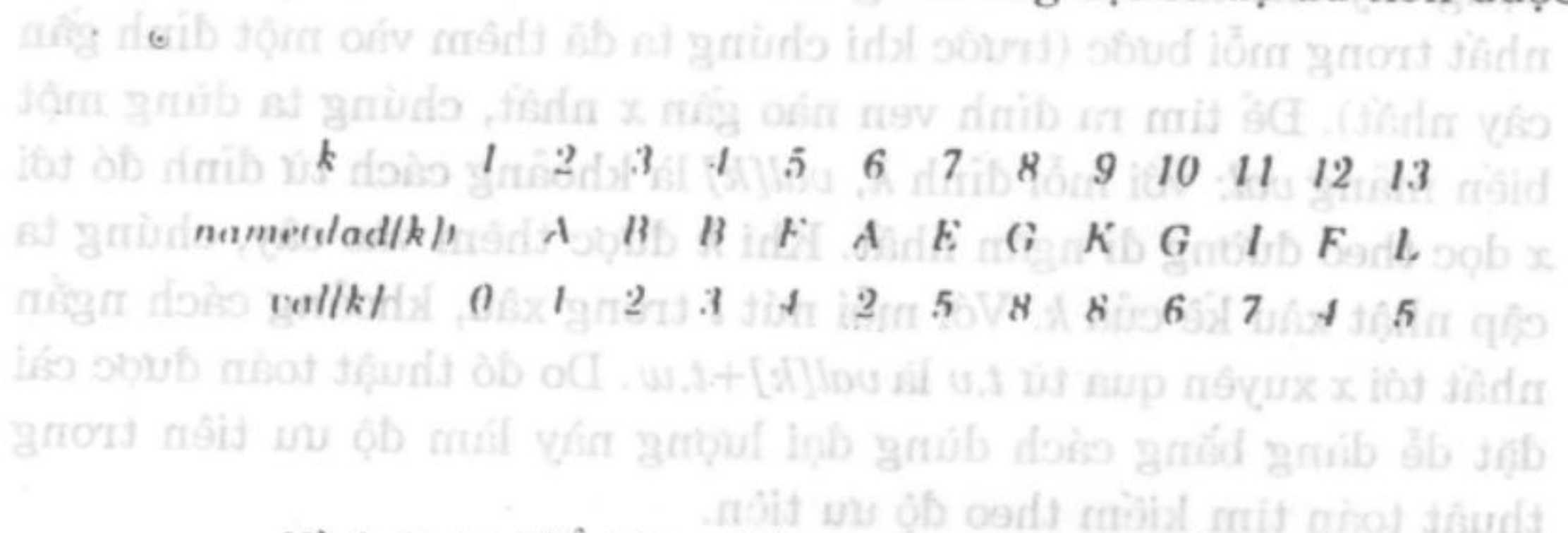
Hình 31.14 Biểu hiện cây bao trùm đường đi ngắn nhất
