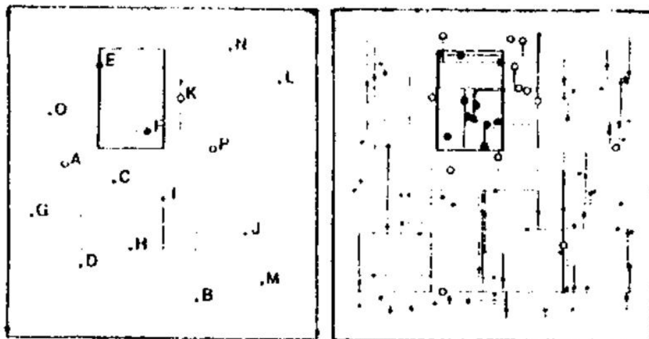
Hình 26.8 Tìm theo khoảng nhờ một cây 2D (chia nhỏ mặt phẳng) các vùng phủ lên hình chữ nhật tìm kiếm. (xem hình 26.7 và 26.8).
