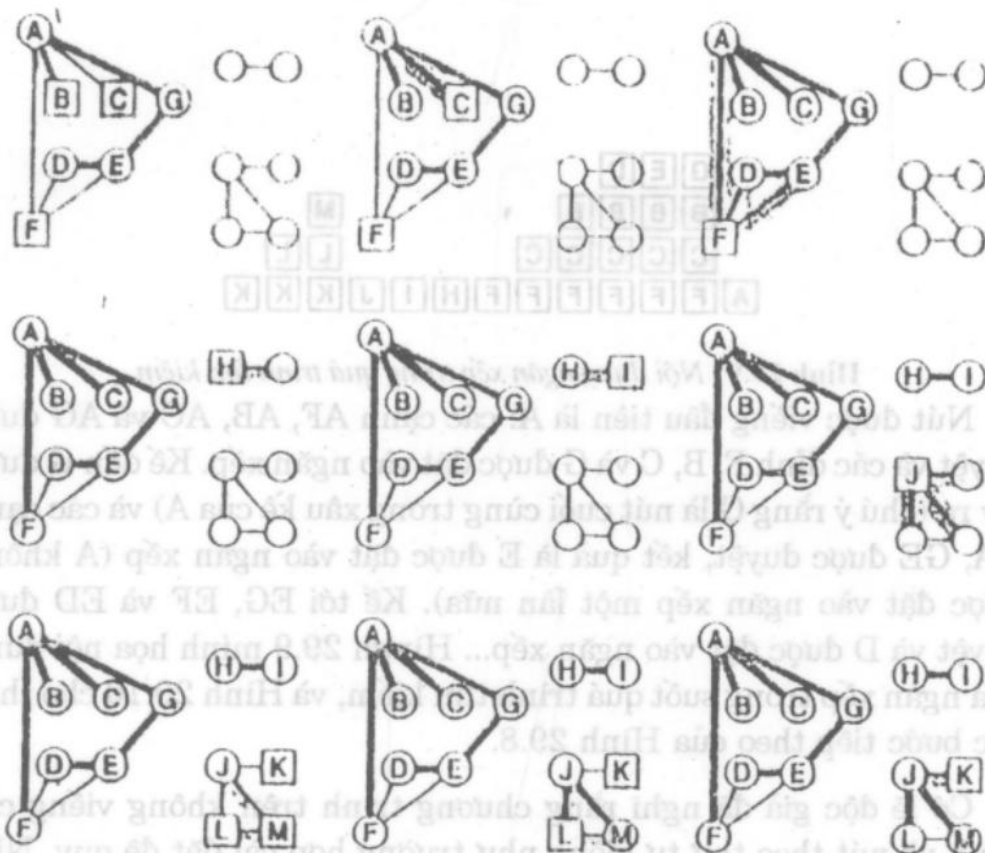
Hình 29.10 Tìm kiếm ưu tiên độ sâu (dựa vào ngăn xếp)
