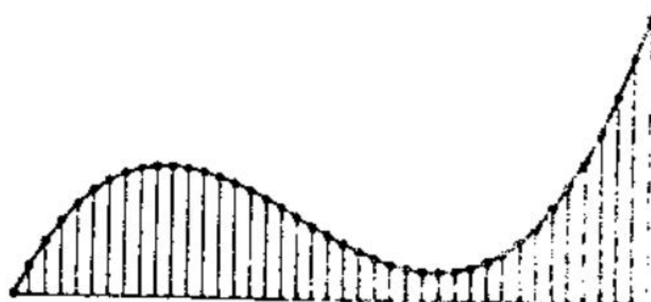
Hình 39.4 Phương pháp hình thang với khoảng chia nhỏ hơn phương pháp hình thang và phương pháp hình chữ nhật, như ta sẽ thấy dưới đây.
