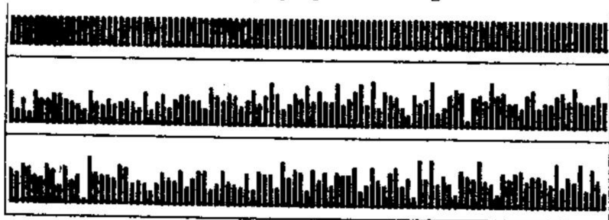
Hình 35.2 Tần số xuất hiện của mỗi giá trị 100 trong ba bảng của phương pháp đồng dư tuyến tính
