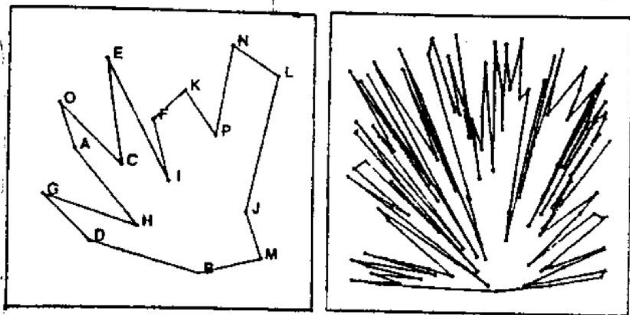
Hình 24.4 Đường khép kín đơn
