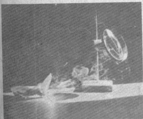
Dùng thấu kính đốt giấy
