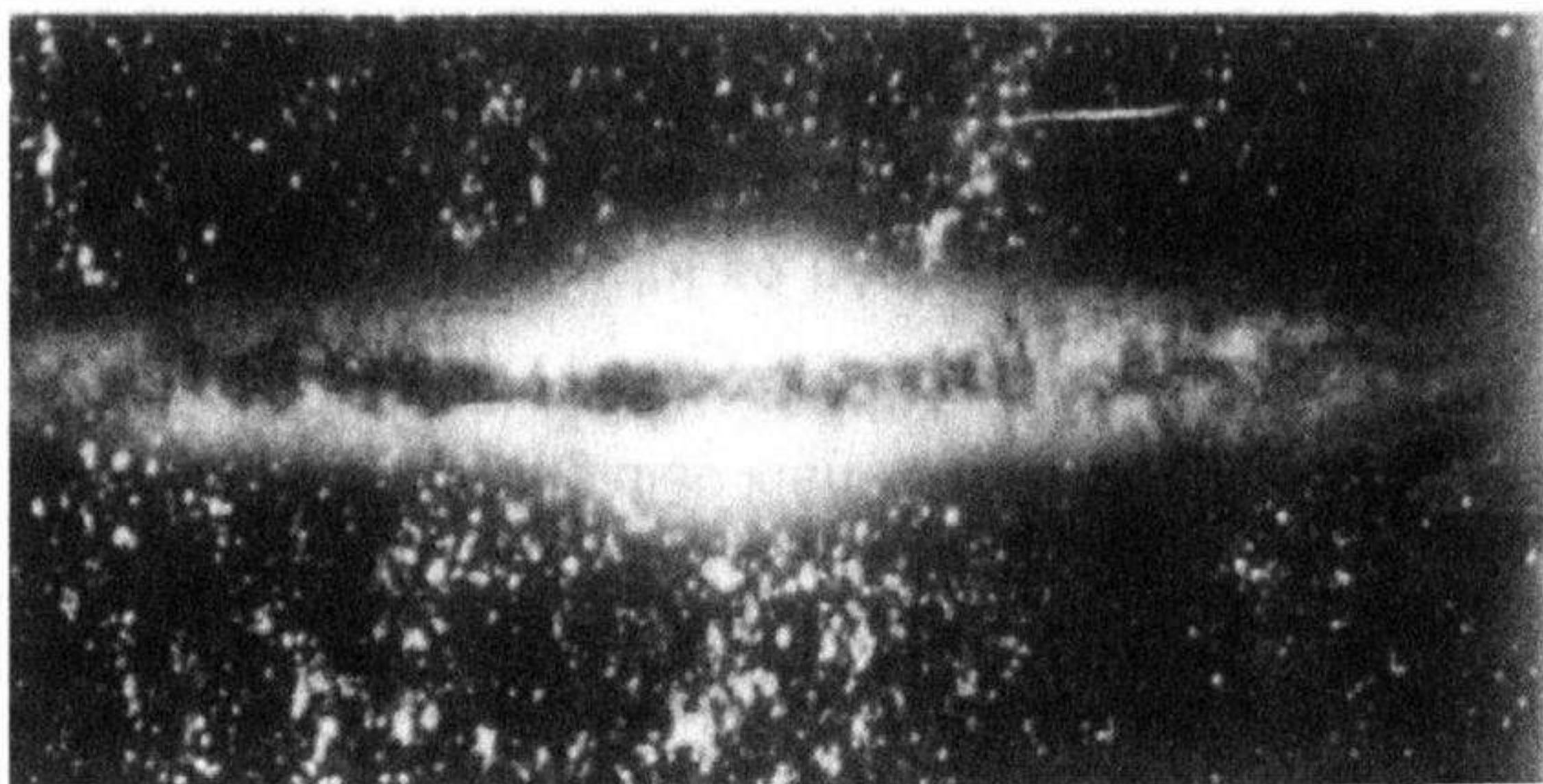
Toàn cảnh dải Ngân Hà. Thái Dương hệ của chúng ta chỉ là một phần nhỏ bé trong đó.
