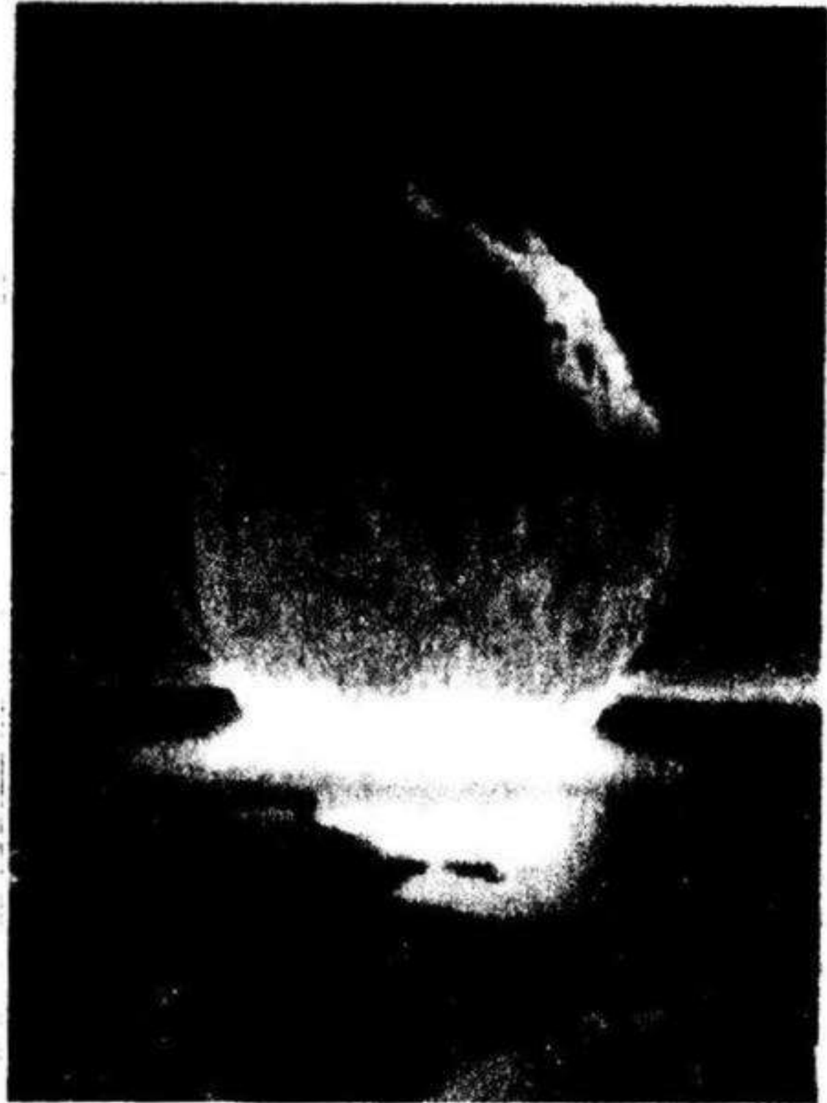
Quang cảnh ở Tunguska trong vụ nổ được vẽ lại bằng vi tính
