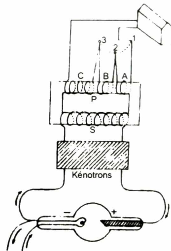
Hình 1.20. Sơ đồ máy Xquang có bộ phận chỉnh lưu
