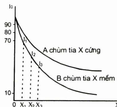
Hình 1.3. Đồ thị giảm cường độ tia X theo chiều dày vật hấp thụ
