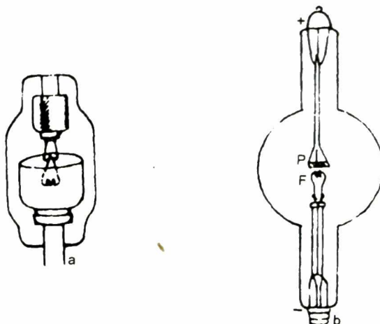
Hình 1.16. Kenotron a) Loại đặt trong dầu, b) Loại đặt giữa không khí
