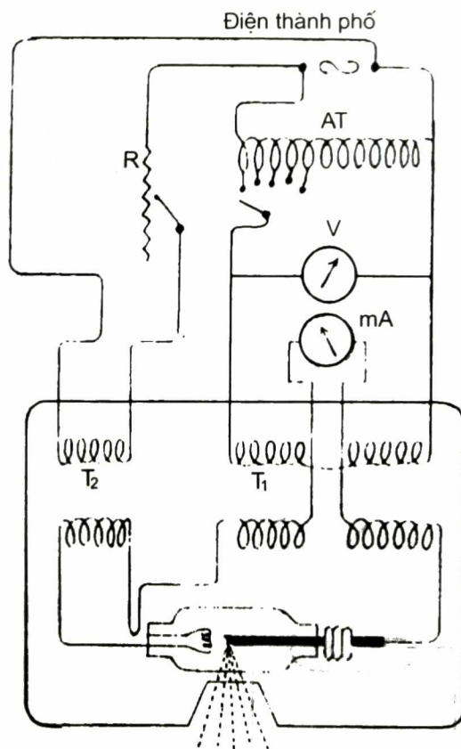
Hình 1.17. Sơ đồ máy X quang nửa sóng
