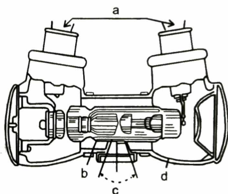
Hình 1.12: Bóng trong vỏ chì chứa dầu
