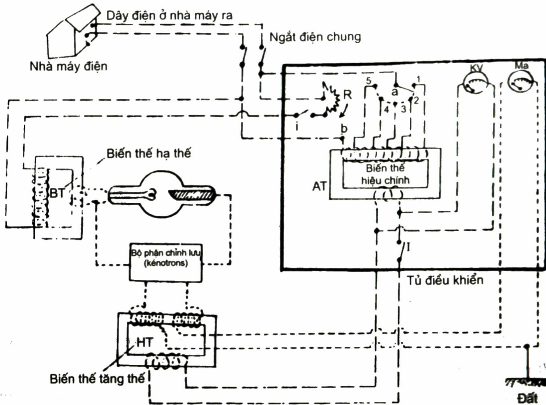
Hình 1.21. Máy 4 kenotron với các bộ phận điều khiển và giám sát
