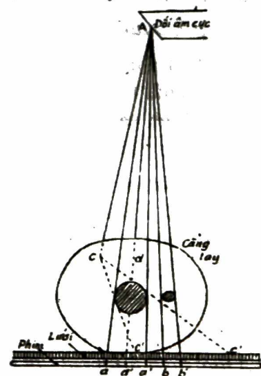
Hình 1.29. Sơ đồ nguyên lý lưới chống mờ di động (Porter Bucky)
