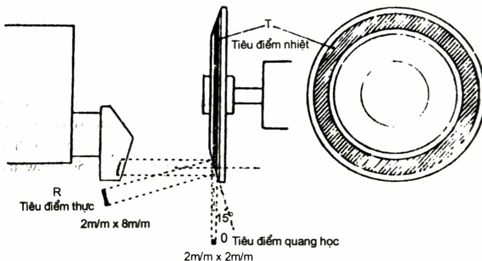
Hình1.15: Sơ đồ bóng đôi âm cực quay
