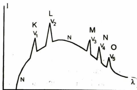
Hình 1.2. Quang phổ vạch
