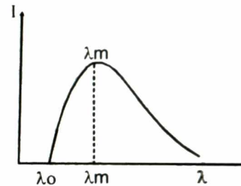
Hình 1.1. Quang phổ liên tục
