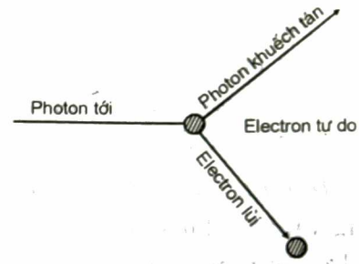
Hình 1.5. Hiệu ứng Compton
