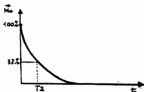
Hình 1.55. Thời gian thư giãn T2
