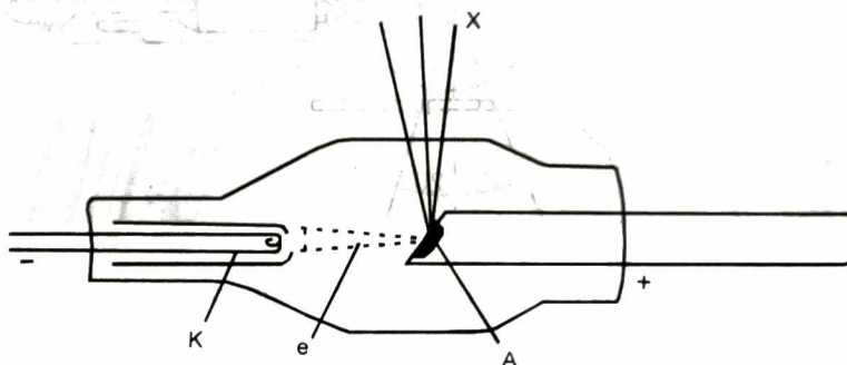
Hình 1.10. Sơ đồ nguyên lý bóng Coolidge
