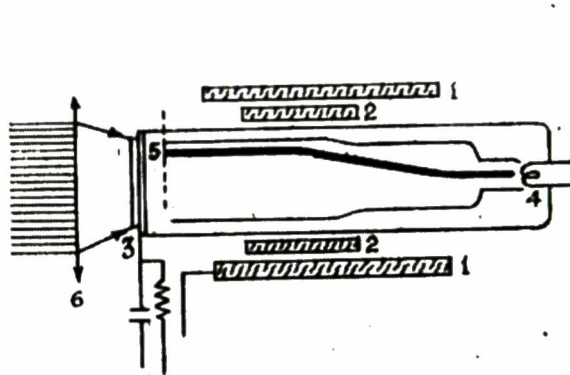
Hình 1.35 Bóng Vidicon
