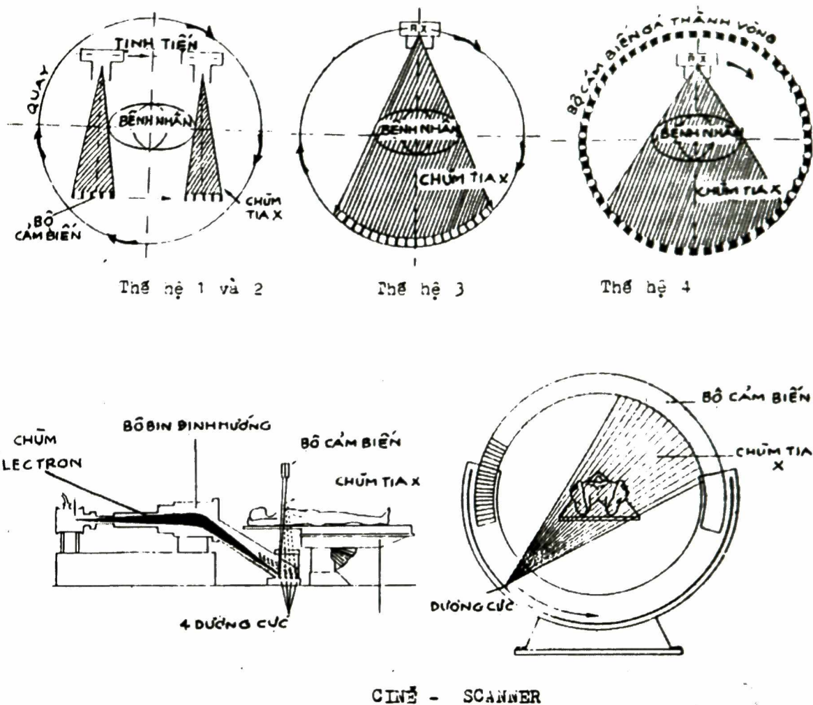
Hình 1.44. Các thế hệ máy chụp cắt lớp vi tính
