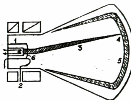
Hình 1.36. Bóng truyền hình
