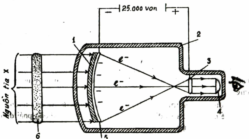
Hình 1.32. Sơ đồ bóng tăng sáng
