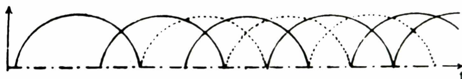
Hình 1.23B. Những giao lưu trực tiếp (đường đậm) và những giao lưu đảo ngược (đường chấm) của dòng điện ba pha sau khi đã qua máy phát điện trên.
