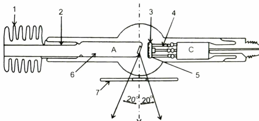
Hình 1.11. Bóng Coolidge có ổ nguội
