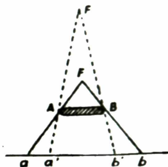
Hình 1.25. bóng X quang càng xa thì hình của vật càng ít bị lớn lên
