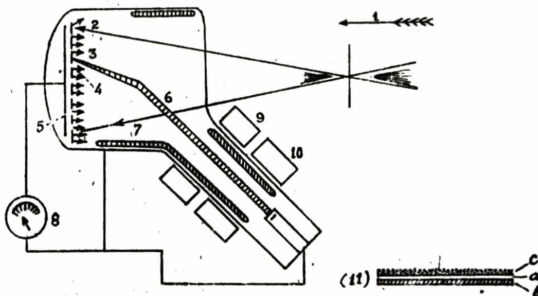
Hình 1.34. Máy Inocop: một loại máy cũ để dễ hiểu sơ đồ nguyên lý
