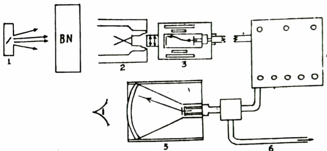
Hình 1.33. Sơ đồ một dây chuyền truyền hình kết hợp với một bóng tăng sáng
