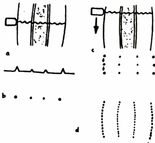
Hình 1.60. Nguyên lý siêu âm vang đổ kiểu B
