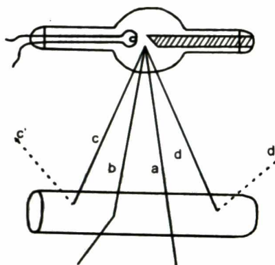
Hình 1.4. Cơ chế sự hấp thụ: các loại tia x thứ cấp
