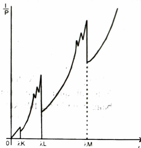
Hình 1.7. Gián đoạn hấp thụ
