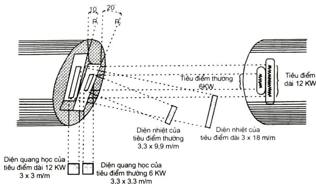
Hình 1.13 Nguyên lý của bóng có hai tiêu điểm, độ nghiêng khác nhau
