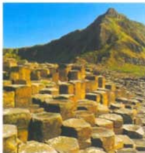
Cảnh đồng đá Giant Causeway được tạo thành từ hàng ngàn cột đá basalt.
