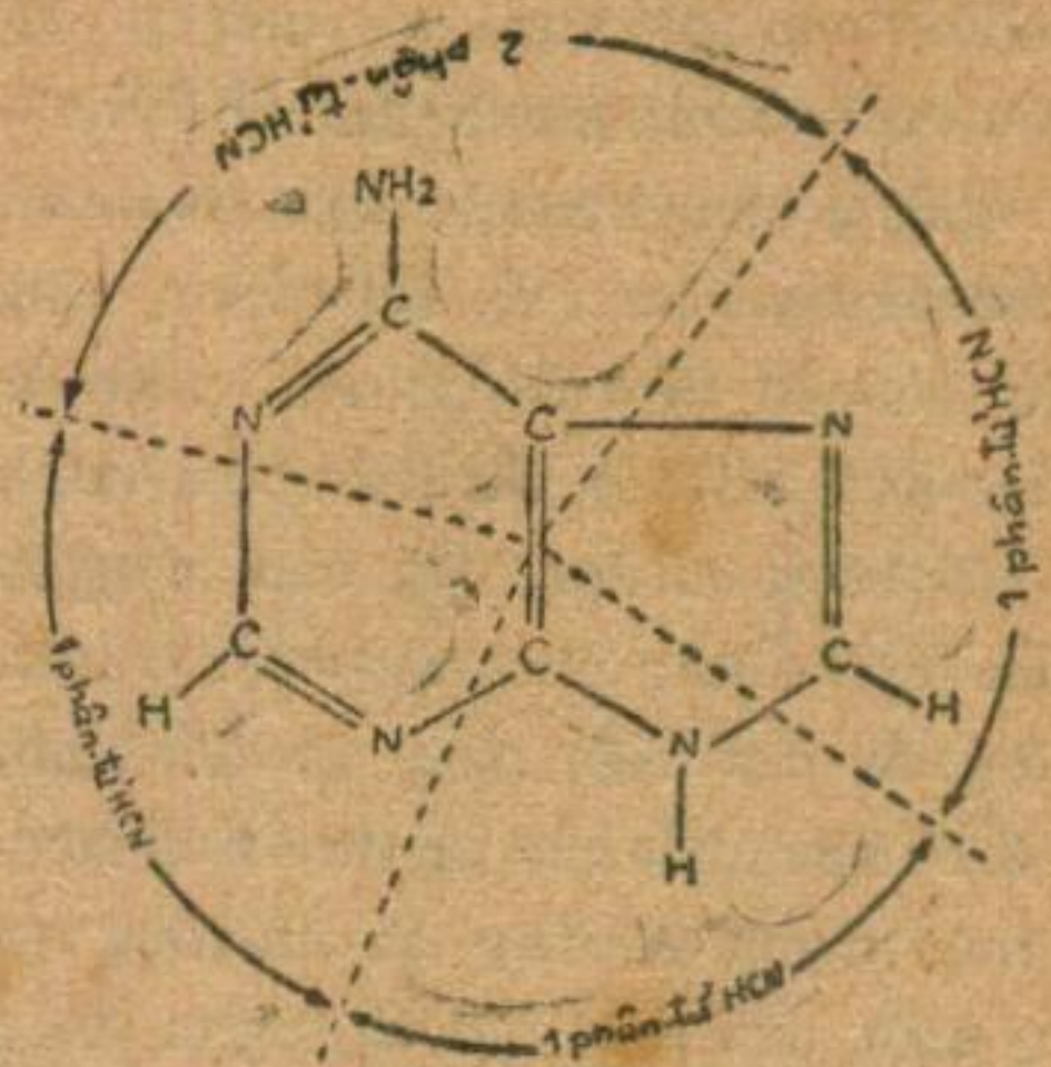
Một phân-tử adénine bằng năm phân- tử acid cyanhydríc (HCN).
