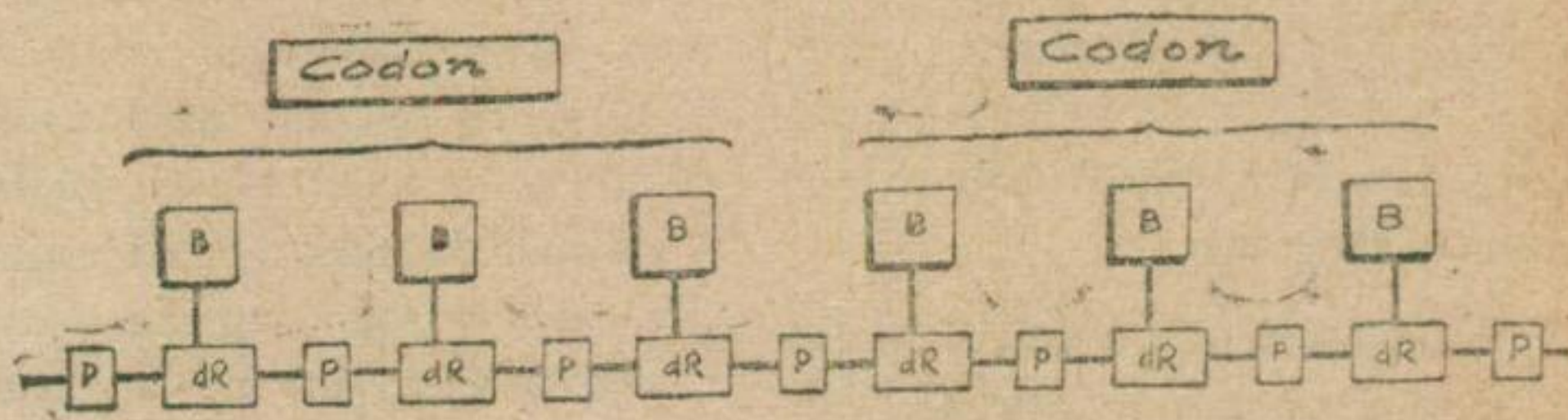
Cấu-trúc theo đường thẳng của ADN và ý-niệm Codon (1)
